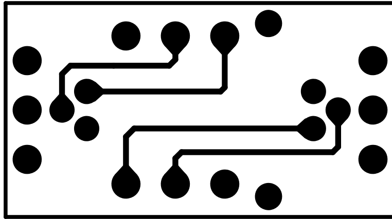
BOT (半田面パターン)
