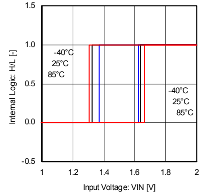
Fig.3 入カスレッシュホールド電圧
