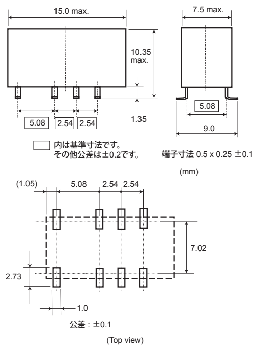
高接続信頼性型／ノンラッチング型 高接続信頼性型／1巻線ラッチング型
