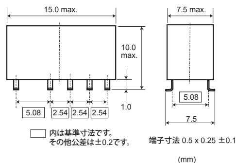
高密度実装型／2巻線ラッチング型
