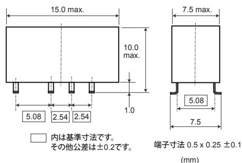
高密度実装型／ノンラッチング型 高密度実装型／1巻線ラッチング型
