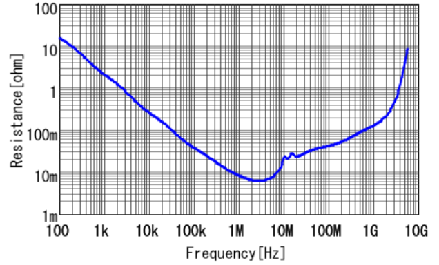
周波数特性R
