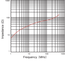
GTR-16-10-10
