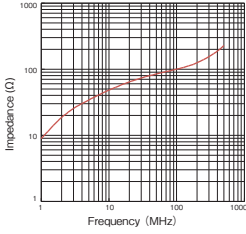
GTR-28-16-20
