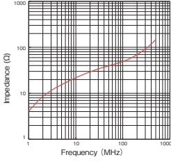
GTR-22-14-10
