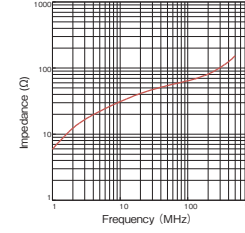
GTR-25-15-12
