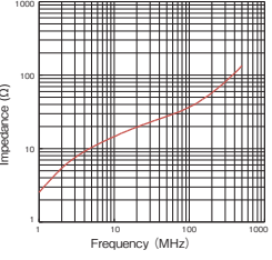
GTR-28-16-13
