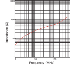
GTR-16-8-16
