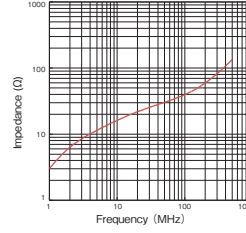
GTR-25-15-8
