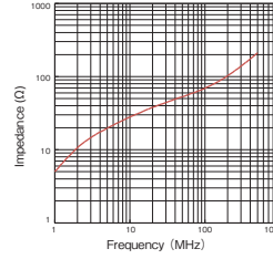
GTR-40-27-15
