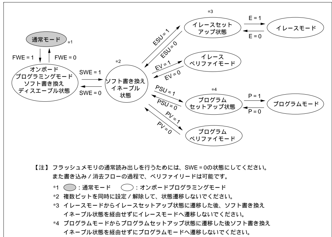
図 18.9 FLMCR1 の各ビット設定による状態遷移
