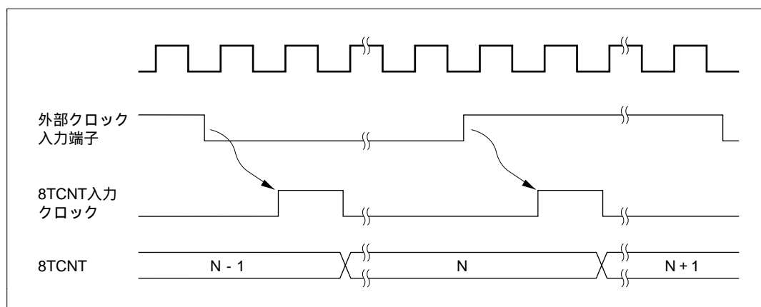
図 10.9 外部クロック動作時のカウントタイミング (両エッジ検出の場合)
