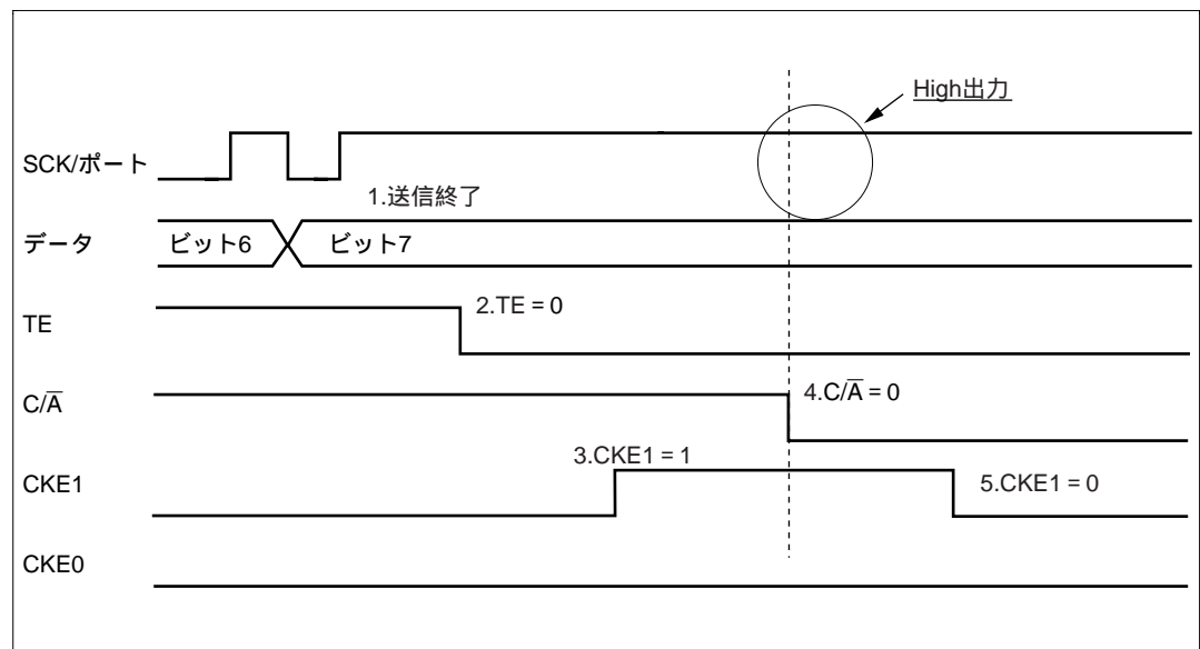
図 13.24 SCK 端子からポート端子へ切り換えるときの動作 (Low 出力の回避例)
