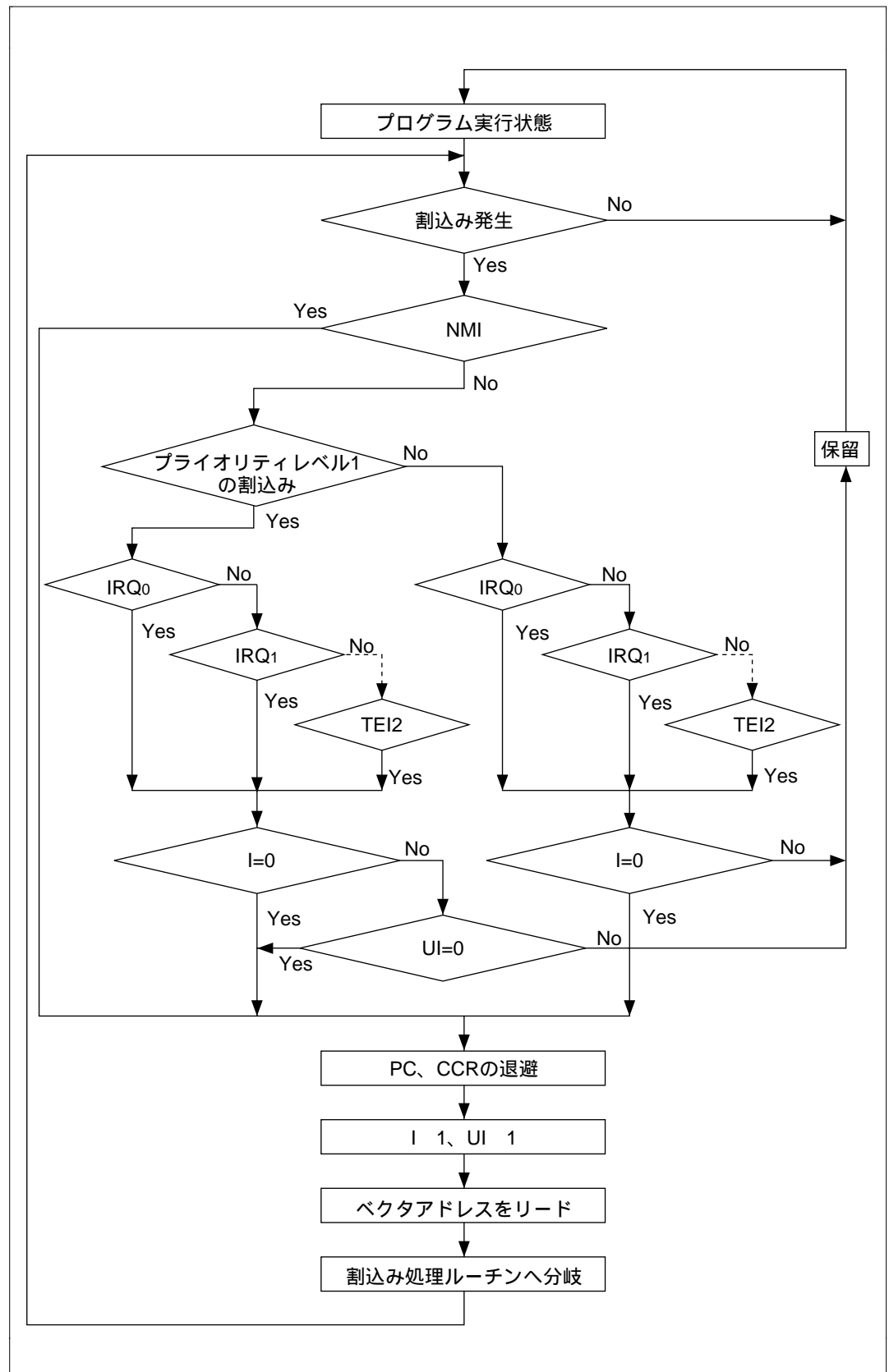
図 5.6 UE = 0 の場合の割り込み受けまでのフロー
