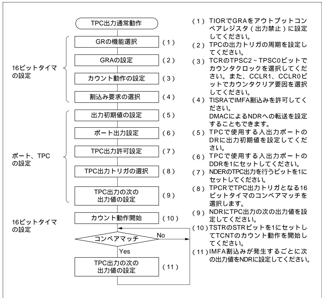
図 11.4 TPC 出力通常動作の設定手順例
