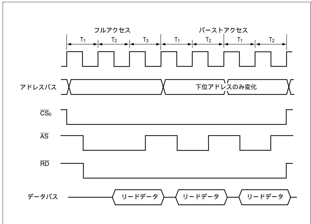
図 6.42 バースト ROM アクセスタイミング例
