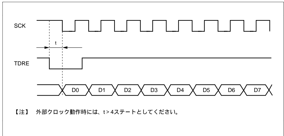
図 13.22 DMAC によるクロック同期式送信時の例
