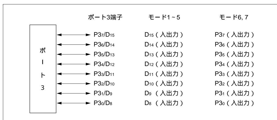
図 8.3 ポート3の端子構成
