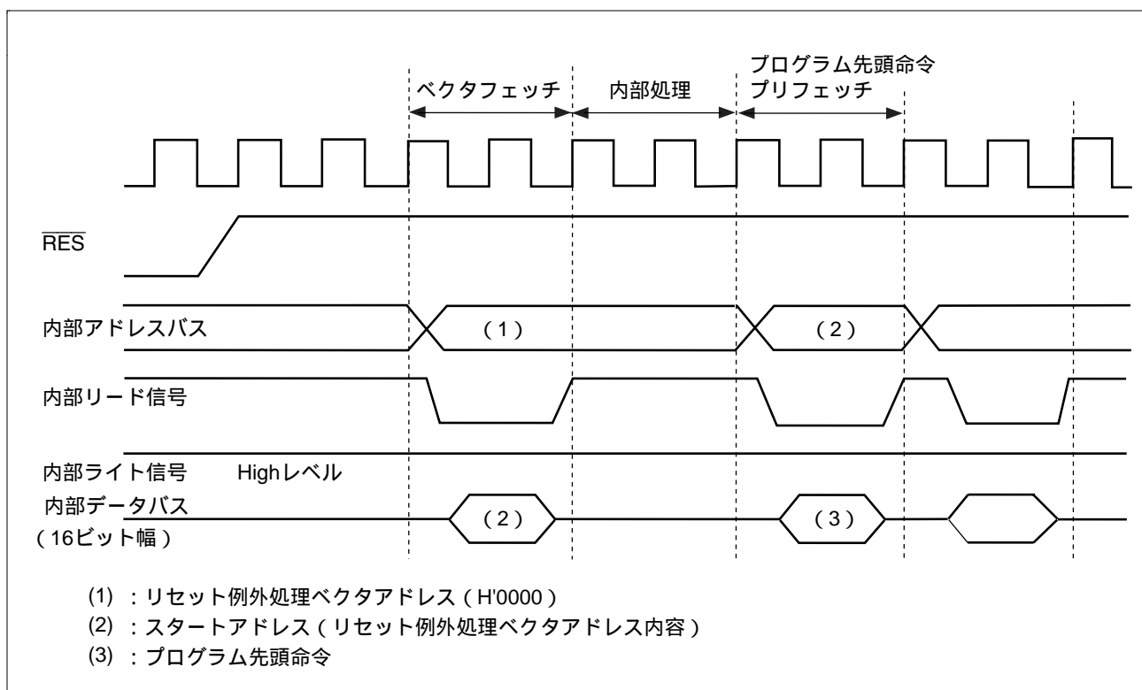
図 4.4 リセットシーケンス (モード6)
