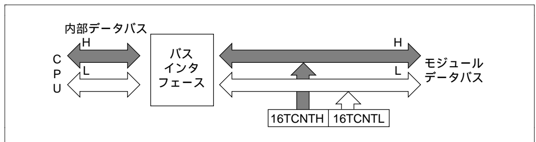
図 9.8 16TCNTHのアクセス動作 [16TCNTH CPU (上位バイト)]
