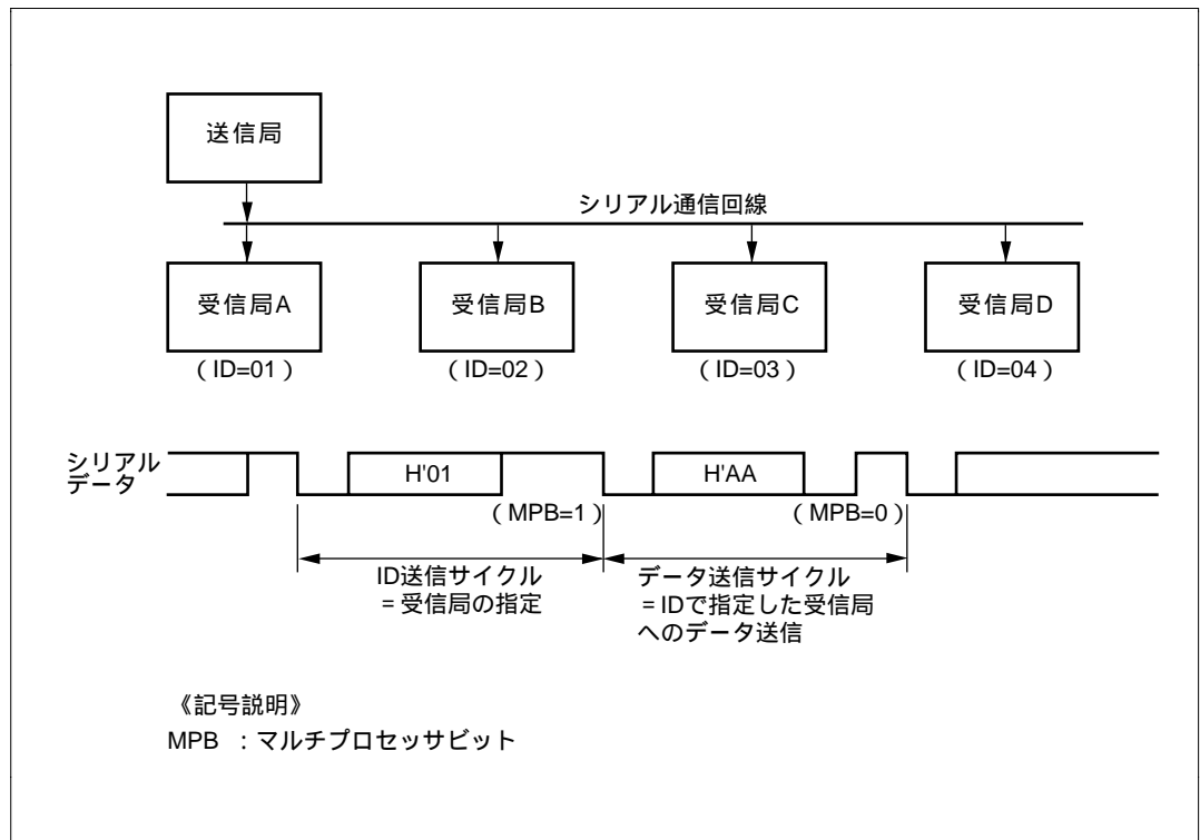
図 13.9 マルチプロセッサフォーマットを使用したプロセッサ間通信の例 (受信局 A へのデータ H'AA の送信の例)
