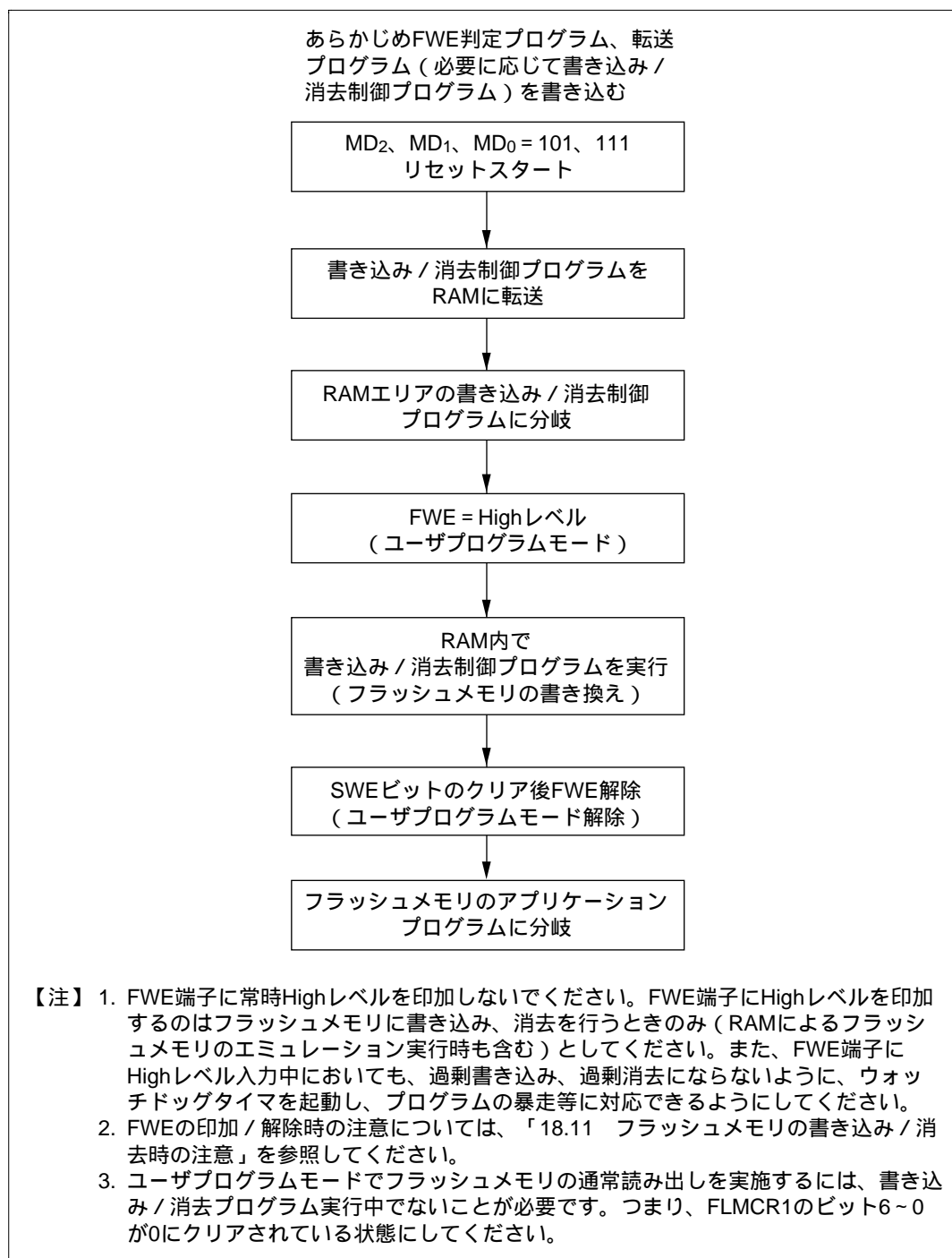
図 18.8 ユーザプログラムモードの実行手順例
