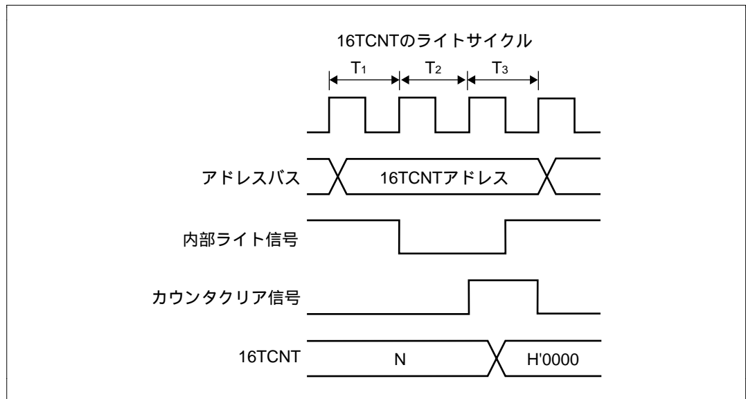
図 9.37 16TCNT のライトとクリアの競合
