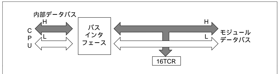
図 9.10 16TCR のアクセス動作 [ CPU 16TCR ]
