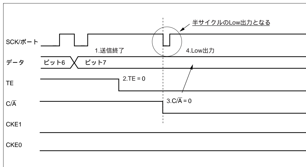
図 13.23 SCK 端子からポート端子へ切り換えるときの動作
