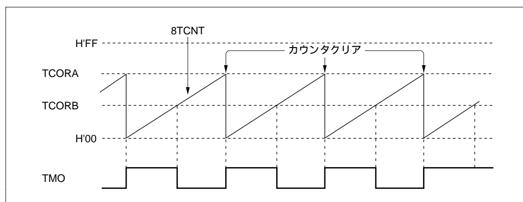
図 10.17 パルス出力例
