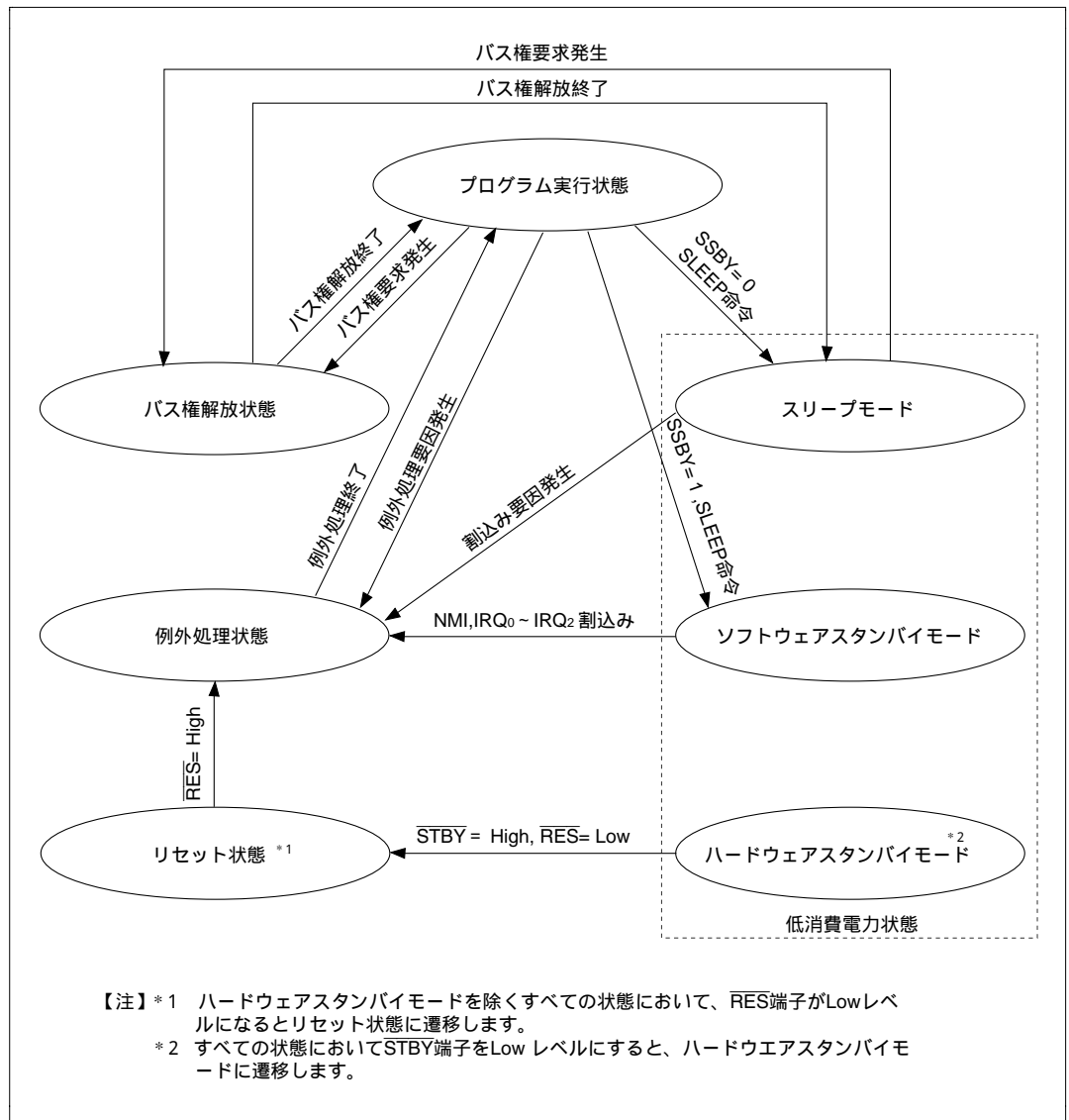
図 2.13 状態遷移図
