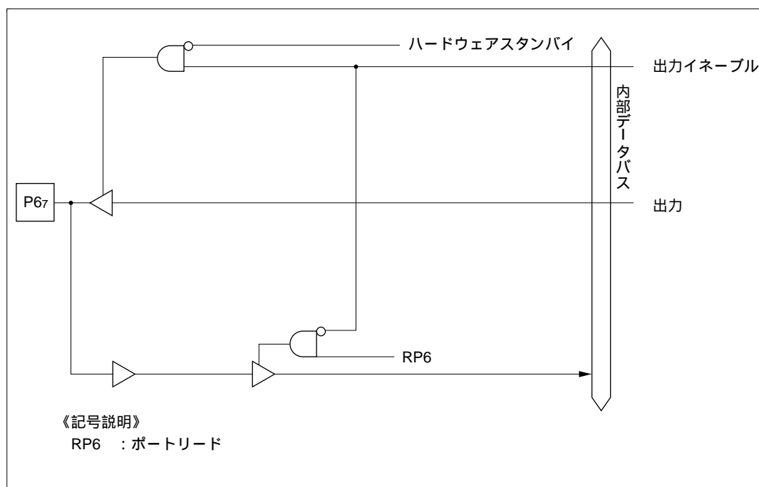
図 C.6 (g) ポート 6 ブロック図 (P6 7 端子)
