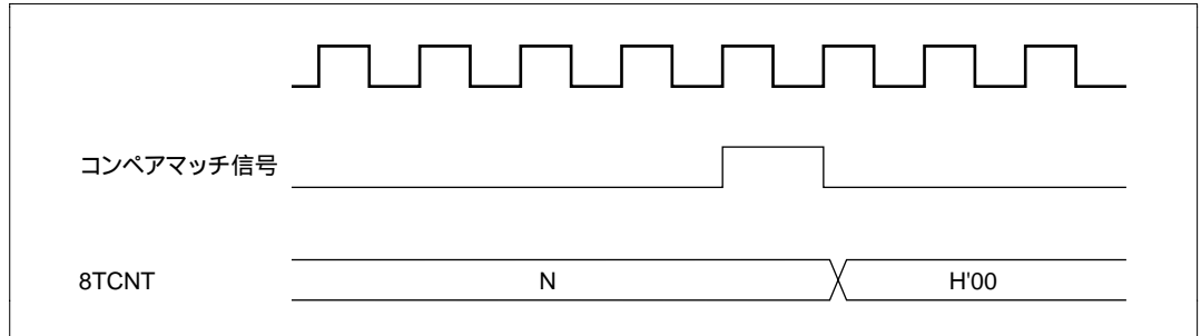
図 10.11 コンペアマッチによるクリアタイミング
