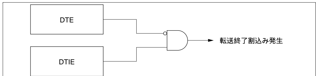
図 7.25 転送終了割り込みブロック図
