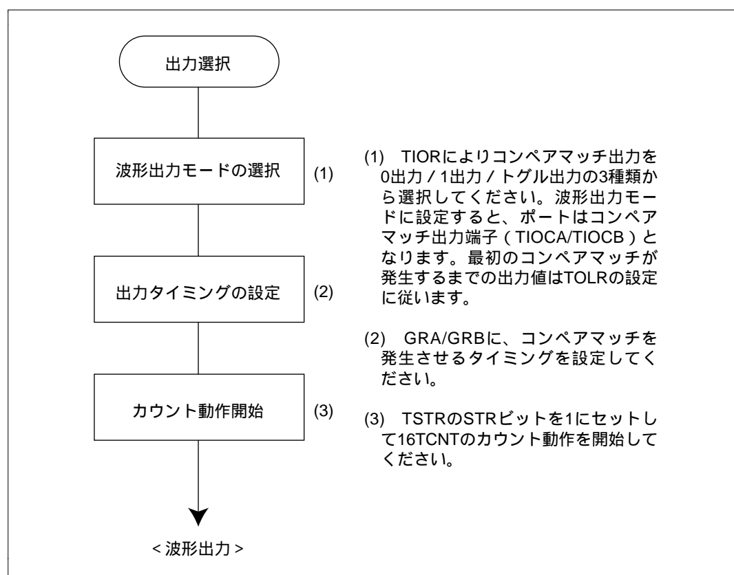
図9.17 コンペアマッチによる波形出力動作例
