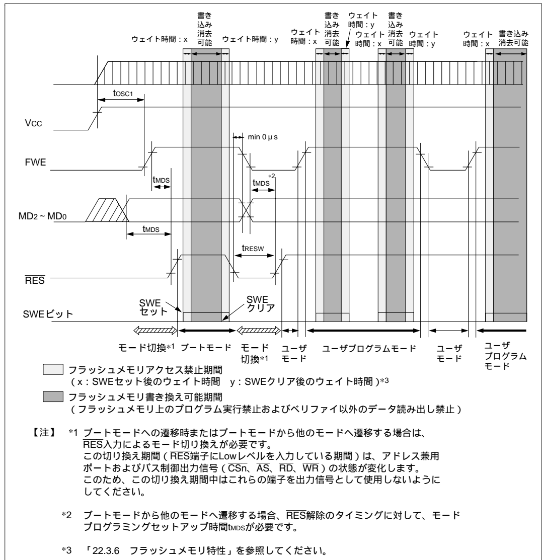
図 18.18 モード遷移タイミング
