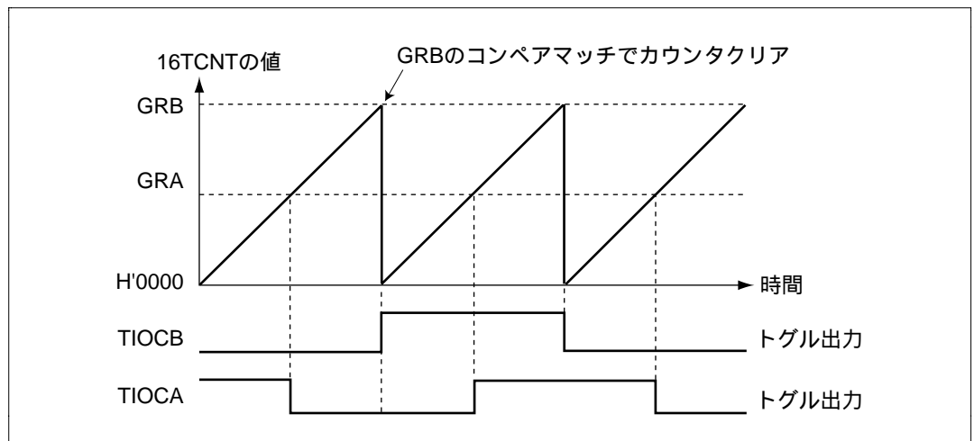
図 9.19 トグル出力の動作例 (TOA=1、TOB=0の場合)
