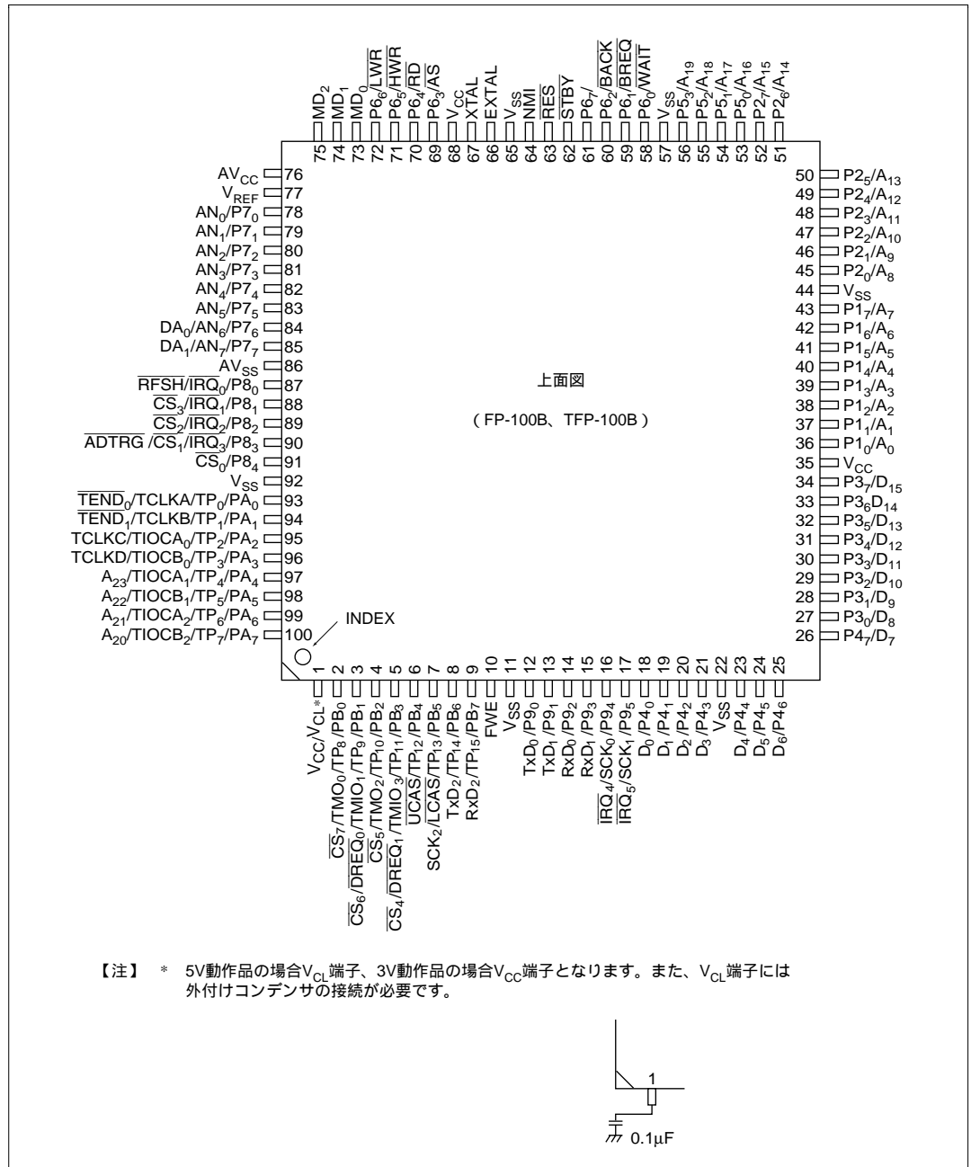
図 1.2 ピン配置図 (FP-100B、TFP-100B : 上面図)
