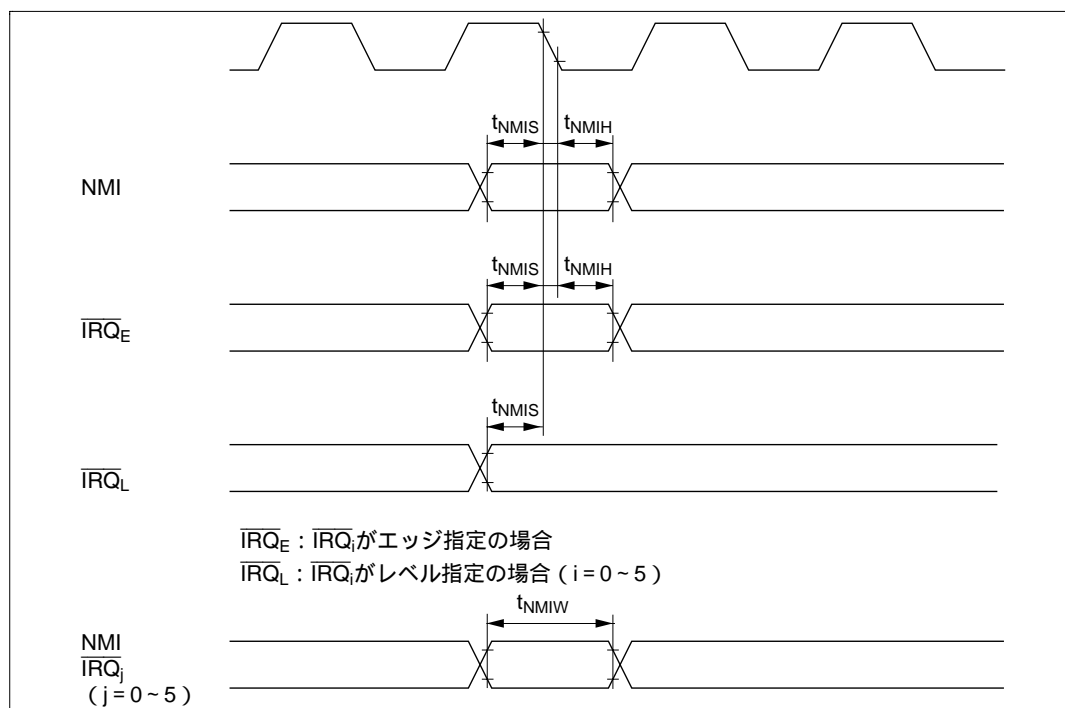
図 21.7 割り込み入力タイミング
