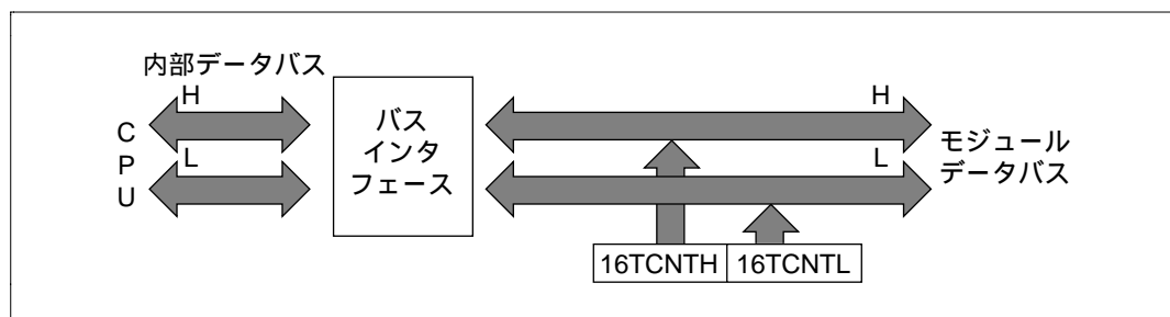
図 9.5 16TCNT のアクセス動作 [ 16TCNT CPU (ワード) ]
