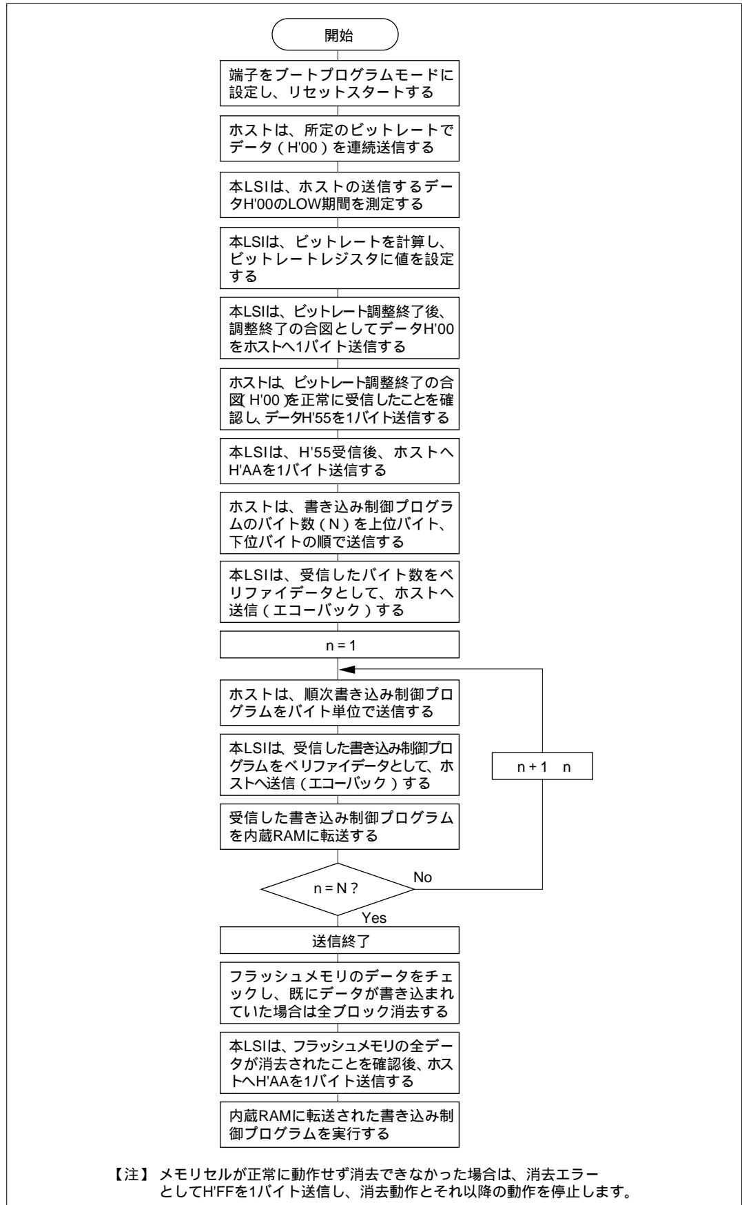
図 18.6 ブートモード実行手順
