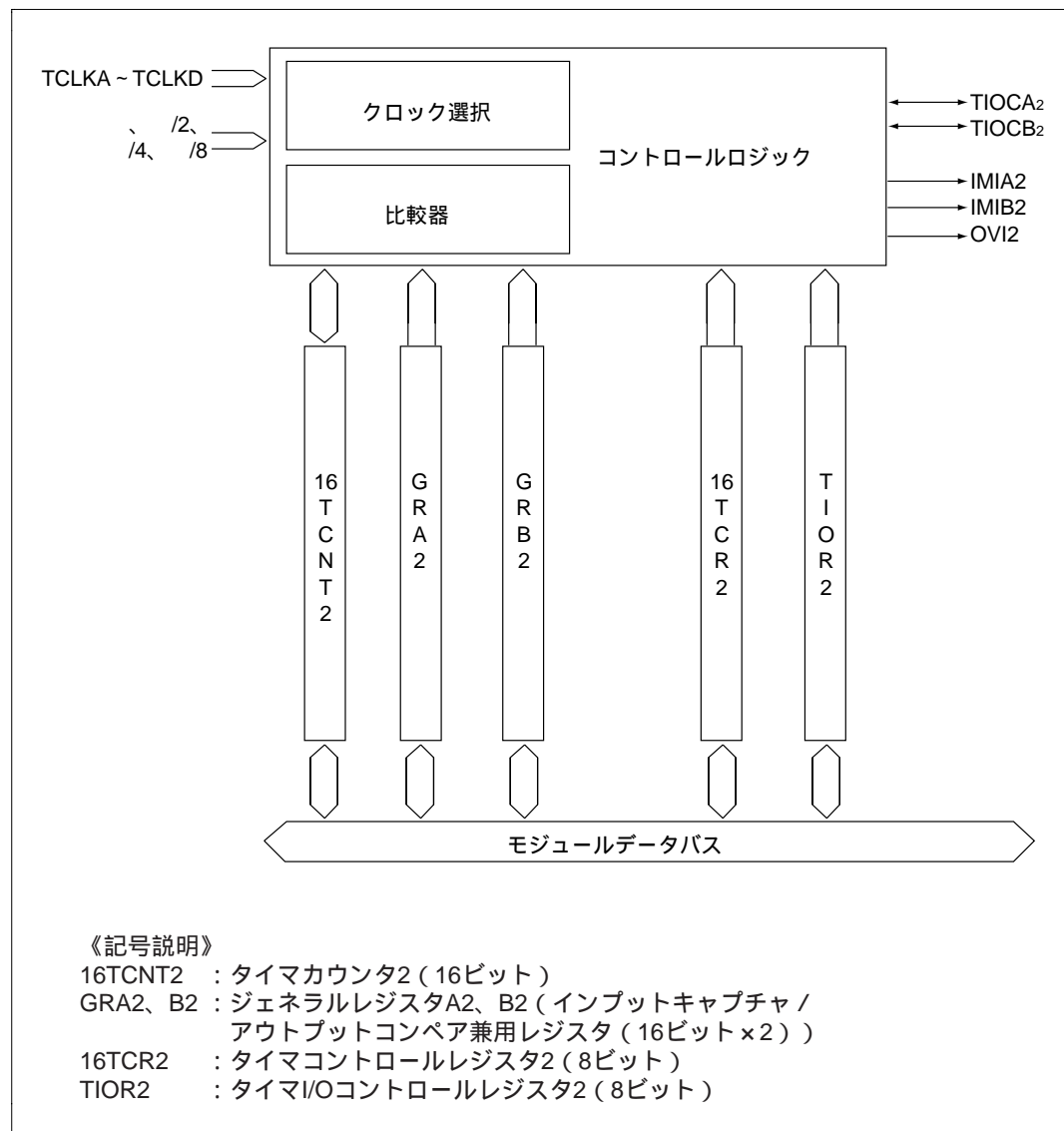
図9.3 チャンネル2のブロック図
