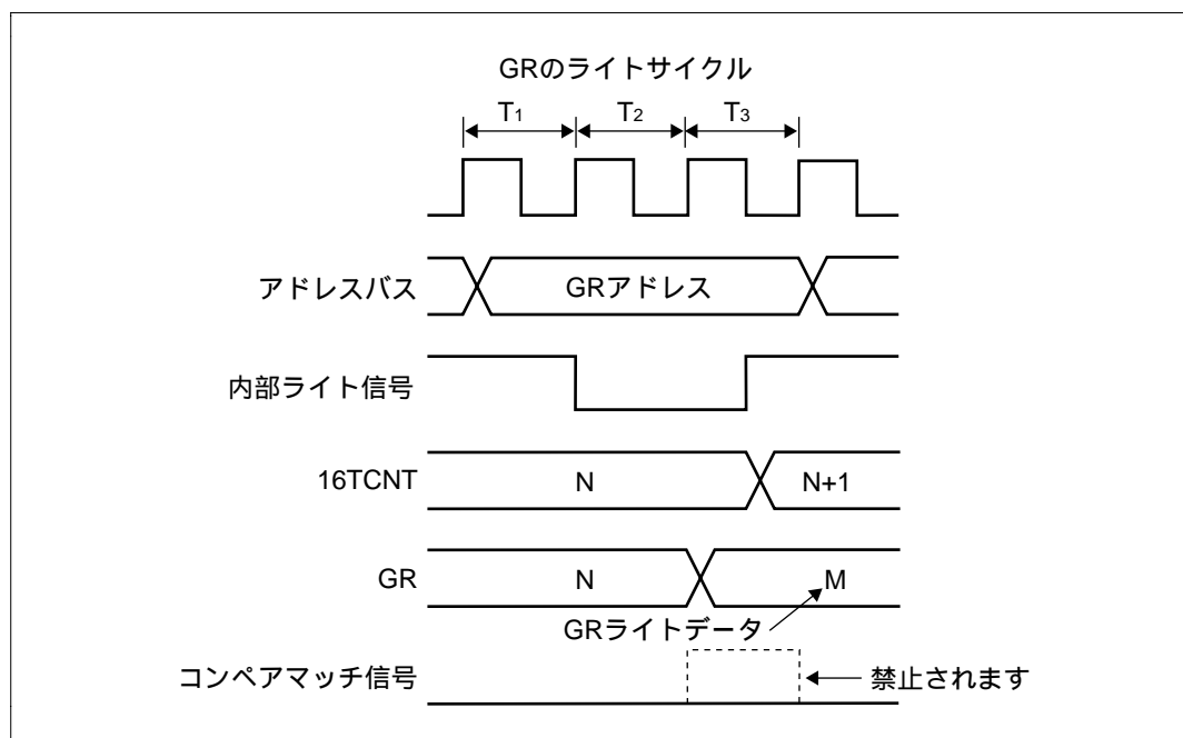
図 9.40 GR のライトとコンペアマッチの競合
