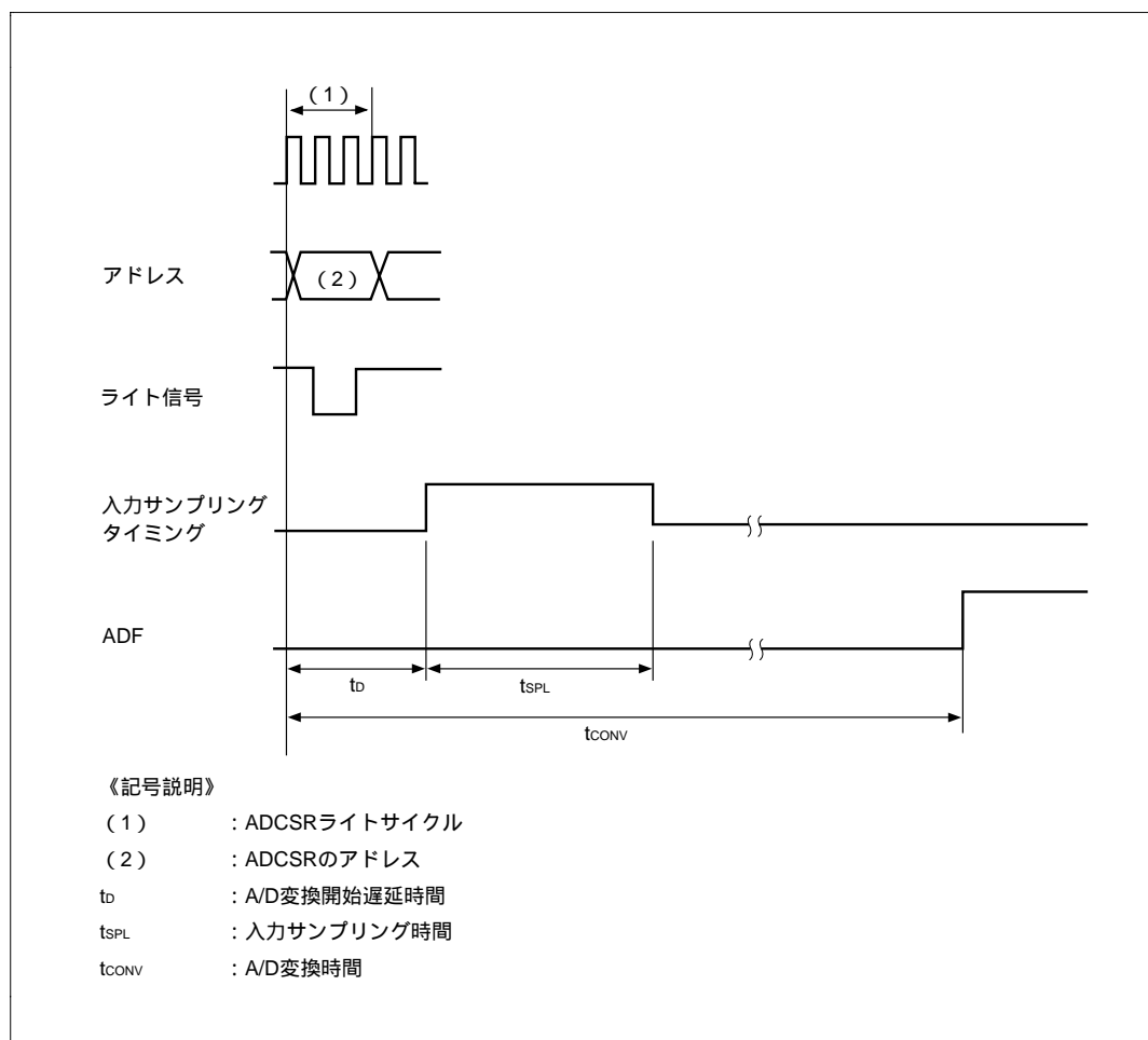
図15.5 A/D変換タイミング
