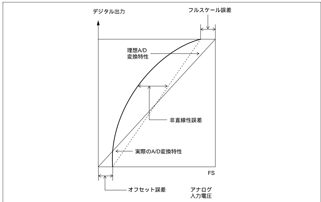
図 15.10 A/D 変換精度の定義 (2)
