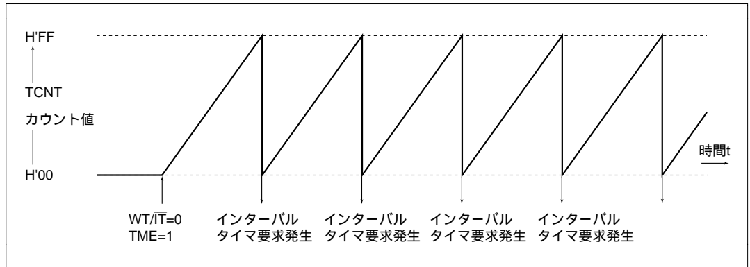
図 12.5 インターバルタイマ時の動作
