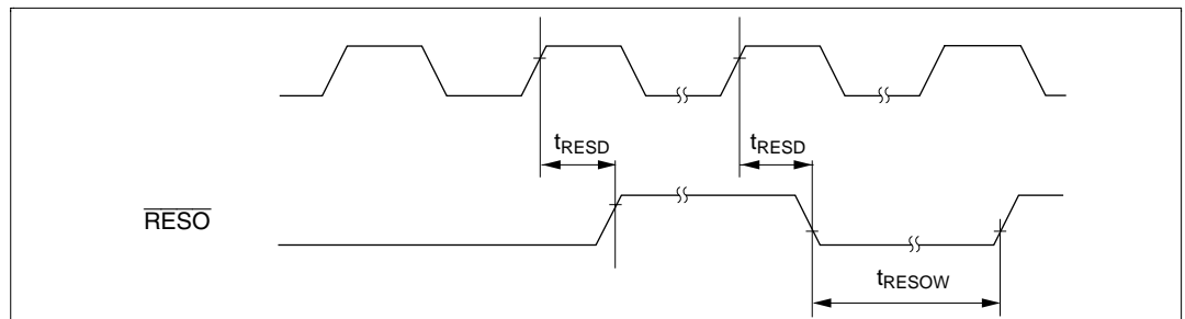
図 21.6 リセット出力タイミング*
