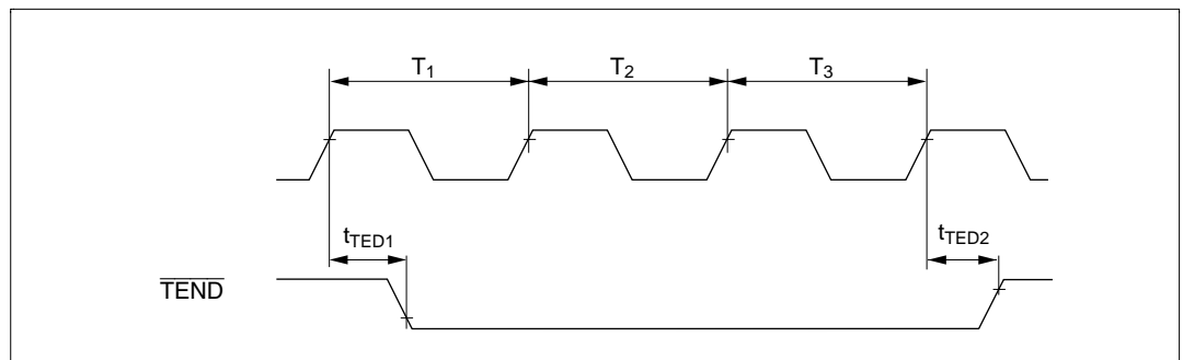
図 21.23 DMAC、 \overline{\text{TEND}} 出力タイミング / 3 ステートアクセス
