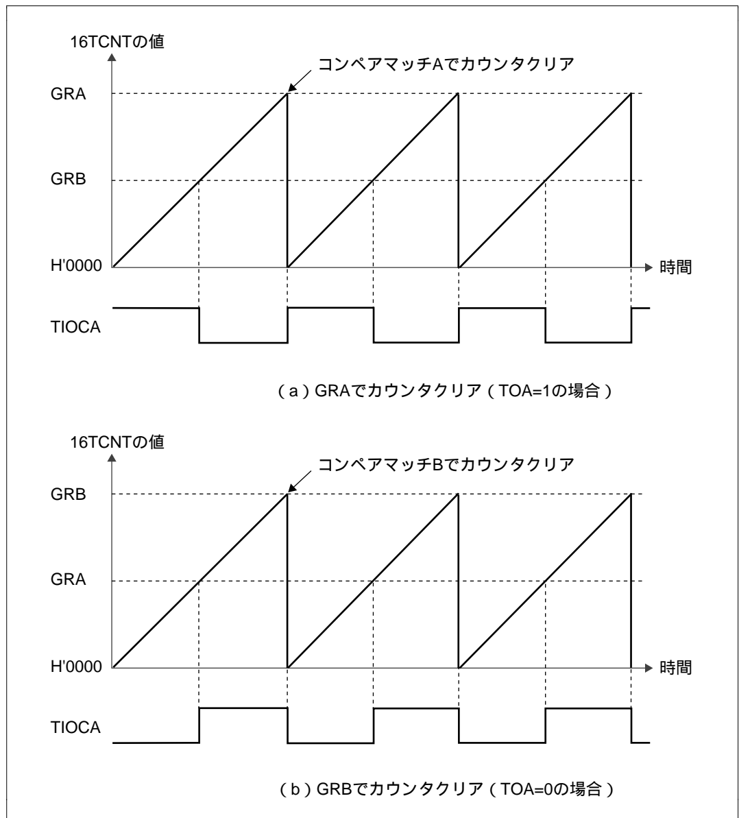
図 9.27 PWM モードの動作例 (1)
