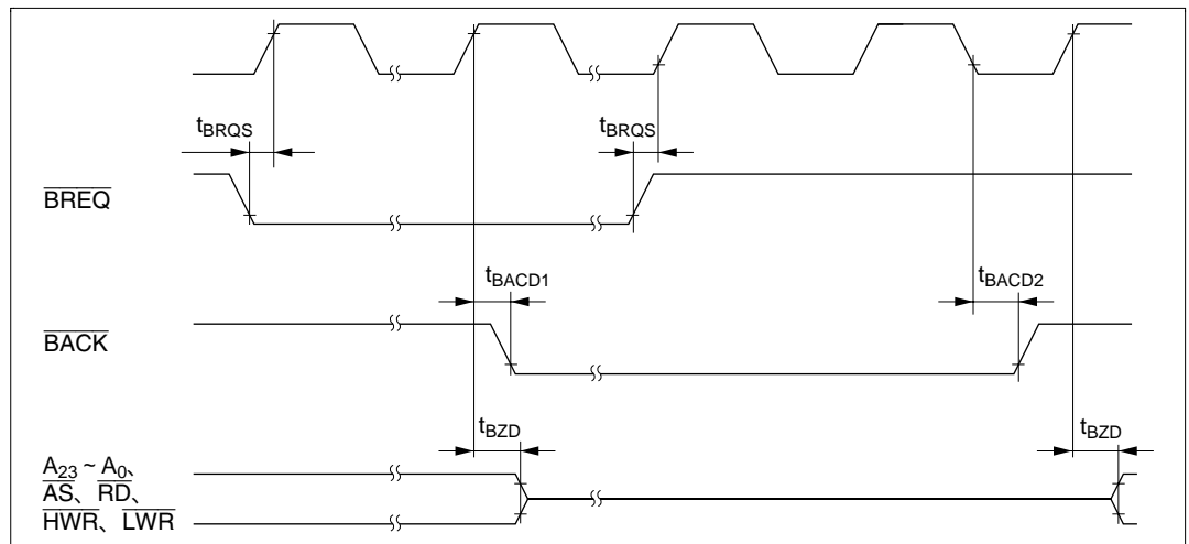
図 21.13 バスリリースモードタイミング
