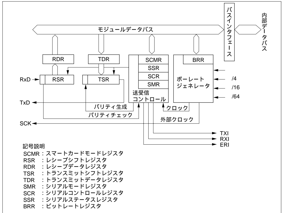
図 14.1 スマートカードインタフェースのブロック図
