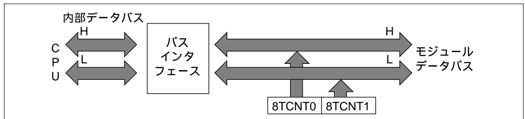
図 10.3 8TCNT のアクセス動作 [ 8TCNT CPU (ワード) ]
