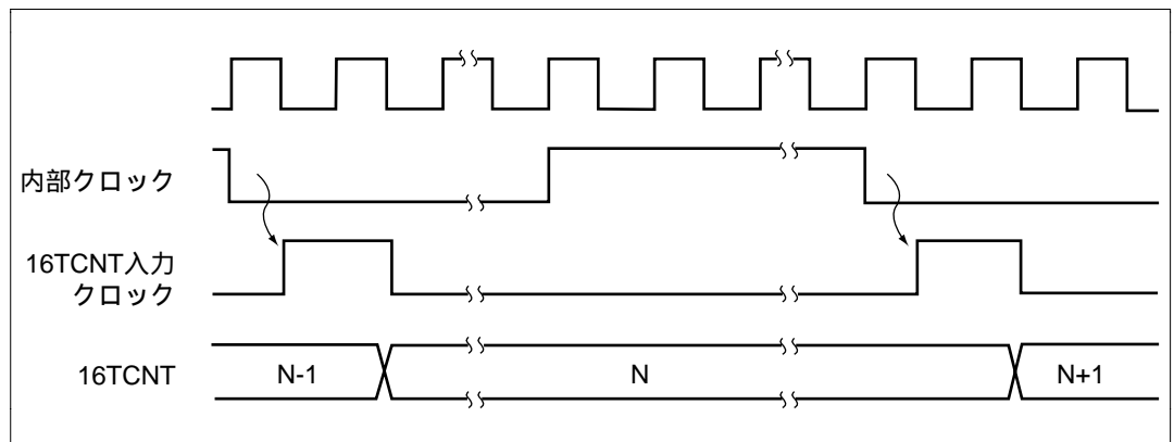
図 9.15 内部クロック動作時のカウントタイミング
