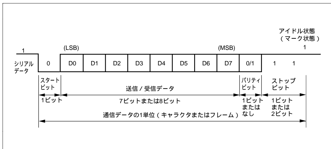
図 13.2 調歩同期式通信のデータフォーマット (8ビットデータ / パリティあり / 2ストップビットの例)
