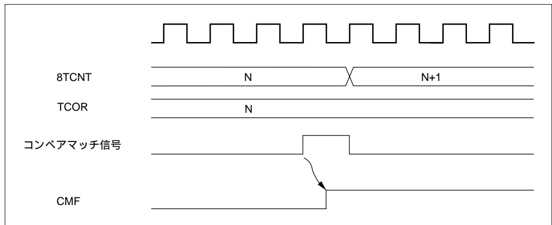
図 10.14 コンペアマッチ時の CMF フラグセットタイミング
