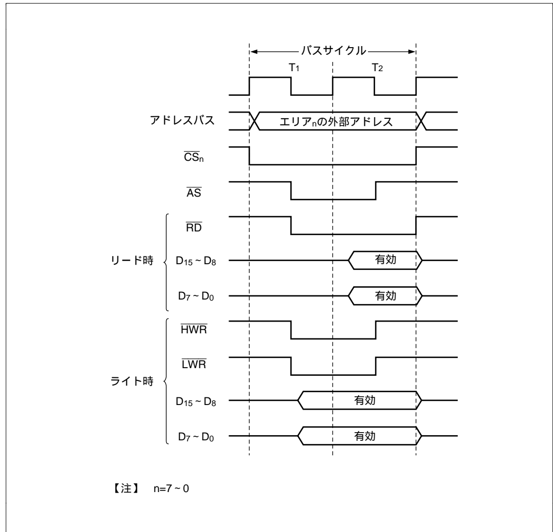
図 6.16 16ビット2ステータアクセス空間のバス制御信号タイミング (ワードアクセス)
