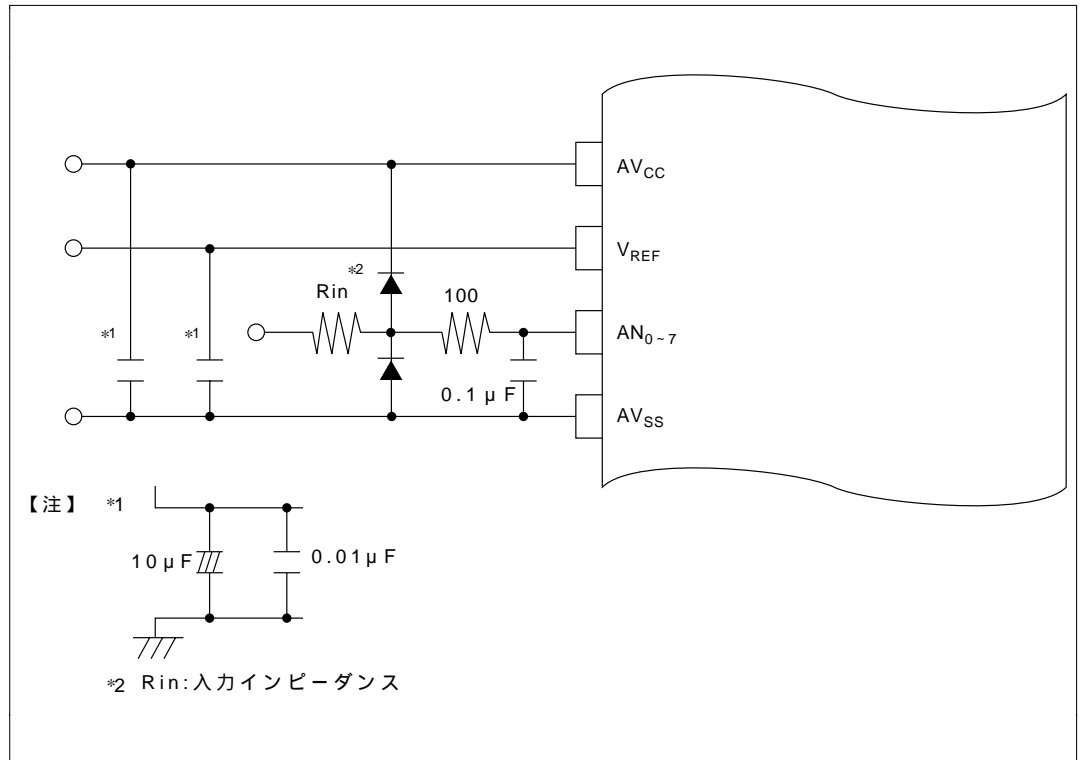
図 15.7 アナログ入力保護回路の例
