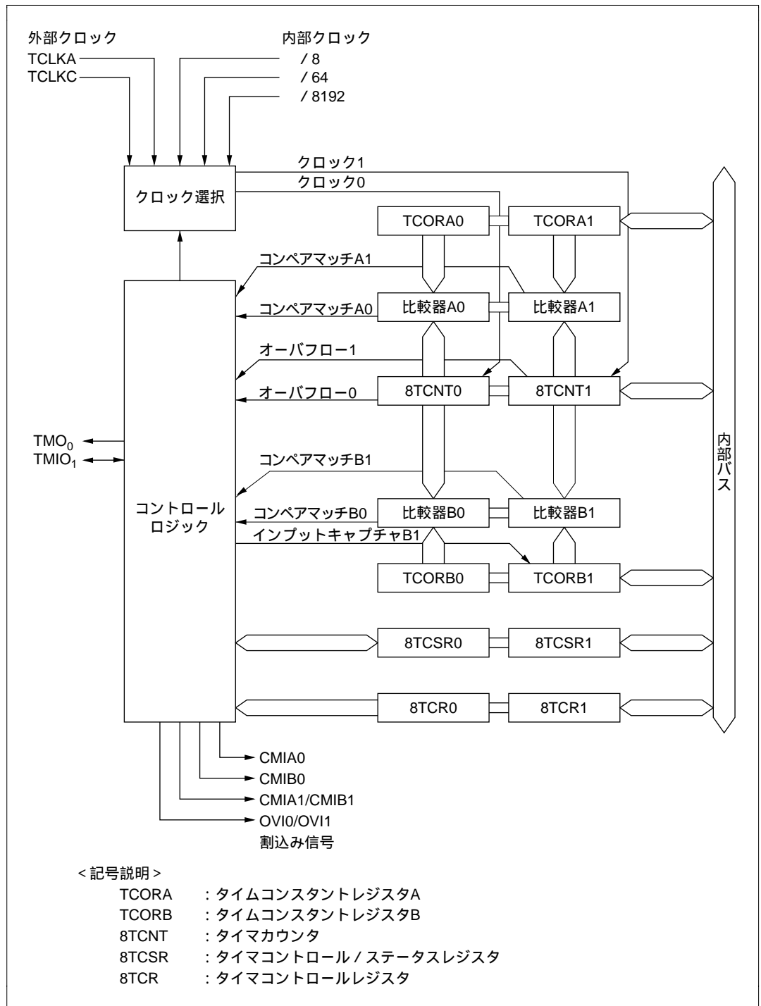
図10.1 8ビットタイマのブロック図(2チャンネル分:グループ0)
