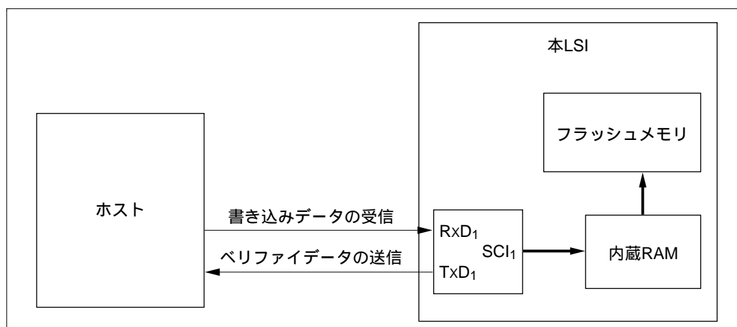
図 18.5 ブートモード時のシステム構成図
