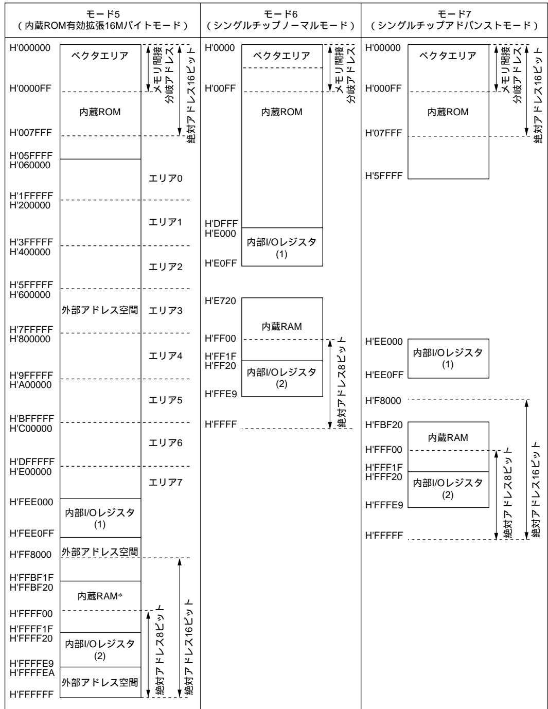
図 3.1 H8/3068F の各動作モードにおけるメモリマップ (EMC ビット=1 のとき) (2)
