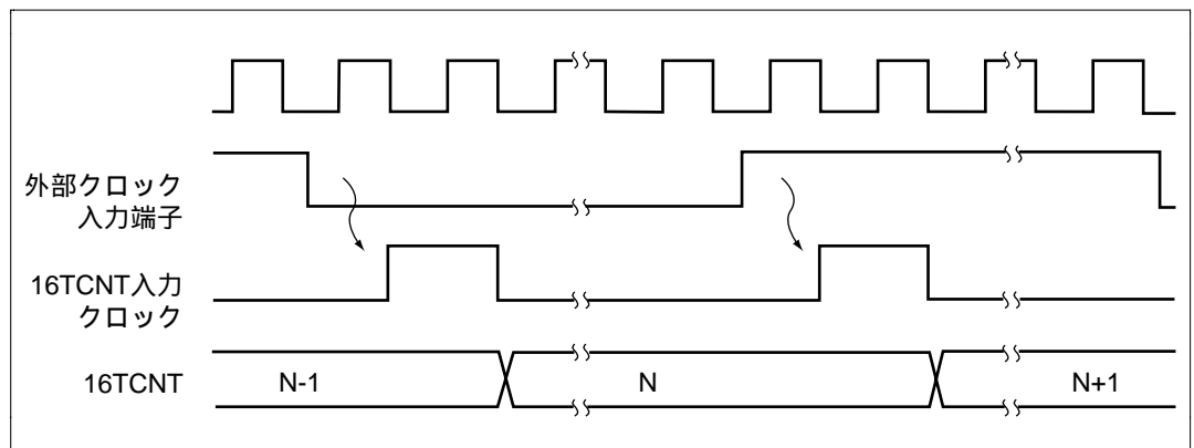
図 9.16 外部クロック動作時のカウントタイミング (両エッジ検出の場合)
