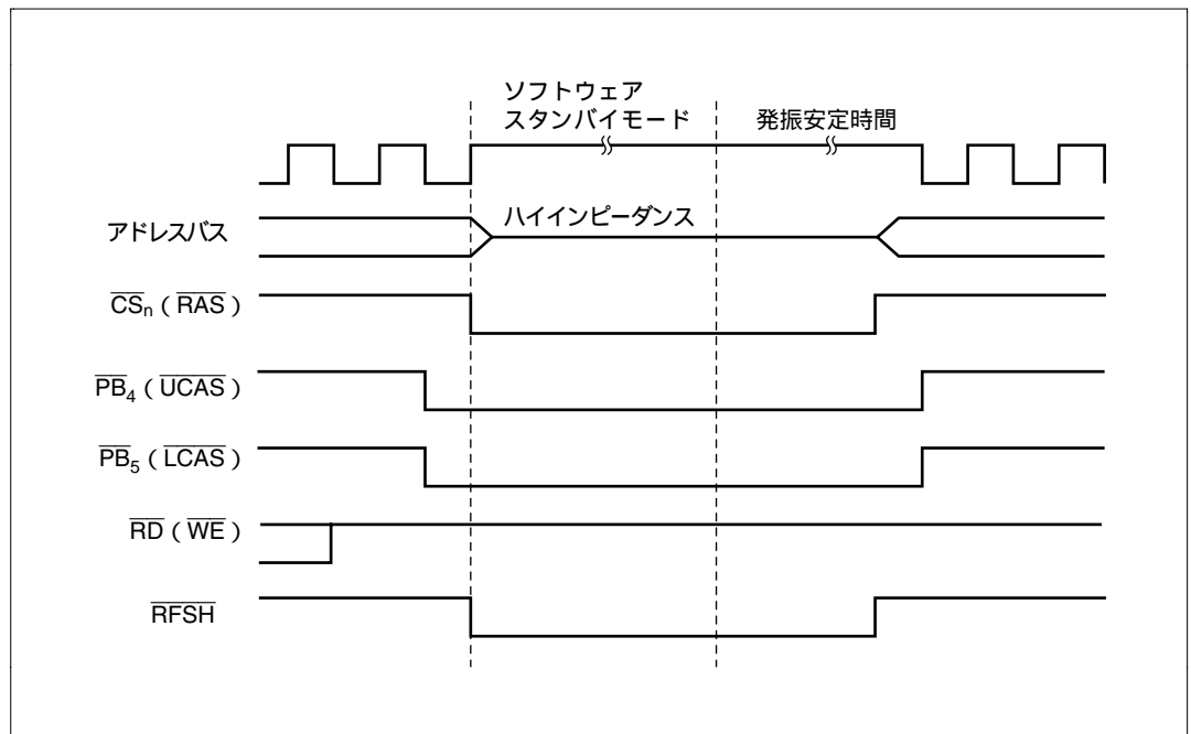
図 6.30 セルフリフレッシュタイミング (CSEL=0 の場合)
