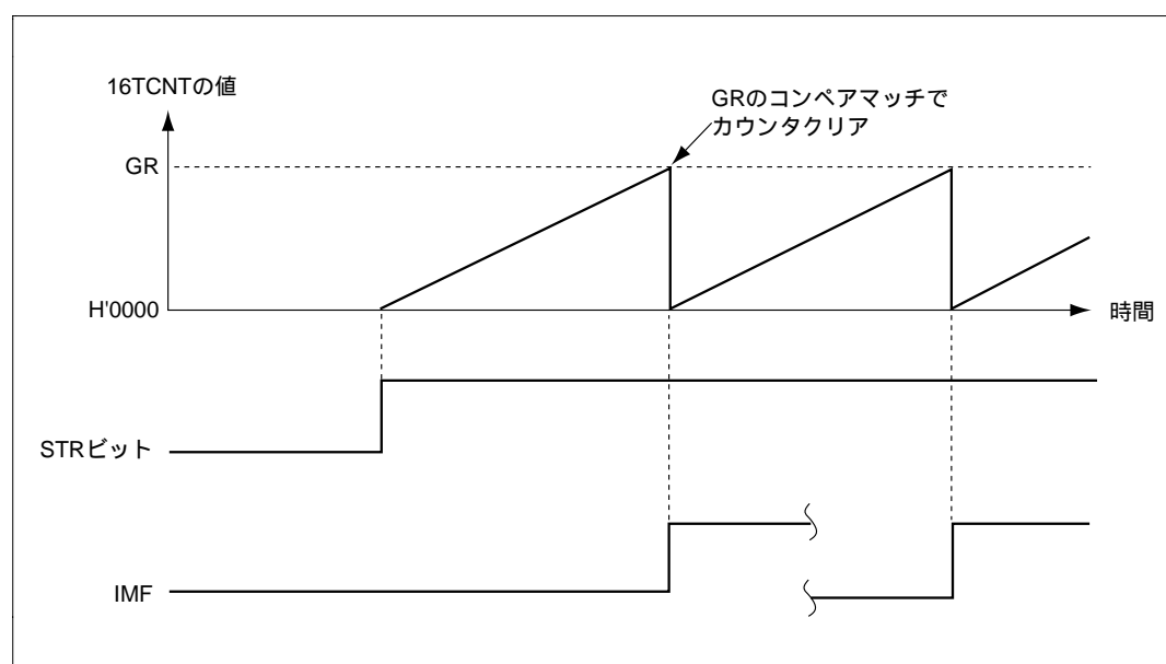
図 9.14 周期カウンタの動作
