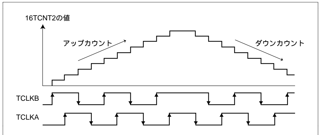
図 9.30 位相計数モードの動作例
