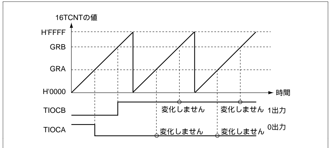
図 9.18 0出力、1出力の動作例 (TOA=1、TOB=0の場合)
