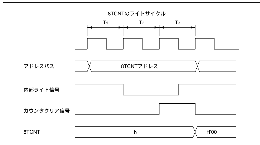
図 10.18 8TCNTのライトとクリアの競合
