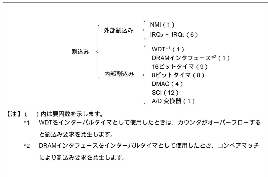
図 4.5 割込み要因と要因数
