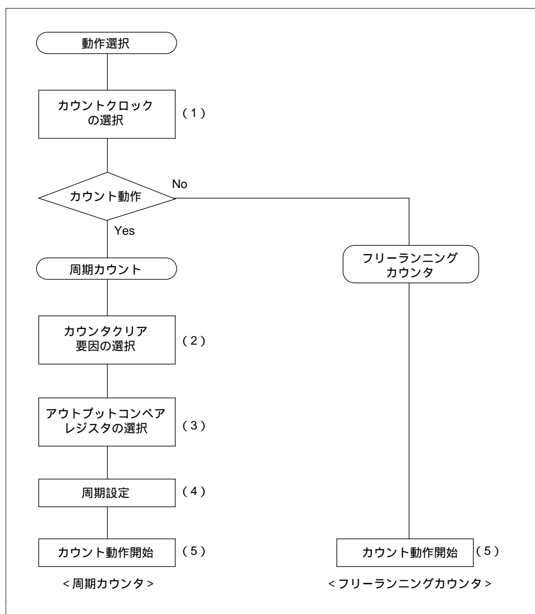
図 9.12 カウント動作設定手順例
