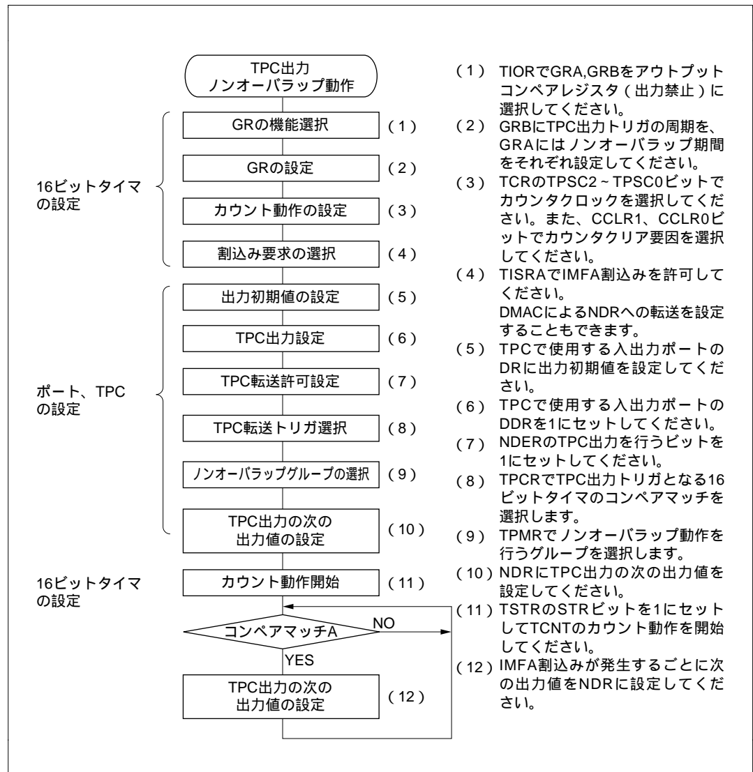
図 11.6 TPC 出力ノンオーバーラップ動作の設定手順例
