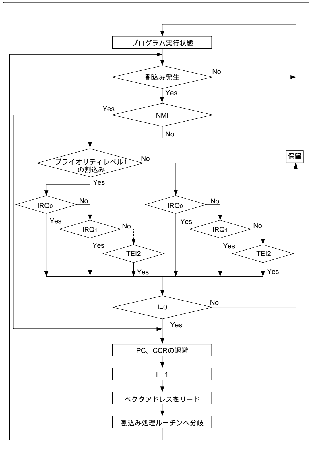
図 5.4 UE = 1 の場合の割り込み受けまでのフロー
