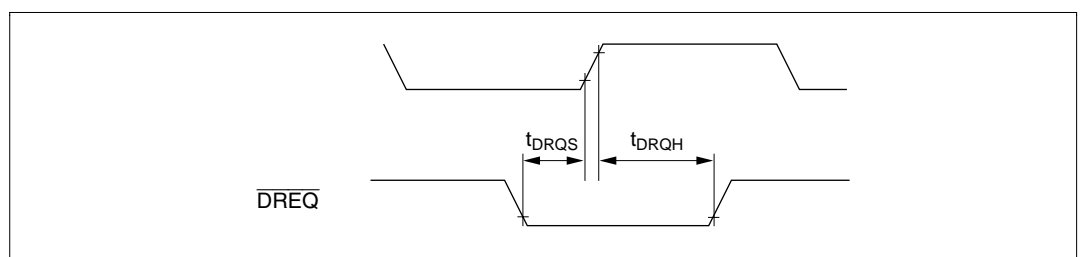
図 21.24 DMAC、 \overline{\text{DREQ}} 入力タイミング
