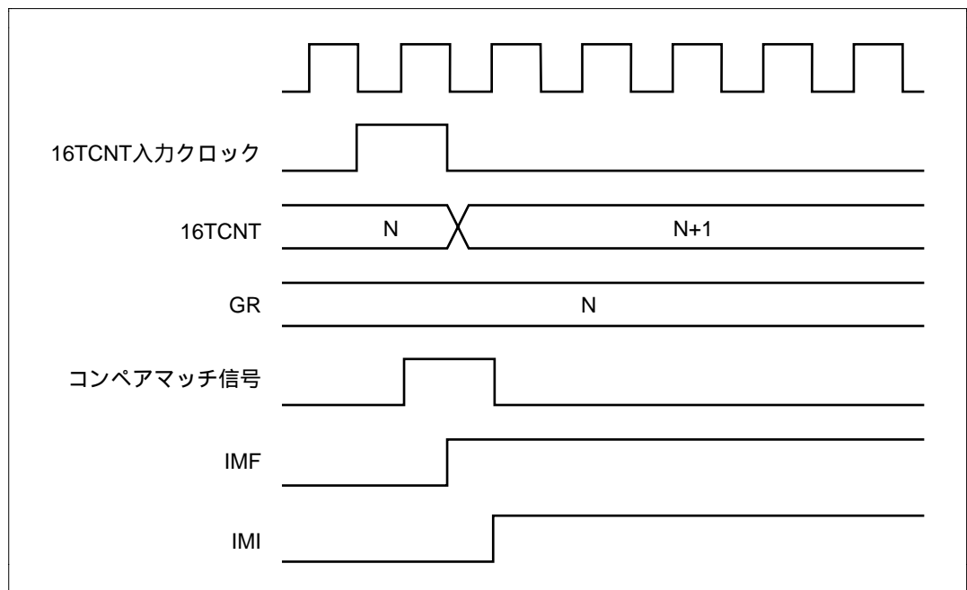
図 9.33 コンペアマッチ時の IMFA、IMFB フラグのセットタイミング
