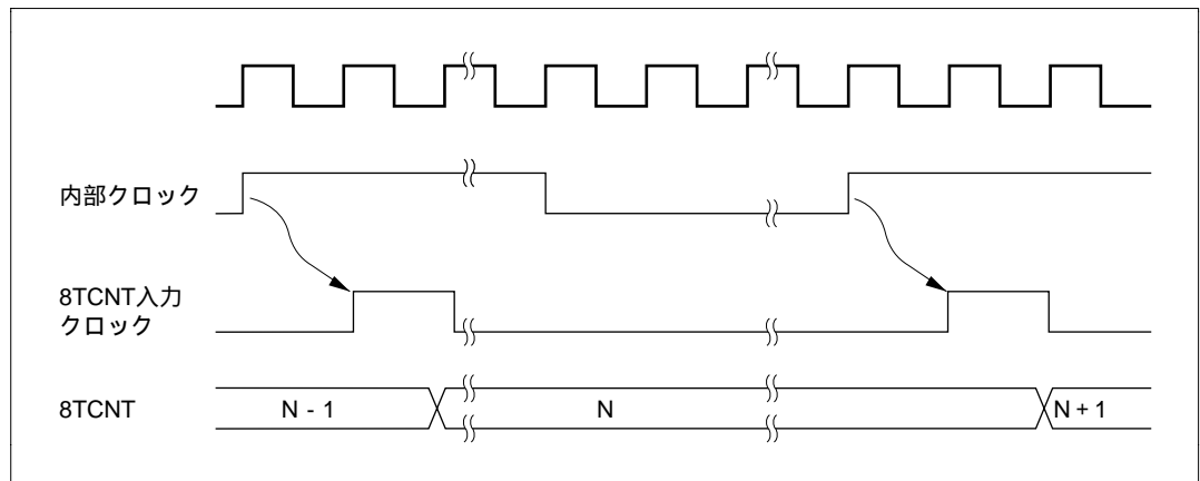
図 10.8 内部クロック動作時のカウントタイミング
