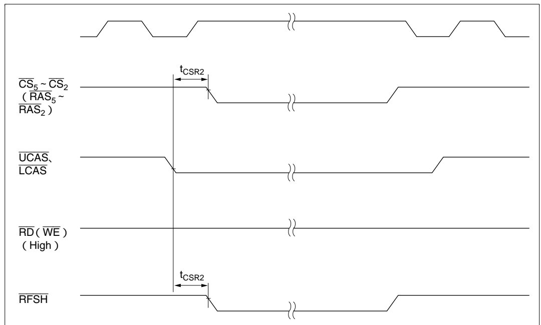
図 21.16 DRAMバスタイミング (セルフリフレッシュ)
