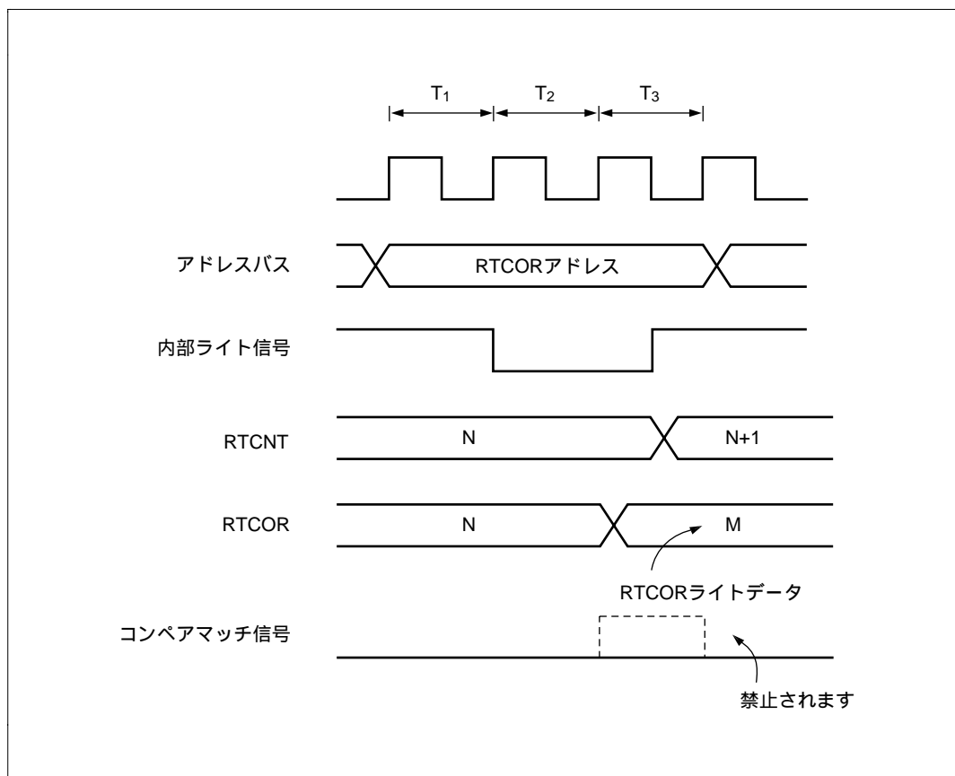
図 6.41 RTCOR のライトとコンペアマッチの競合
