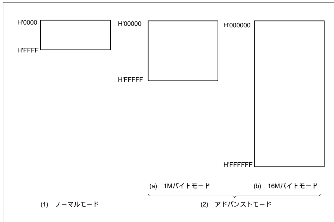
図2.2 メモリマップ
