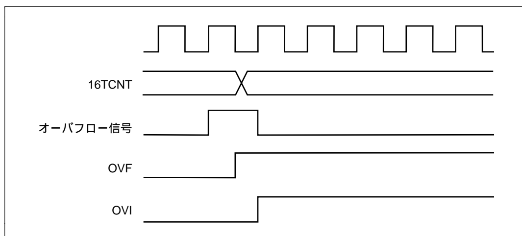
図 9.35 OVF のセットタイミング
