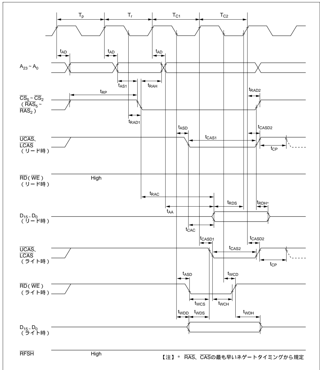
図 21.14 DRAMバスタイミング (リード/ライト時)
