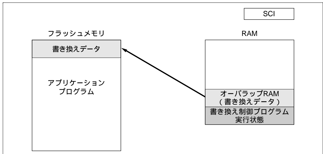
図 18.4 ユーザプログラムモードのオーバーラップ RAM データの書き込み
