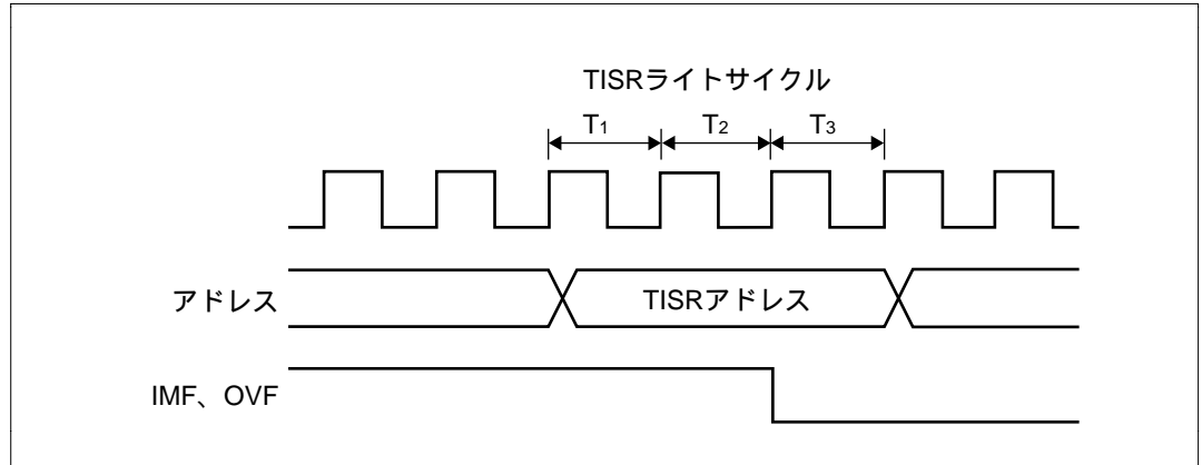
図 9.36 ステータスフラグのクリアタイミング
