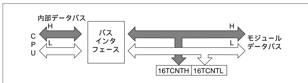
図 9.6 16TCNTH のアクセス動作 [ CPU 16TCNTH (上位バイト) ]
