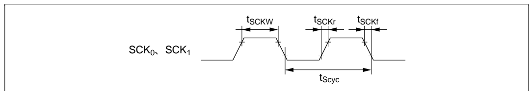
図 21.20 SCI 入力クロックタイミング
