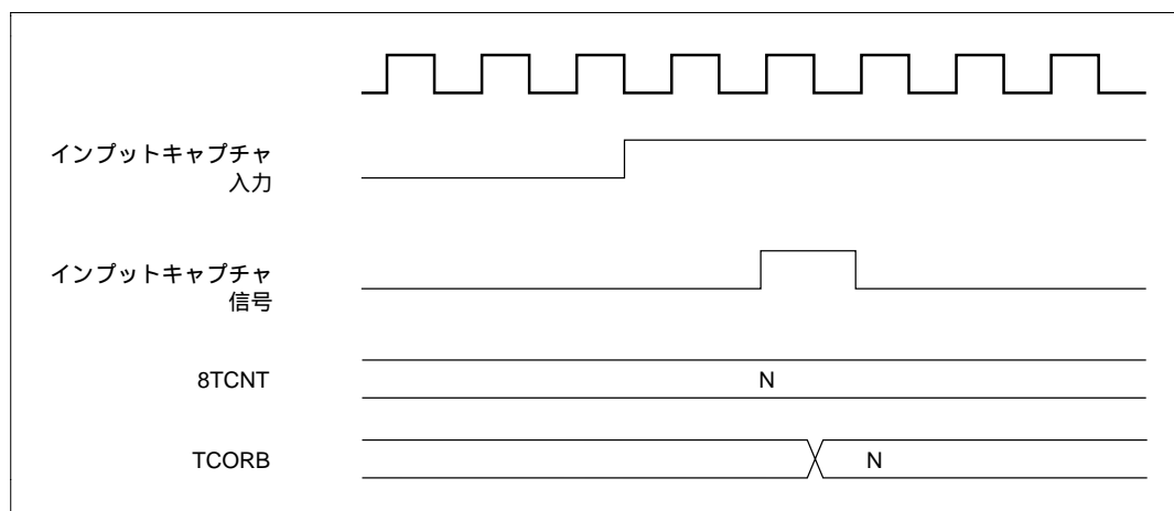
図 10.13 インพุットキャプチャ入力信号タイミング
