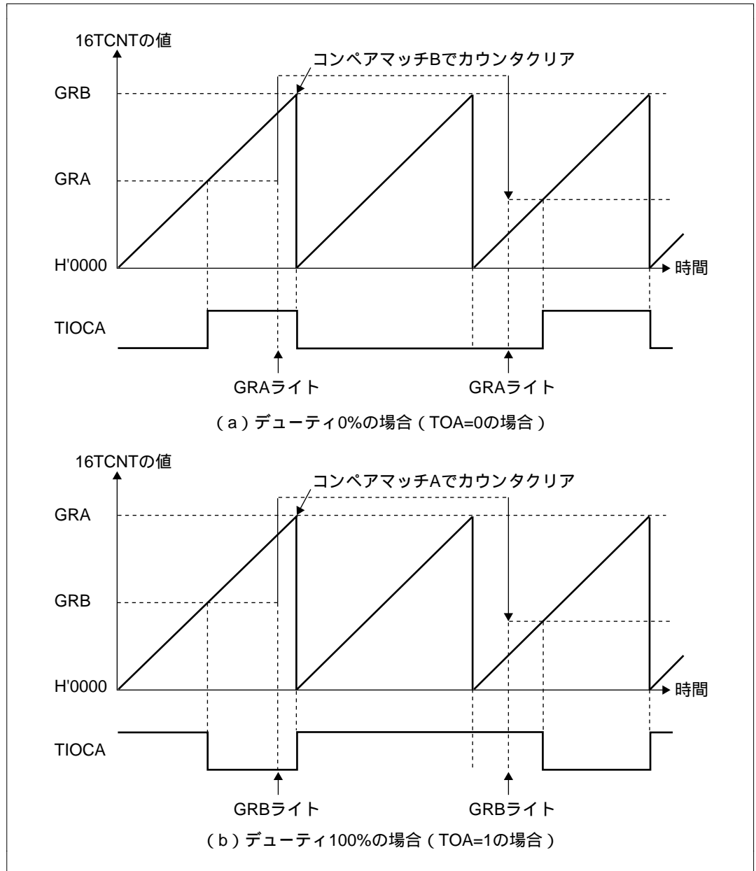
図9.28 PWMモードの動作例(2)
