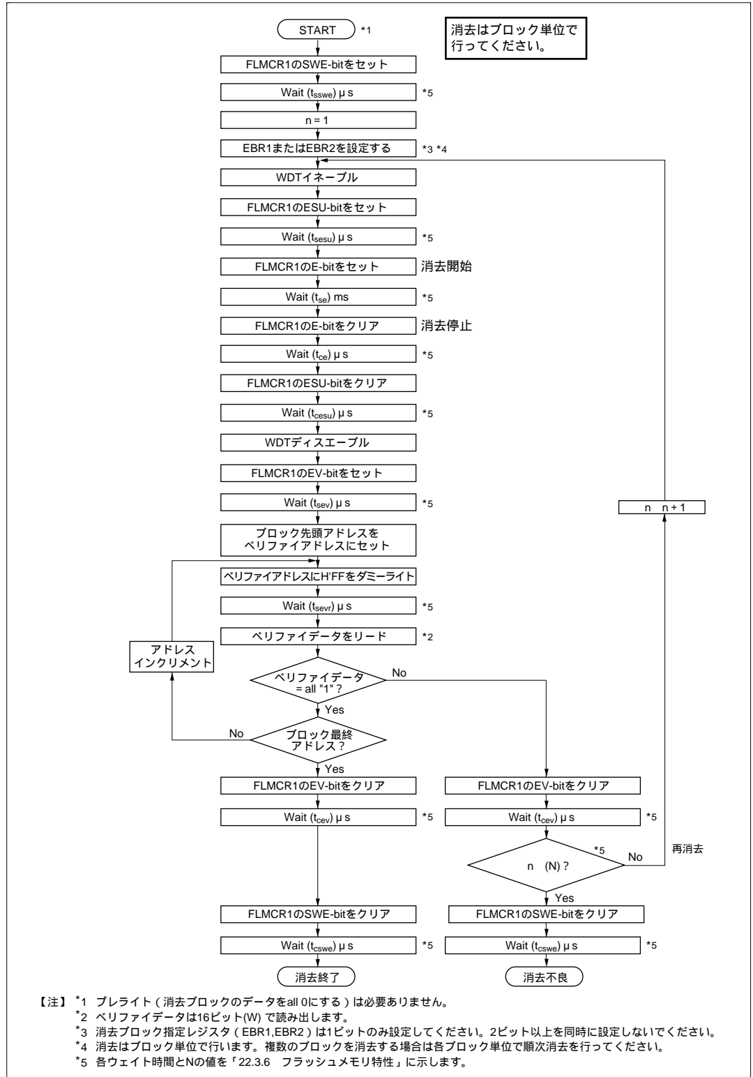
図 18.11 イレース/イレースベリファイフロー（単一ブロック消去）
