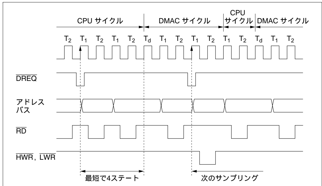
図 7.16 ノーマルモード時の \overline{\text{DREQ}} 端子の立下がりエッジで DMAC 起動タイミング
