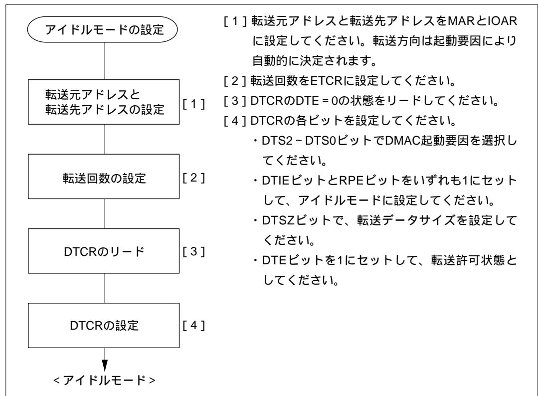
図 7.5 アイドルモードの設定手順例
