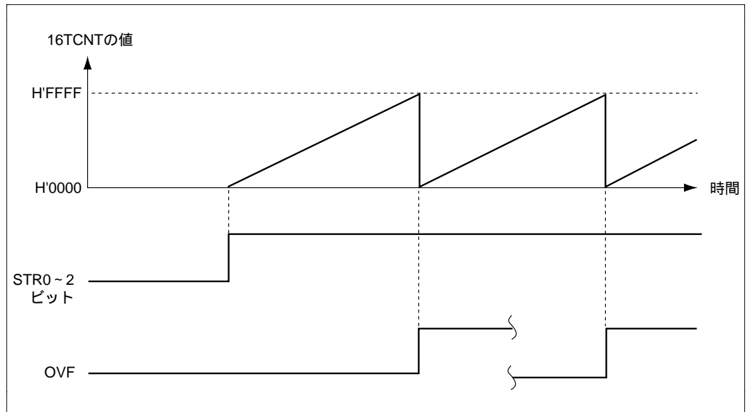
図 9.13 フリーランニングカウンタの動作
