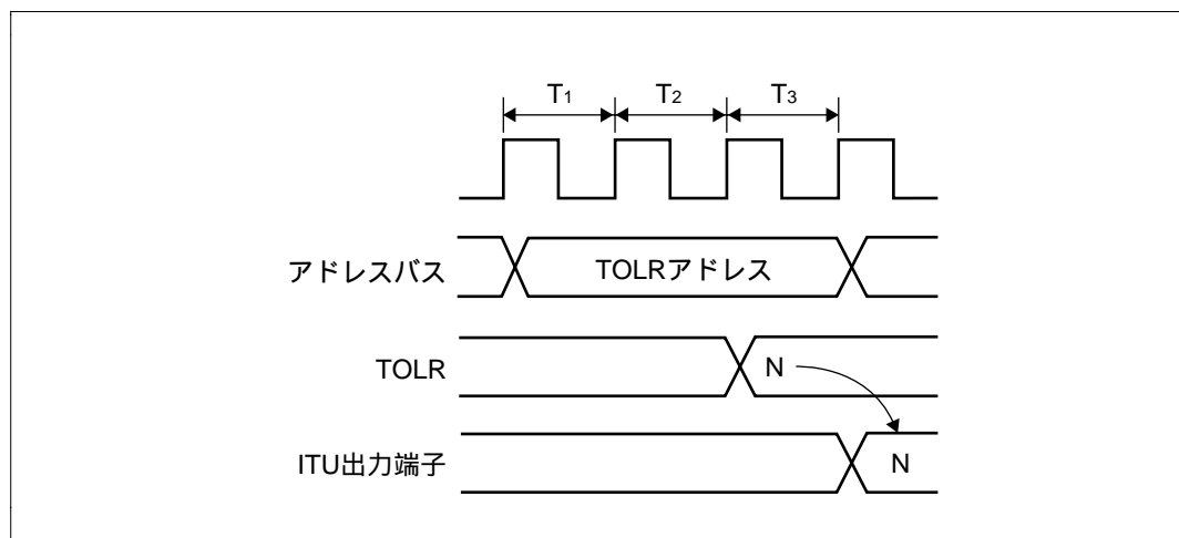
図 9.32 TOLR へのライトによる 16 ビットタイマ出力初期値設定タイミング
