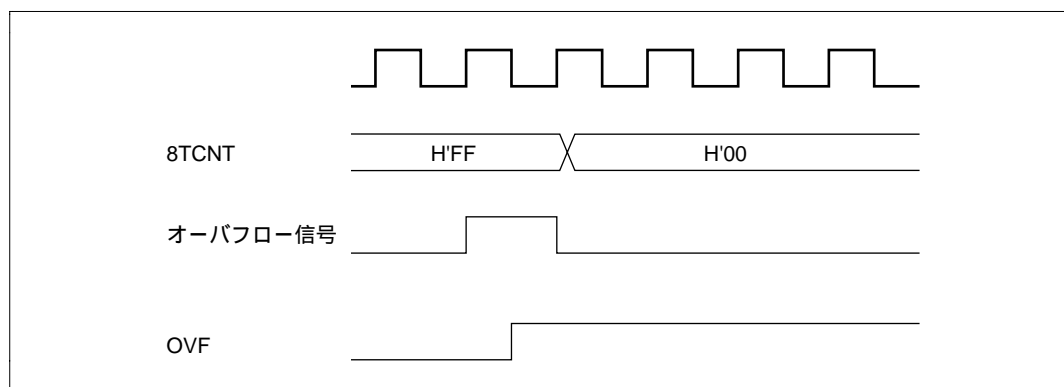
図 10.16 OVF のセットタイミング
