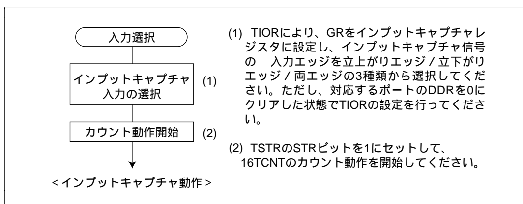
図 9.21 インพุットキャプチャ動作の設定手順例
