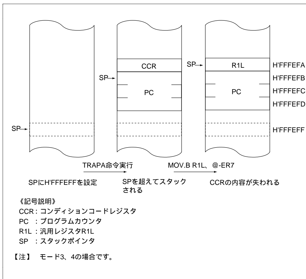
図 4.7 SP を奇数に設定したときの動作
