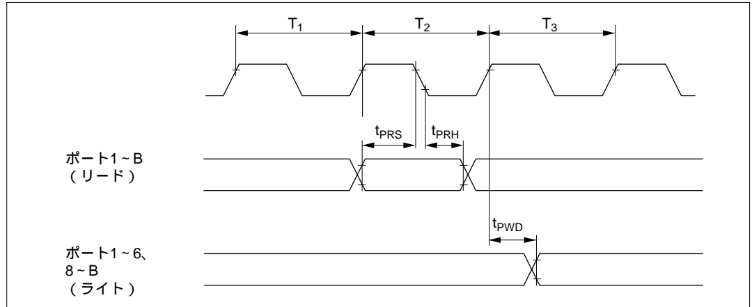
図 21.17 TPC、I/Oポート入出力タイミング
