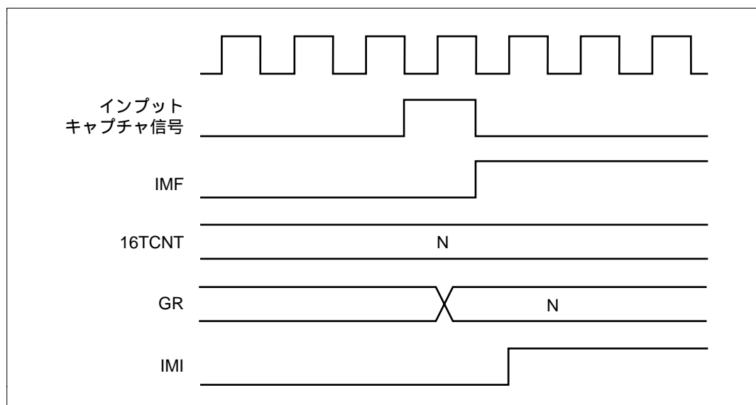
図 9.34 インพุットキャプチャ時の IMFA、IMFB フラグのセットタイミング
