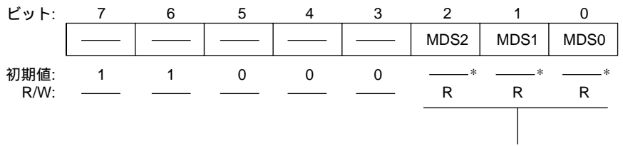
モードセレクト2~0
