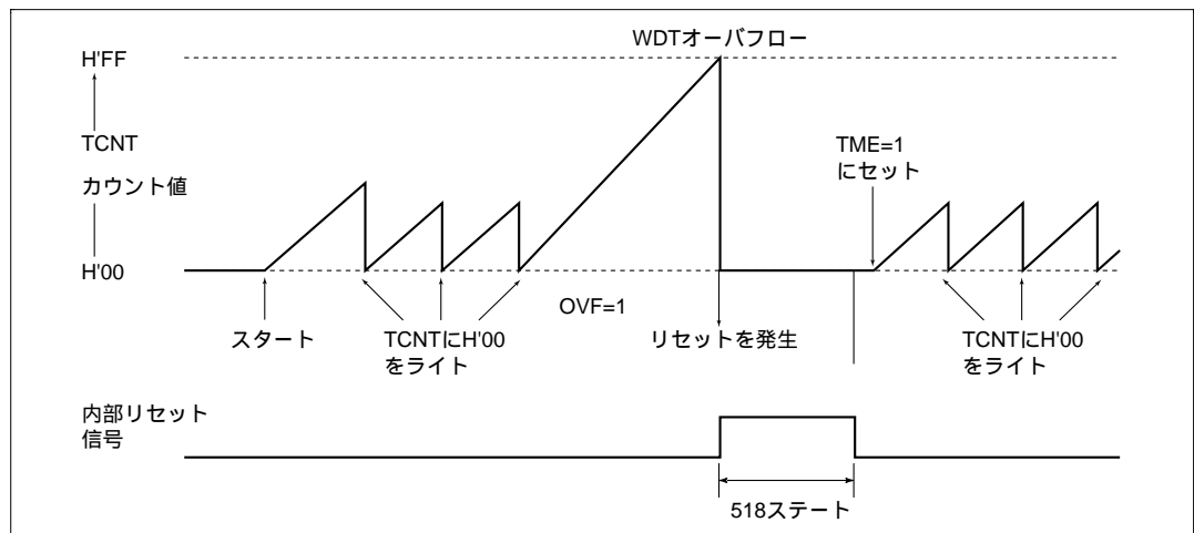
図 12.4 ウォッチドッグタイマモード時の動作
