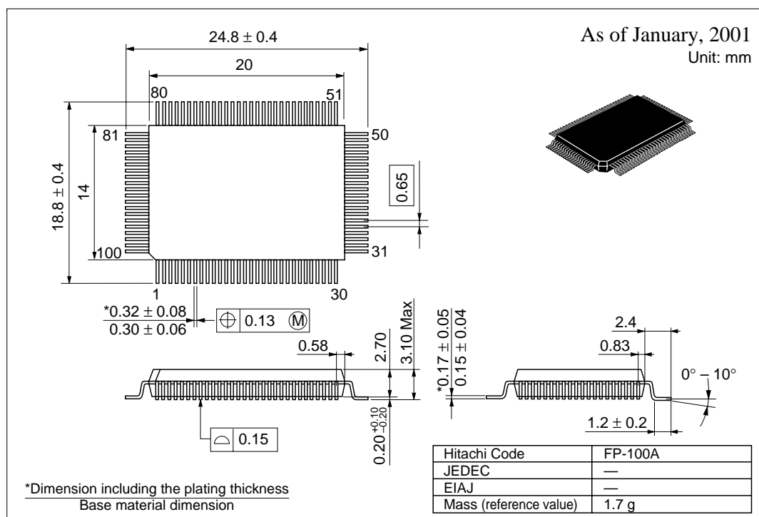
図 G.3 外形寸法図 (FP-100A) 単位 : mm
