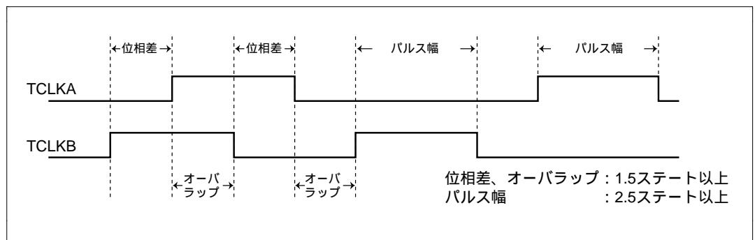
図 9.31 位相計数モード時の位相差、オーバーラップおよびパルス幅
