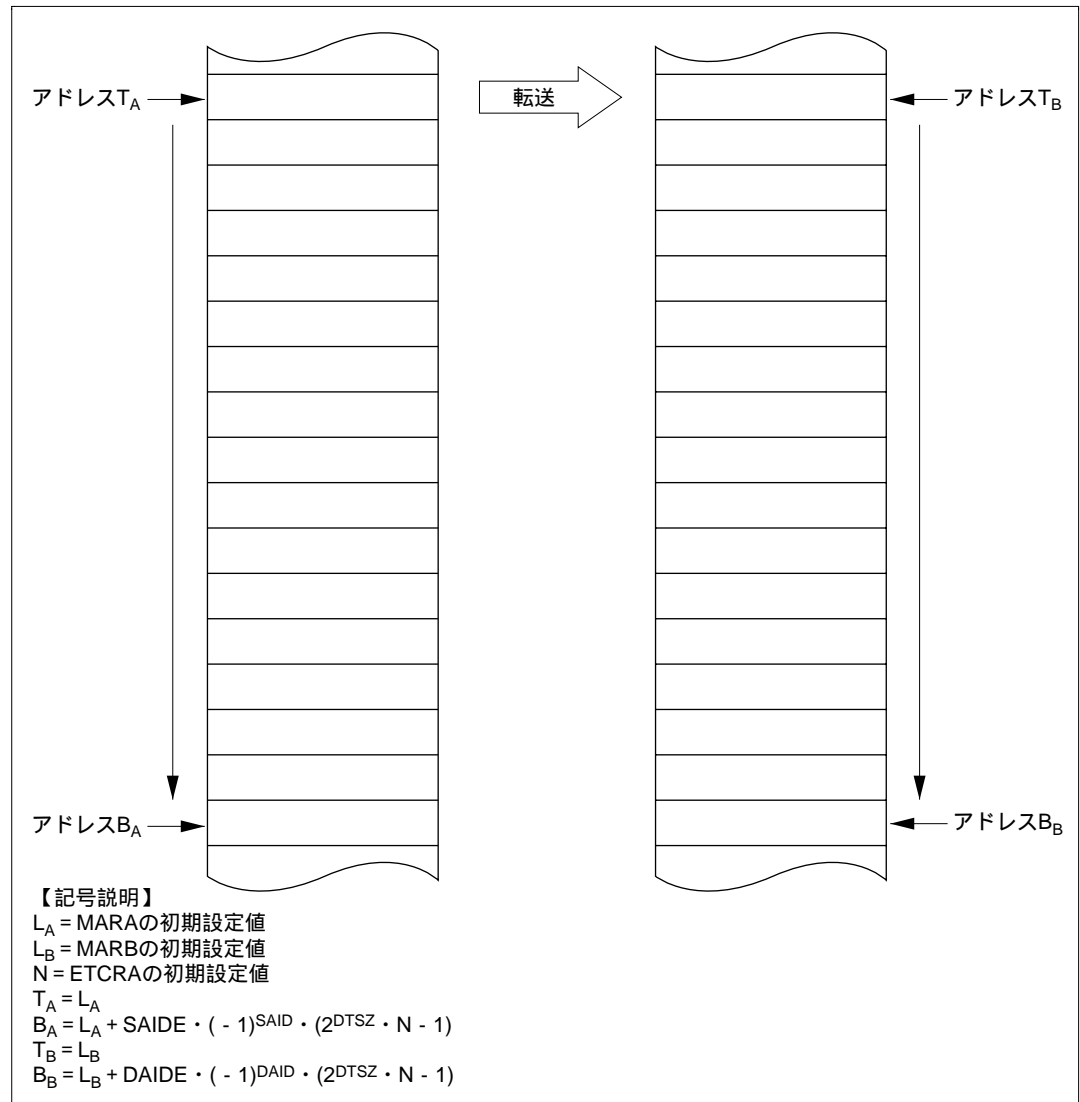
図 7.8 ノーマルモードの動作
