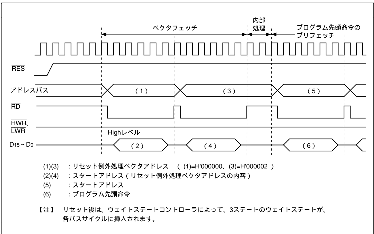
図 4.3 リセットシーケンス (モード 2、4)
