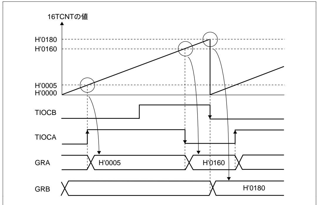
図 9.22 インพุットキャプチャ動作例
