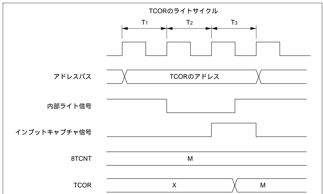
図 10.23 TCOR とインพุットキャプチャの競合
