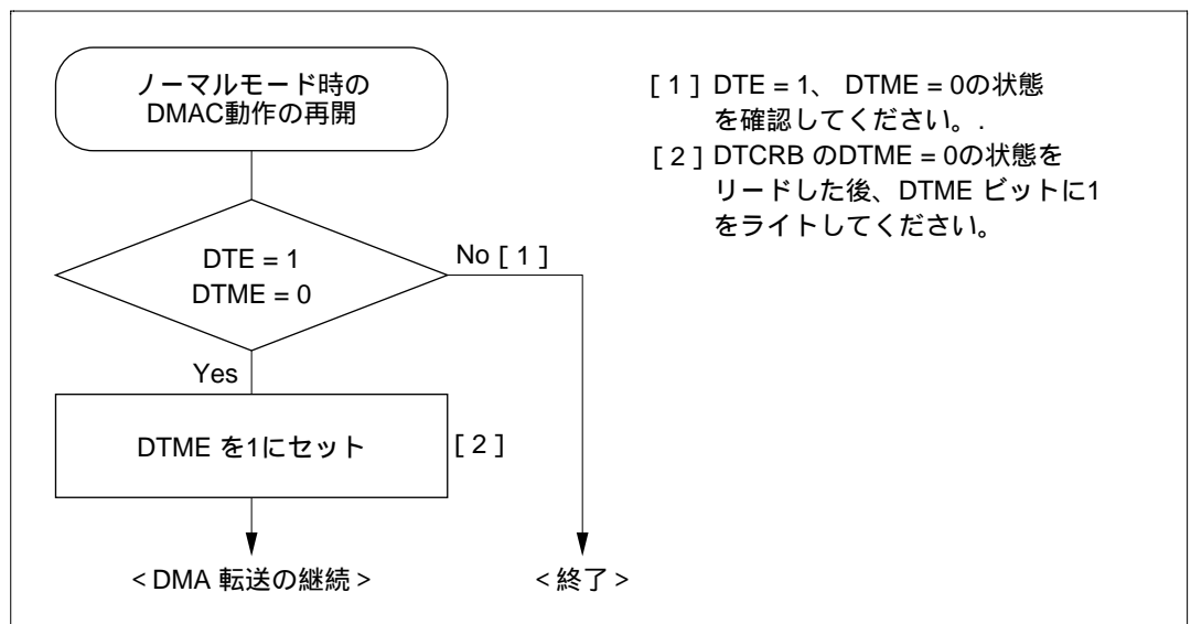
図 7.21 NMI 割込みにより停止した DMAC 動作再開手順例
