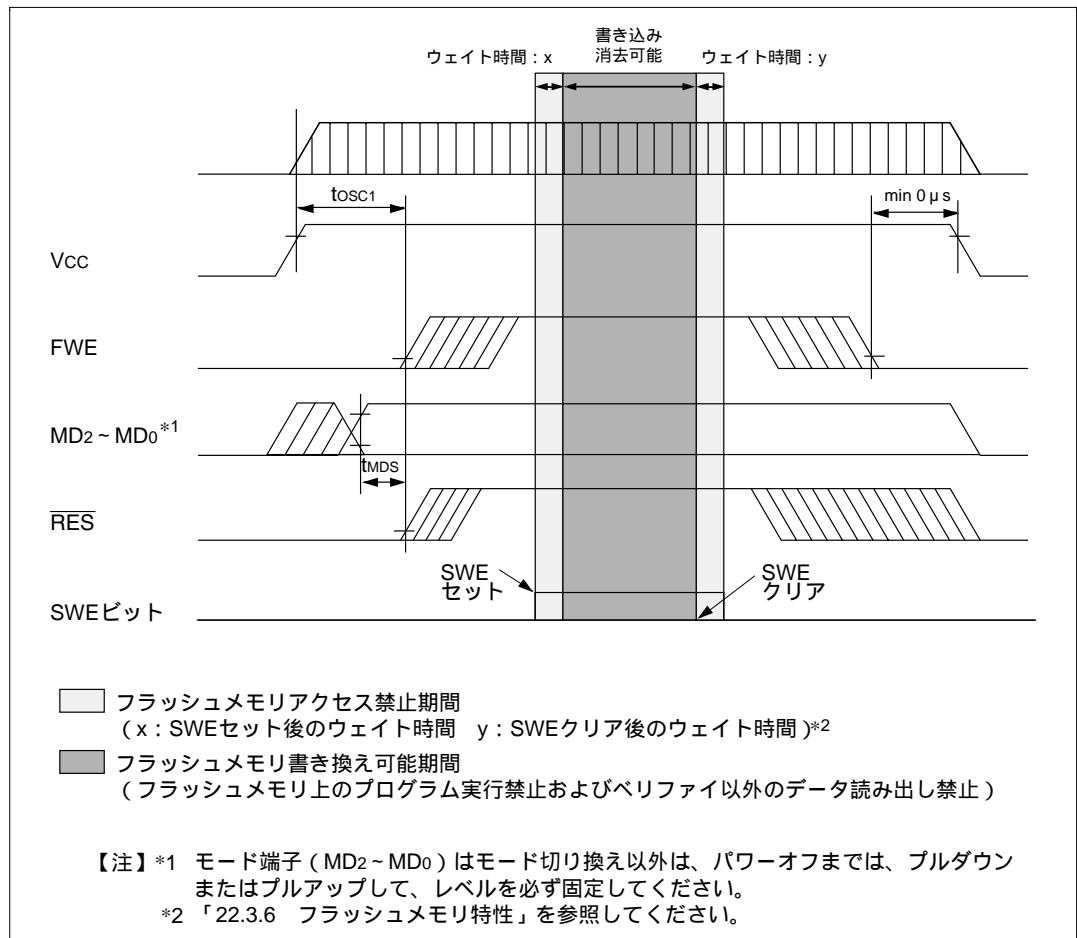
図 18.17 電源投入 / 切断タイミング (ユーザプログラムモード)
