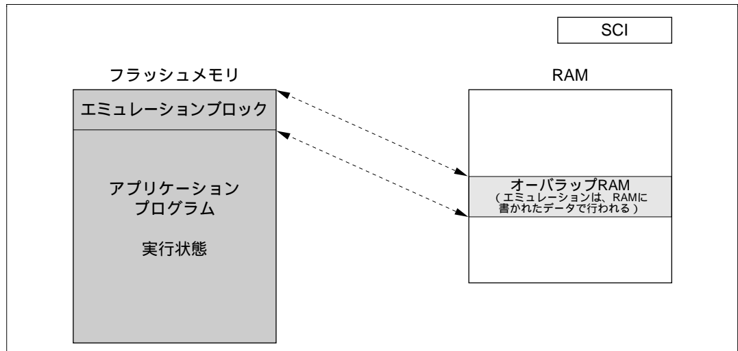
図 18.3 ユーザモード、ユーザプログラムモードのオーバーラップ RAM データの読み出し
