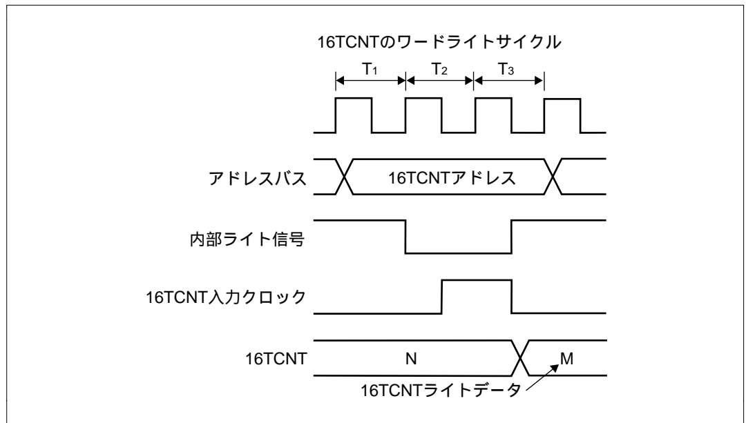
図9.38 16TCNTのワードライトとカウントアップの競合
