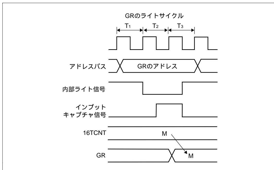
図 9.44 GRのライトと入力キャプチャの競合
