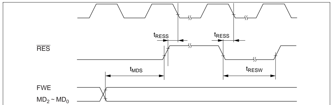
図 21.5 リセット入力タイミング
