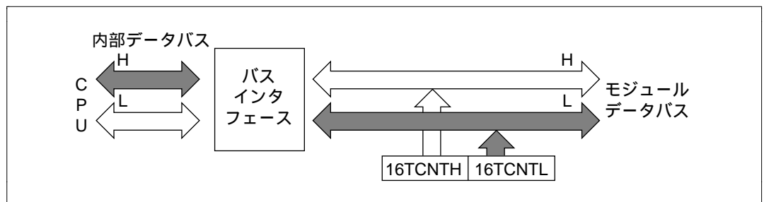
図 9.9 16TCNTLのアクセス動作 [16TCNTL CPU (下位バイト)]
