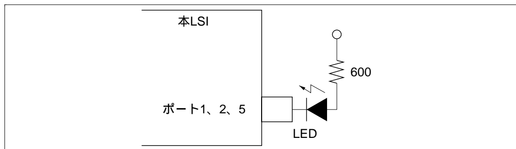
図 21.2 LED 回路例
