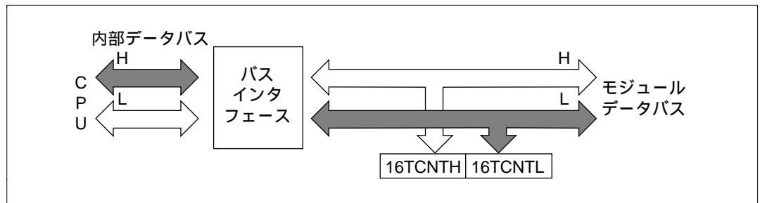
図 9.7 16TCNTLのアクセス動作 [CPU 16TCNTL (下位バイト)]
