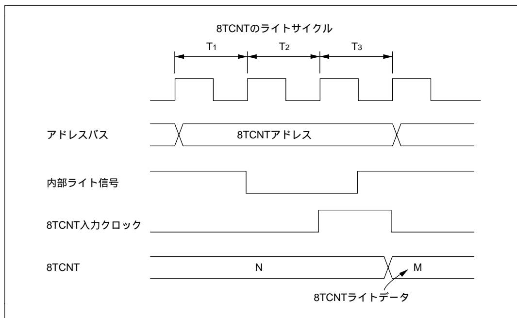
図 10.19 8TCNTのライトとカウントアップの競合
