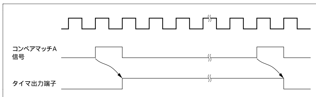
図 10.10 タイマ出力タイミング
