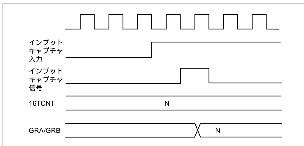
図 9.23 インพุットキャプチャ入力信号タイミング
