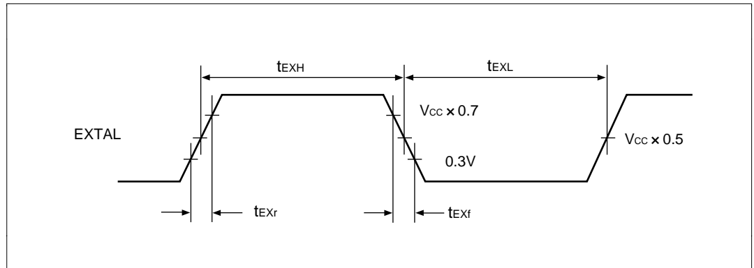
図 19.6 外部クロック入力タイミング
