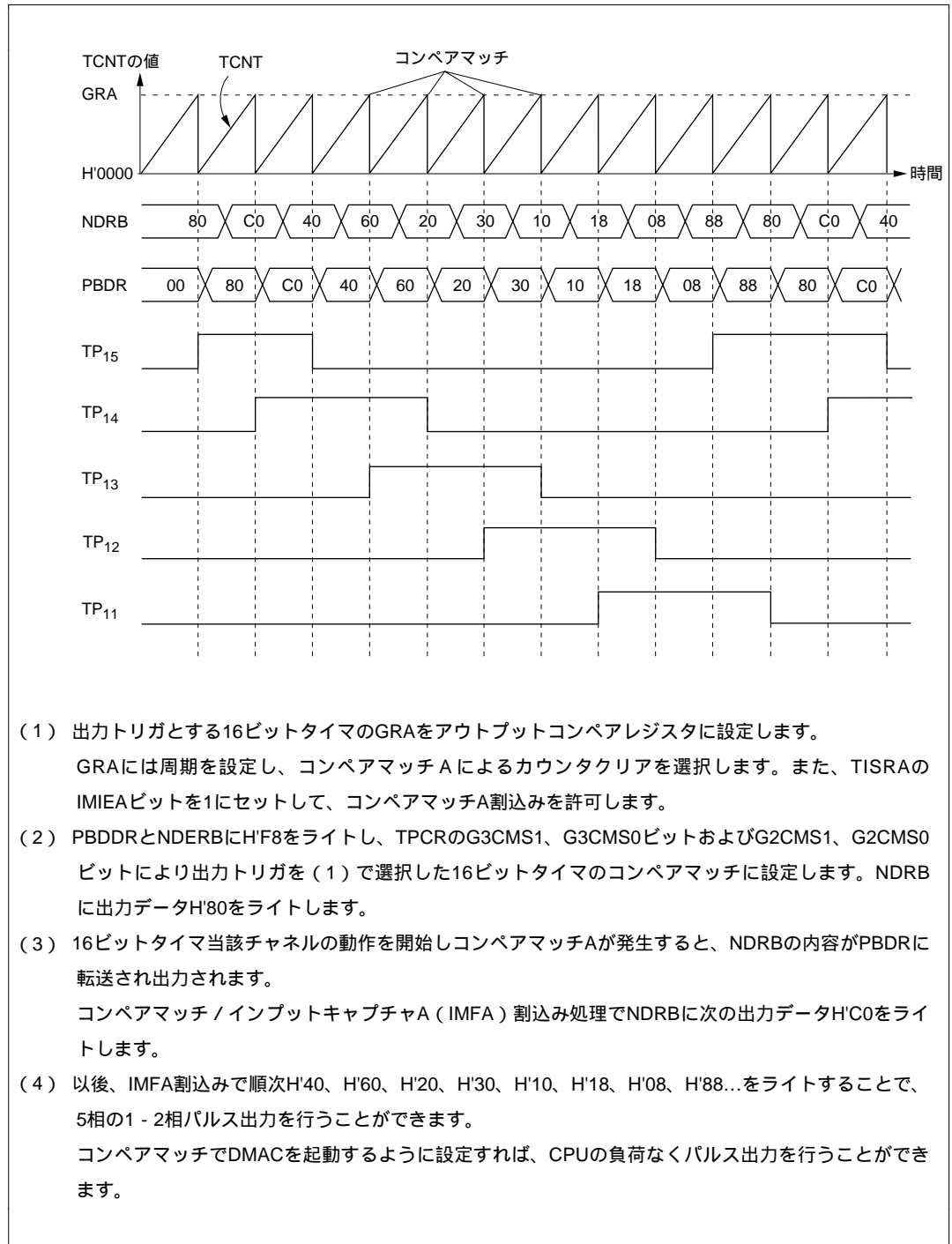
図 11.5 TPC 出力通常動作例 (5 相パルス出力例)
