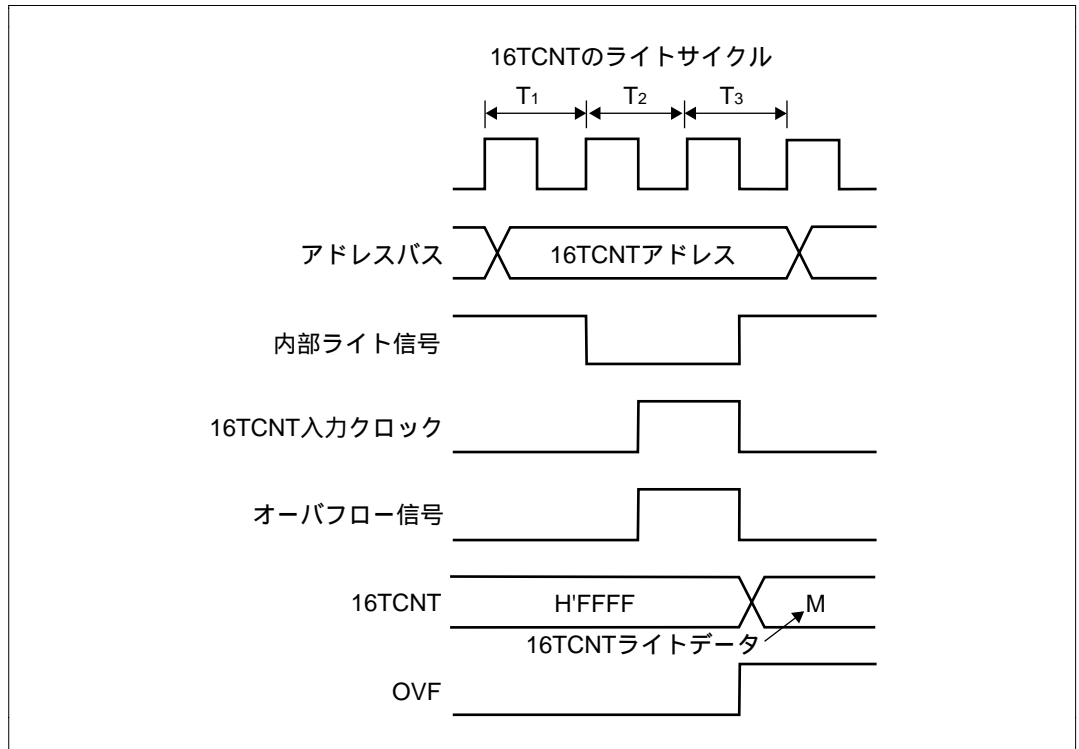
図 9.41 16TCNTのライトとオーバーフローの競合
