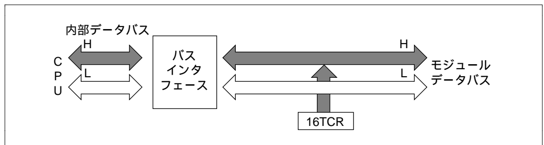
図 9.11 16TCR のアクセス動作 [ 16TCR CPU ]
