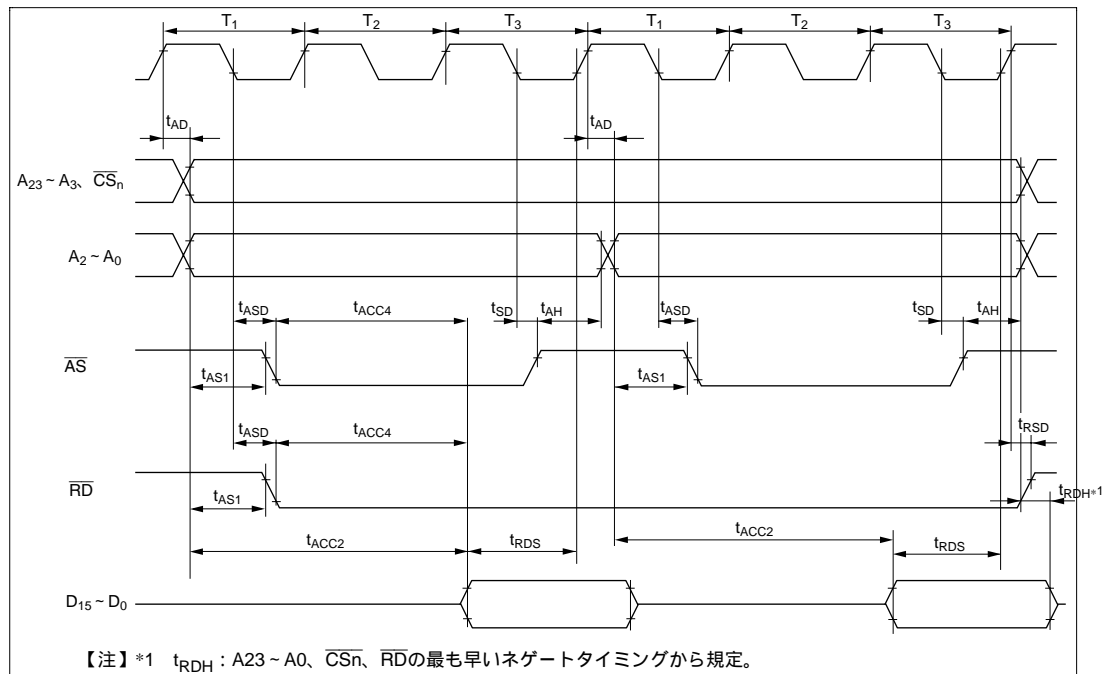
図 21.12 バーストROMアクセスタイミング (バーストサイクル3ステート)
