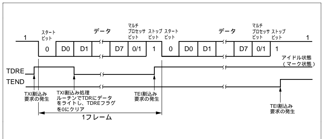
図 13.11 SCIの送信時の動作例 (8ビットデータ/マルチプロセッサビットあり/1ストップビットの例)
