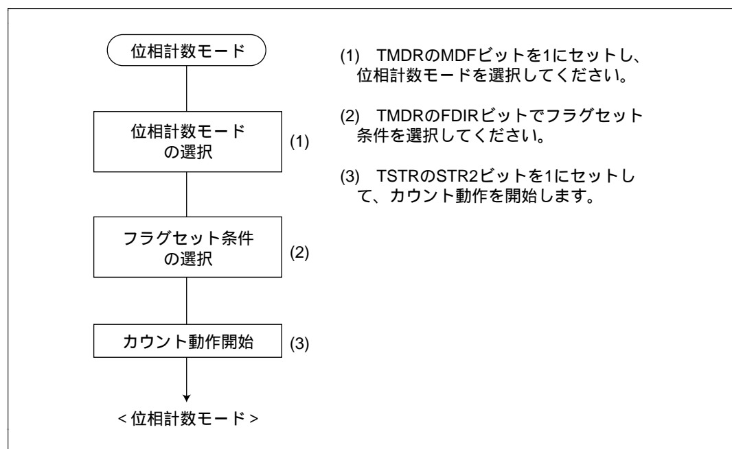
図 9.29 位相計数モードの設定手順例
