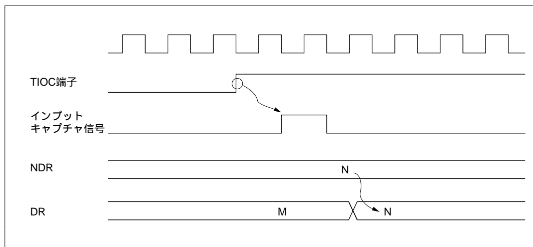
図 11.8 インพุットキャプチャによる TPC 出力例
