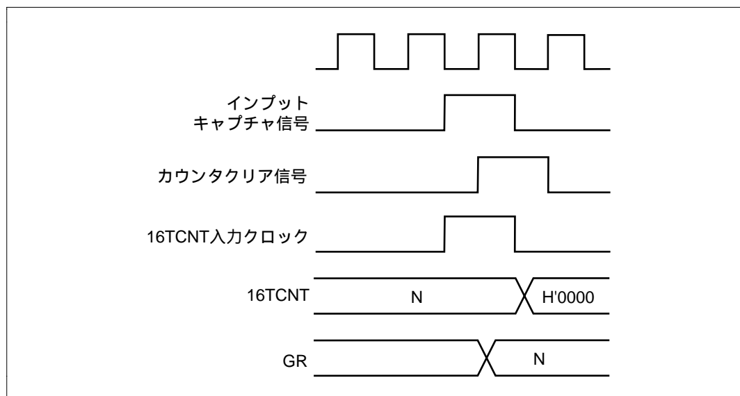
図 9.43 インพุットキャプチャによるカウンタクリアとカウントアップの競合
