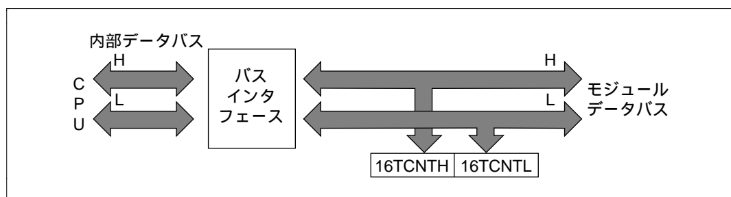
図 9.4 16TCNT のアクセス動作 [ CPU 16TCNT (ワード) ]
