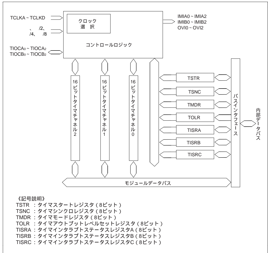
図9.1 16ビットタイマのブロック図(全体図)
