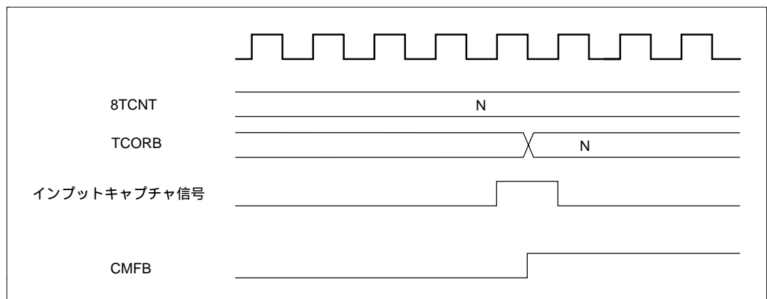
図 10.15 インพุットキャプチャ時の CMFB フラグセットタイミング
