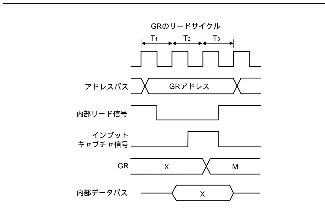
図 9.42 GR のリードとインプットキャプチャの競合
