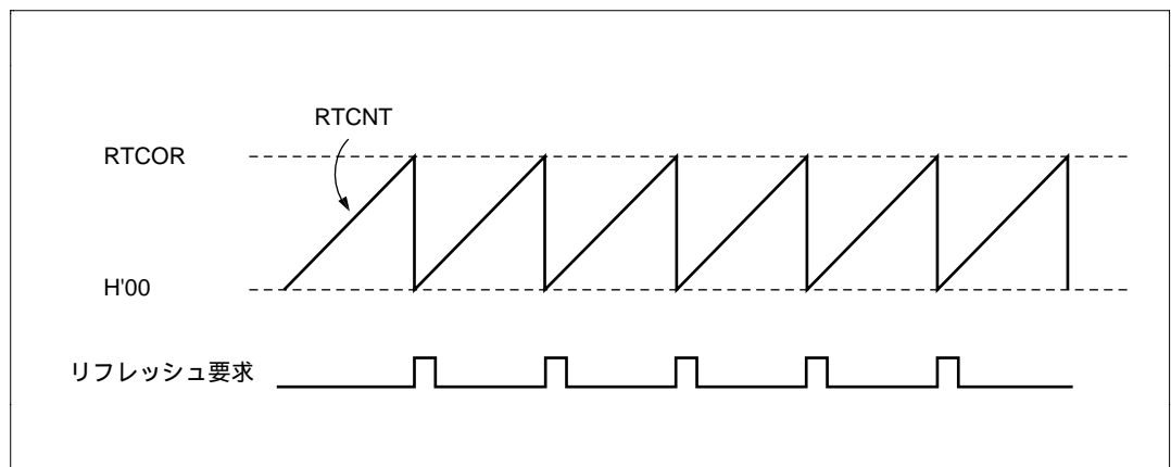
図 6.26 RTCNT の動作
