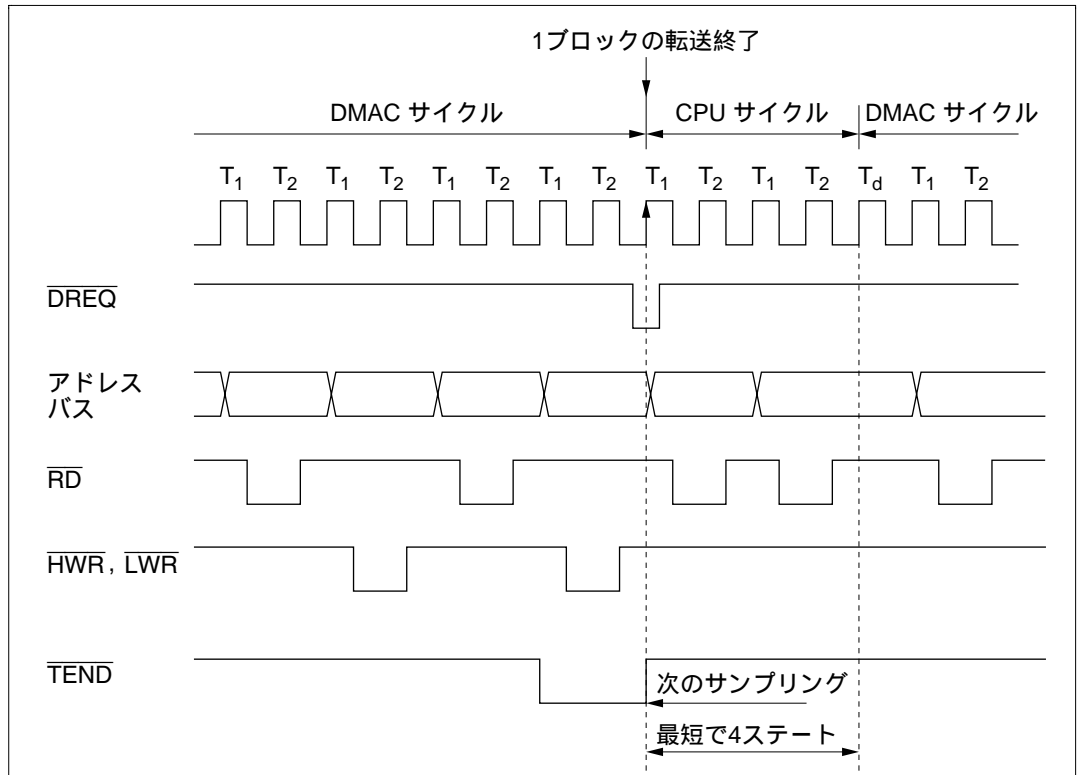
図 7.18 ブロック転送モード時の \overline{\text{DREQ}} 端子の立下がりエッジによる DMAC 起動タイミング
