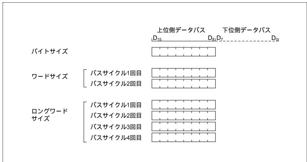
図6.7 アクセスサイズとデータアライメント制御 (8ビットアクセス空間)
