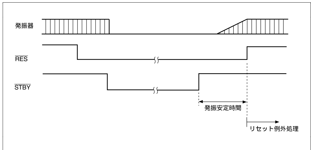
図 20.2 ハードウェアスタンバイモードのタイミング
