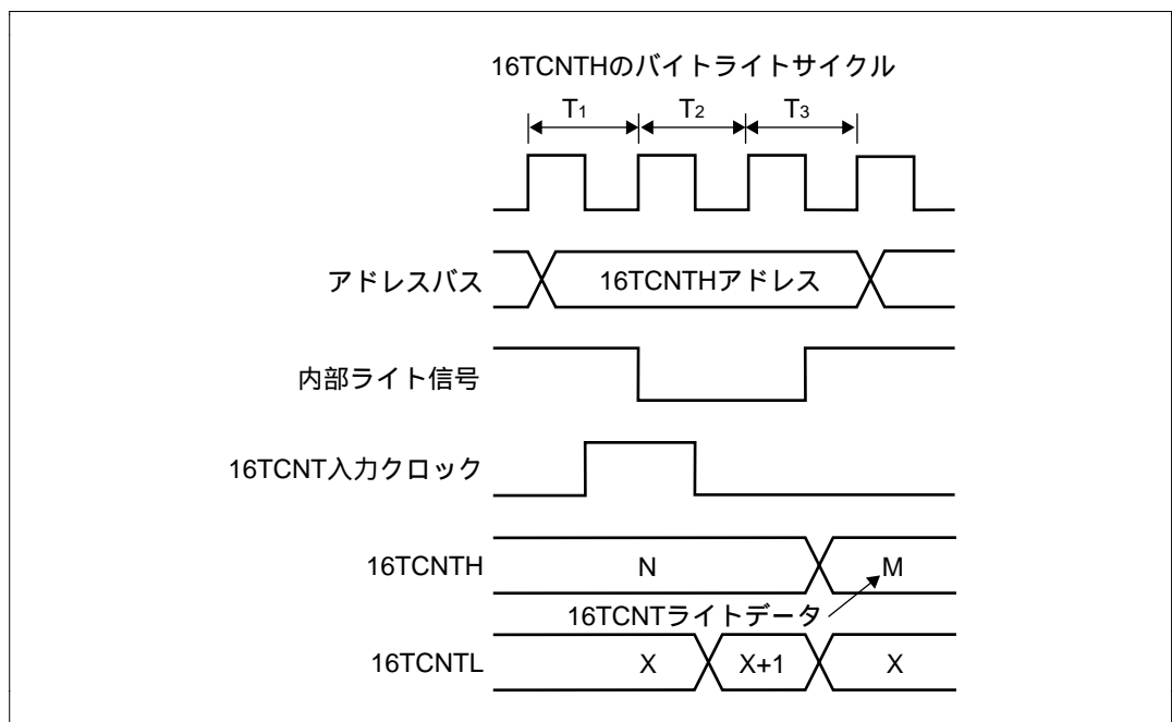
図 9.39 16TCNTのバイトライトとカウントアップの競合
