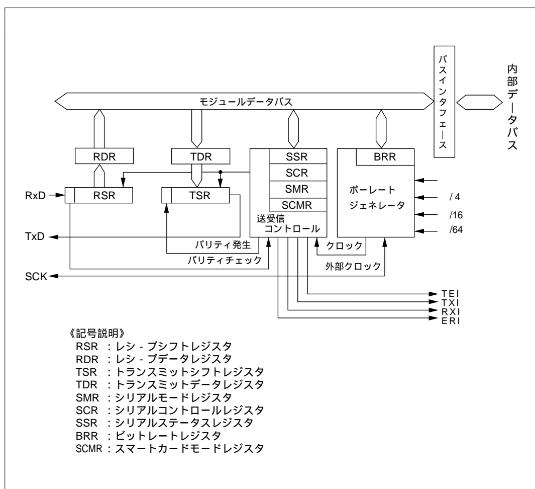
図 13.1 SCI のブロック図
