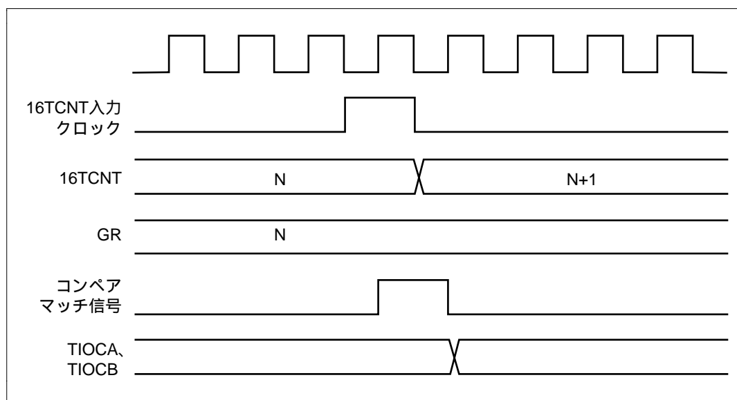
図 9.20 アウトプットコンペア出力タイミング
