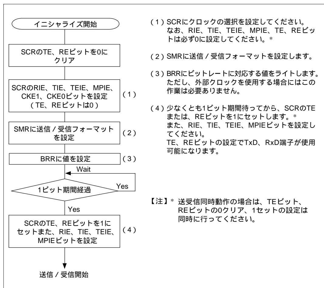
図13.15 SCIのイニシャライズフローチャートの例
