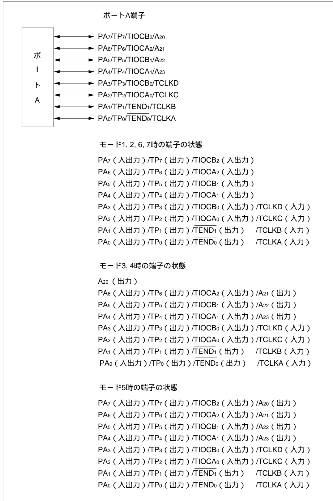
図 8.10 ポート A の端子構成
