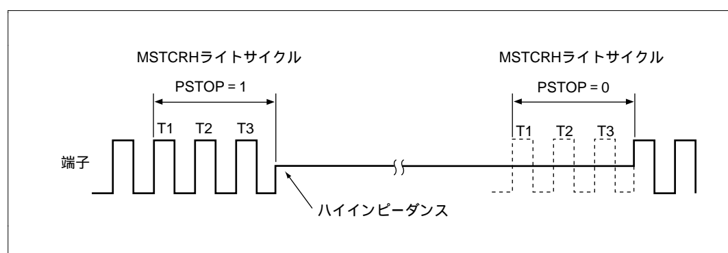
図 20.3 クロック発振開始、発振停止タイミング
