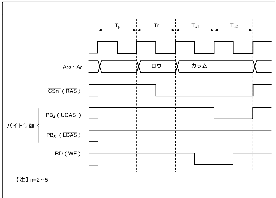
図 6.21 制御タイミング (CSEL=0 の場合の上位バイトライトアクセス時)
