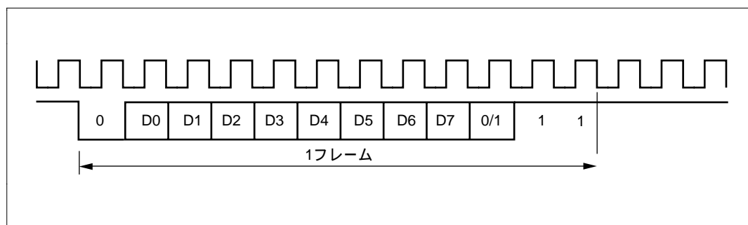
図13.3 出力クロックと通信データの位相関係（調歩同期式モード）
