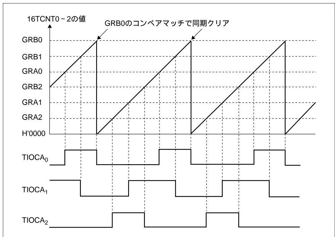
図9.25 同期動作例
