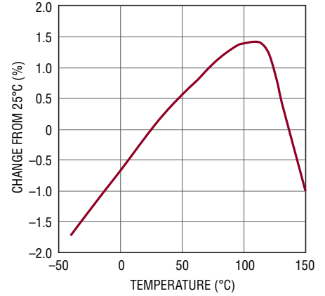
RUNピンのヒステリシス電流と温度
