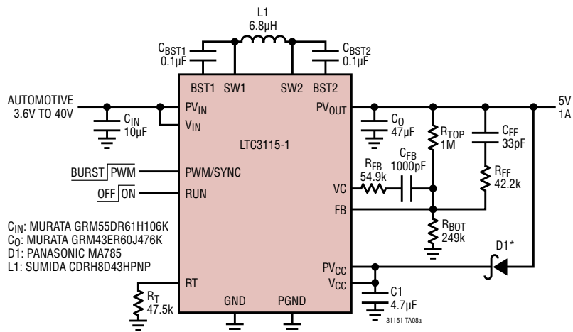
コールドクランクに対応できる自動車用 750kHz、5Vレギュレータ
