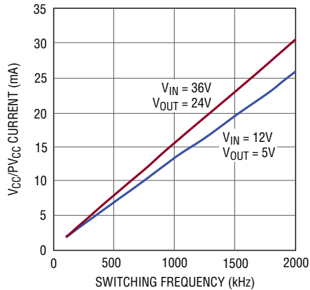
V_{\text{CC}}/\text{PV}_{\text{CC}} 電源電流の合計とスイッチング周波数
