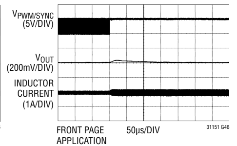
フェーズロック・ループの解除 ( V_{IN} = 24\text{V} , 1.2MHz クロック)
