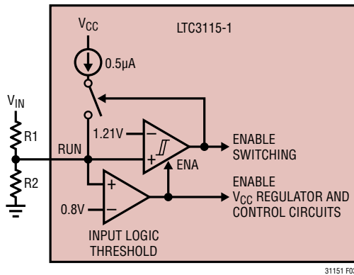
図3.RUNピンの高精度コンパレータ
