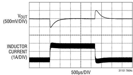
0Aから1.5Aの負荷ステップ ( V_{IN} = 24V )
