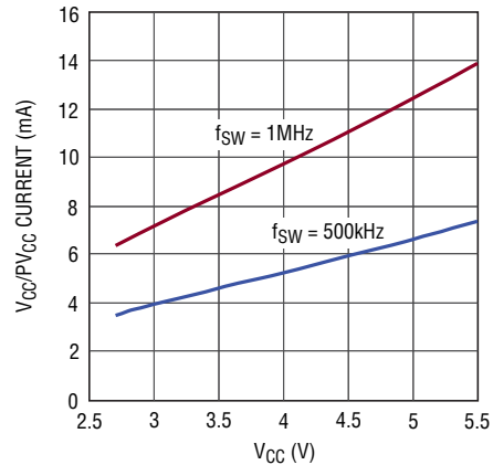
V_{\text{CC}}/\text{PV}_{\text{CC}} 電源電流の合計と V_{\text{CC}}
