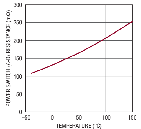
パワースイッチの抵抗と温度
