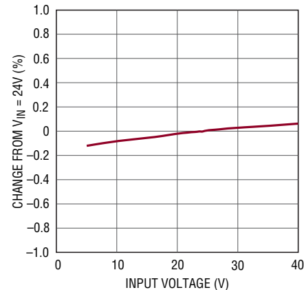
V_{\text{CC}} レギュレータの入力レギュレーション
