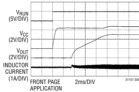
ソフトスタートの波形
