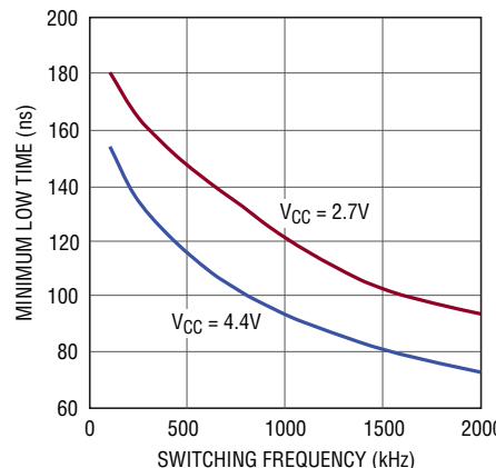
SW1、SW2の最小“L”時間とスイッチング周波数
