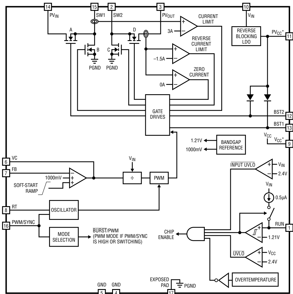
ブロック図 ピン番号はDHDパッケージのみを示す。
