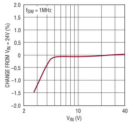
発振器周波数とV IN
