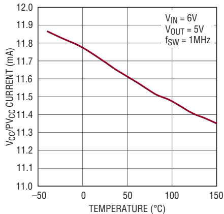
V_{\text{CC}}/\text{PV}_{\text{CC}} 電源電流の合計と温度
