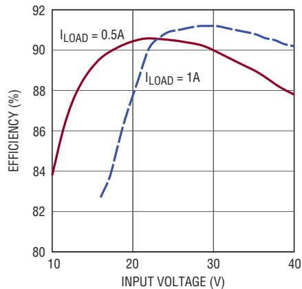
効率とVIN
