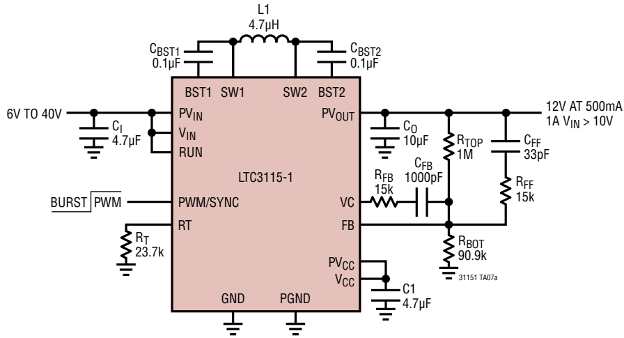
小型サイズの1.5MHz、12V電源
