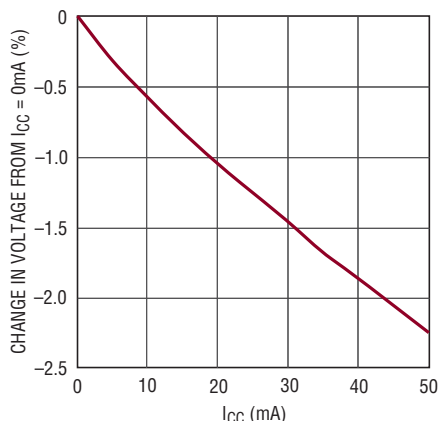
V_{\text{CC}} レギュレータの負荷レギュレーション
