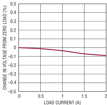
V_{\text{CC}} レギュレータの負荷レギュレーション
