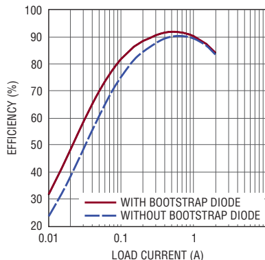
効率と負荷電流 VIN = 12V
