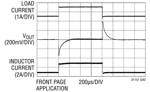
負荷トランジェント (0Aから1A) ( V_{IN} = 3.6\text{V} , V_{OUT} = 5\text{V} )
