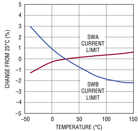
インダクタ電流制限しきい値と温度
