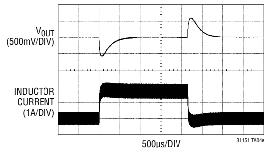
0Aから1.5Aの負荷ステップ ( V_{IN} = 40V )
