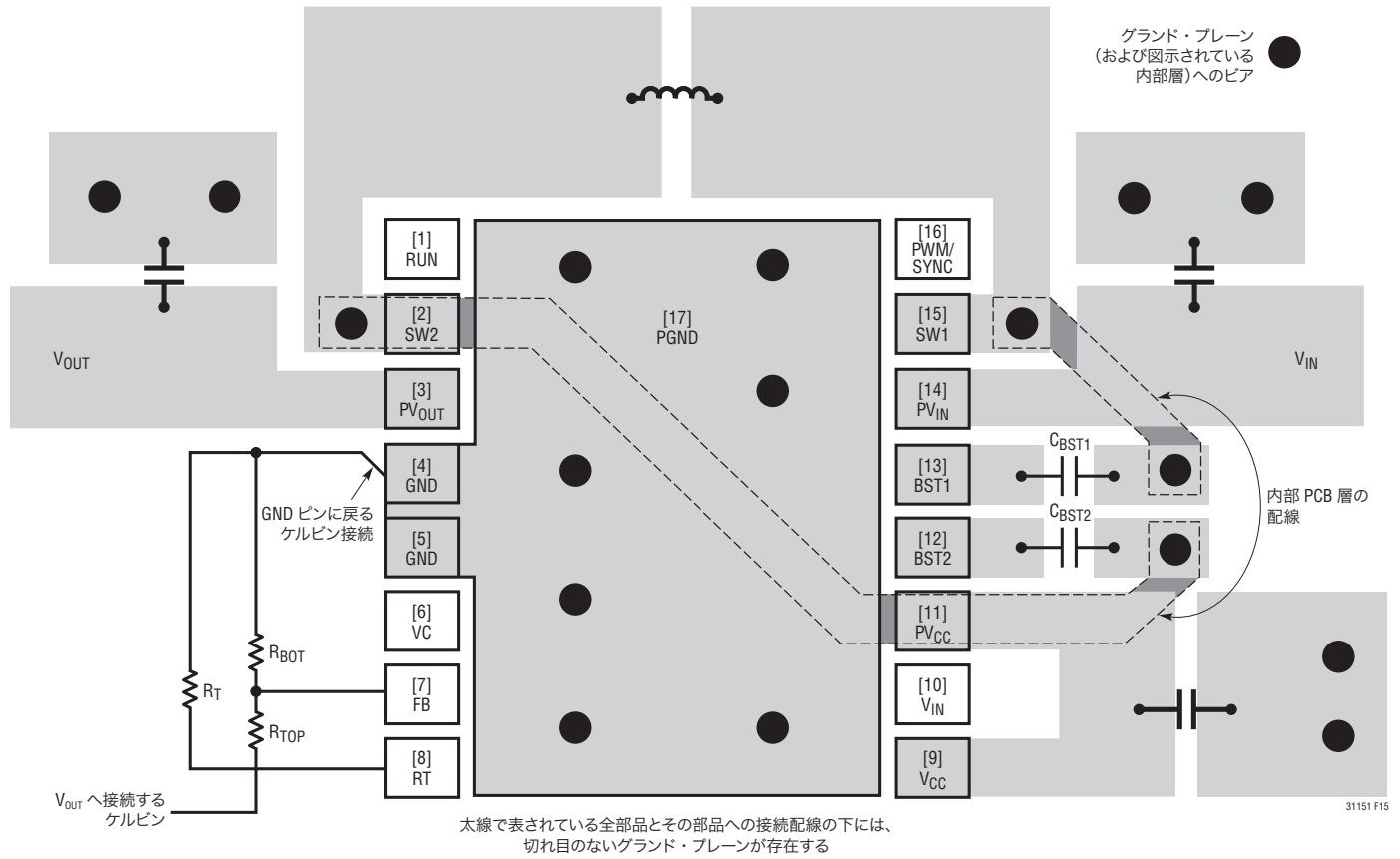
図 15.DHD パッケージの推奨 PCB レイアウト
