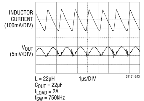
PWM モードの出力電圧リップル ( V_{IN} = 24\text{V} , V_{OUT} = 5\text{V} )
