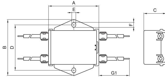
RSEL-20R5/2001/2002/2003/2006W(L)
