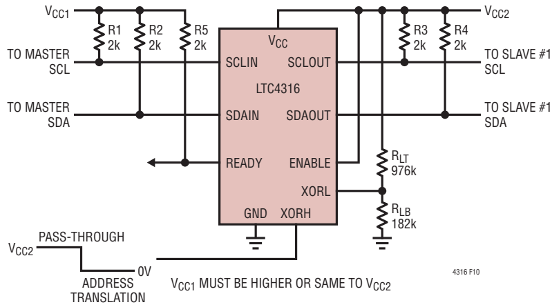
図 10. パススルー・モード向けオプションを備えたアプリケーション
