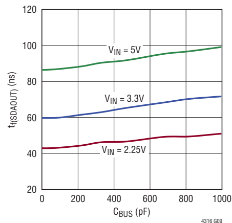
SDAOUTの立ち下がり時間とバス容量
