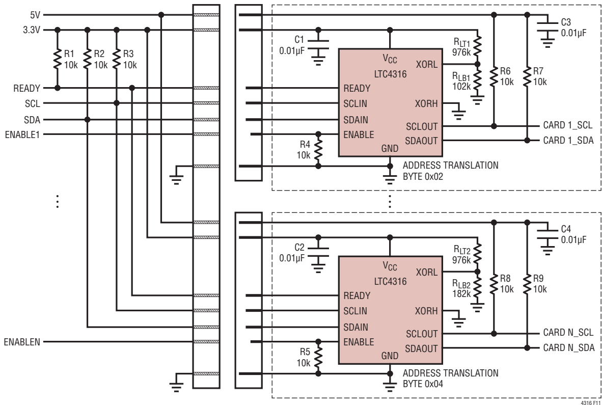
図 11. 時差接触コネクタを使用した I 2 C 活線挿抜アプリケーションでの LTC4316
