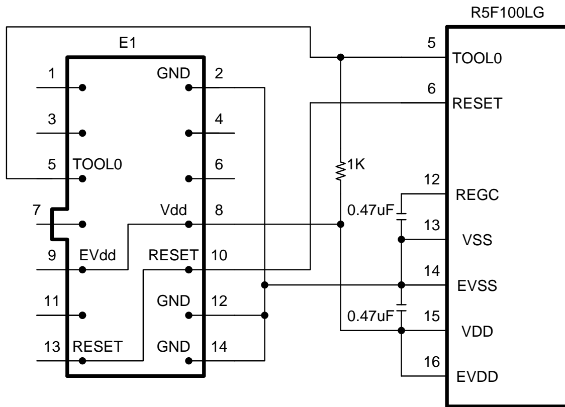
E 1 接続書き込み回路例
