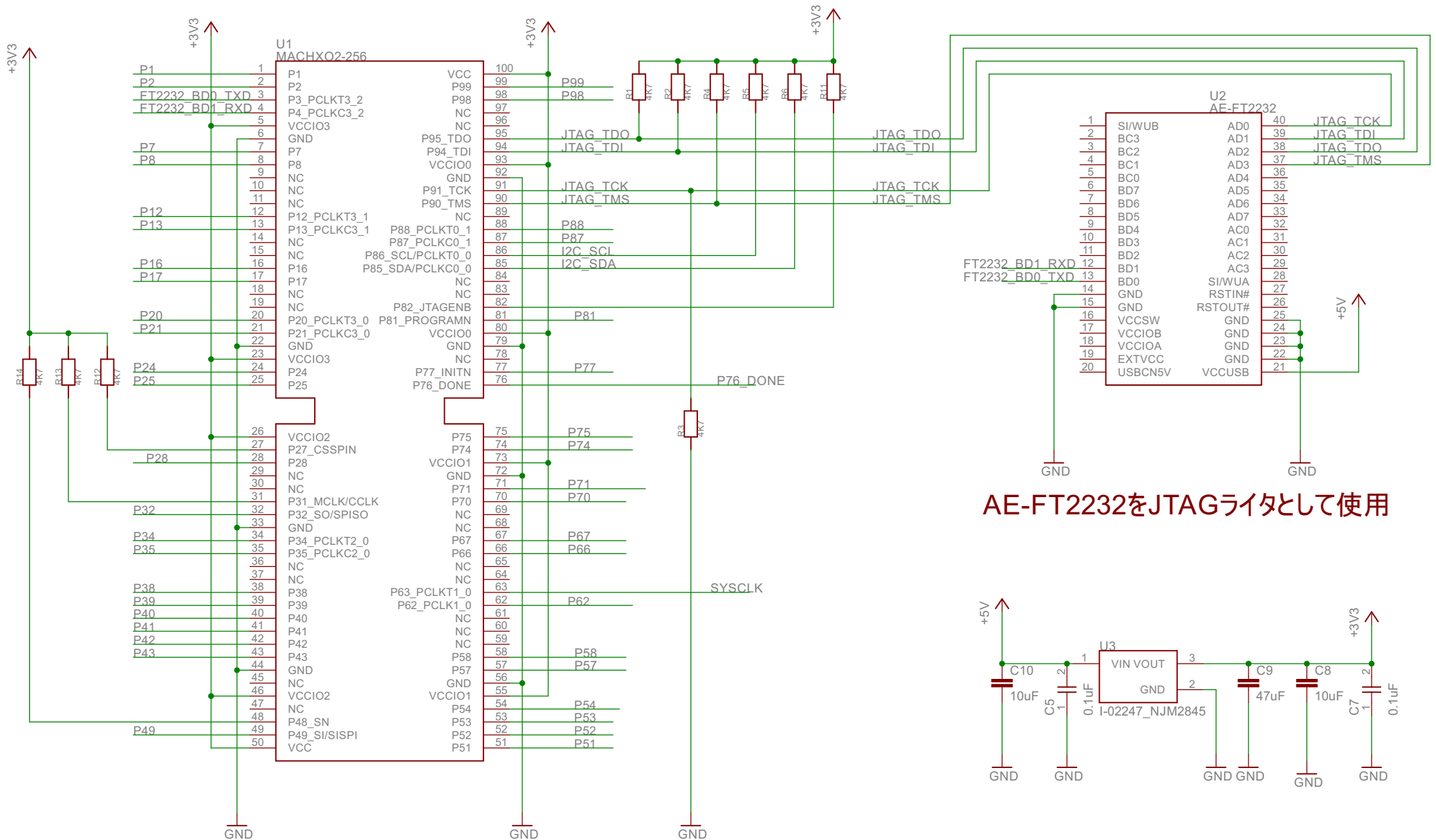
MachXO2のコンフィグ回路及びJTAG回路
