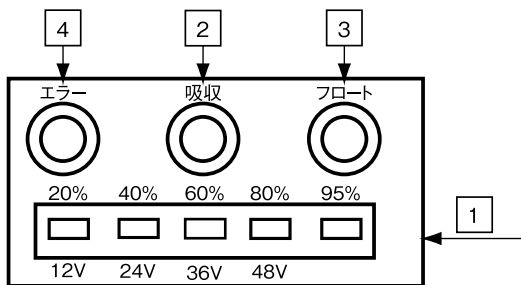
図 1-3 本体パネル
