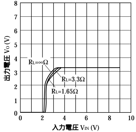
図 12 出力電圧 - 入力電圧特性 (PQ3RD23)
