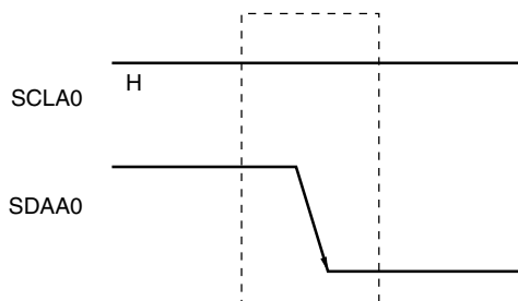
図13-14 スタート・コンディション
