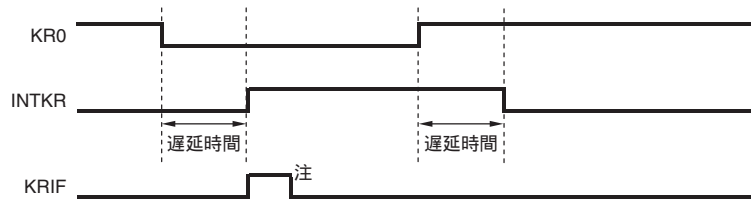
図15-5 1つのチャンネルへのキー割り込み入力時のINTKR信号の動作 (KRMD = 0, KREG = 0設定時)
