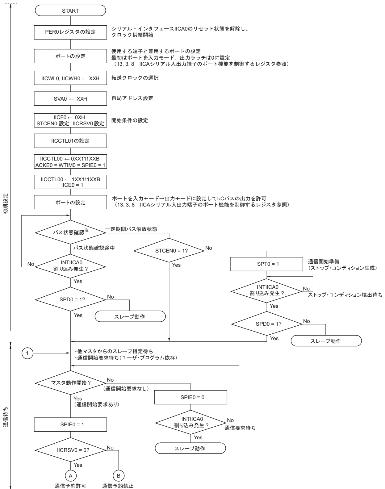
図13-29 スレープ動作手順 (1)
