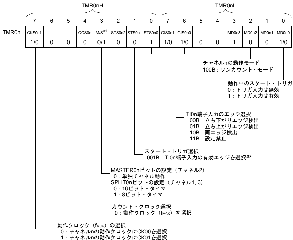
図6-62 デレイ・カウンタのレジスタ設定内容例
