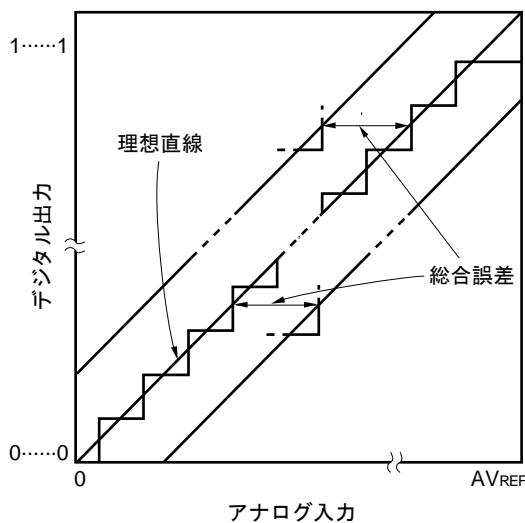
図10-17 総合誤差
