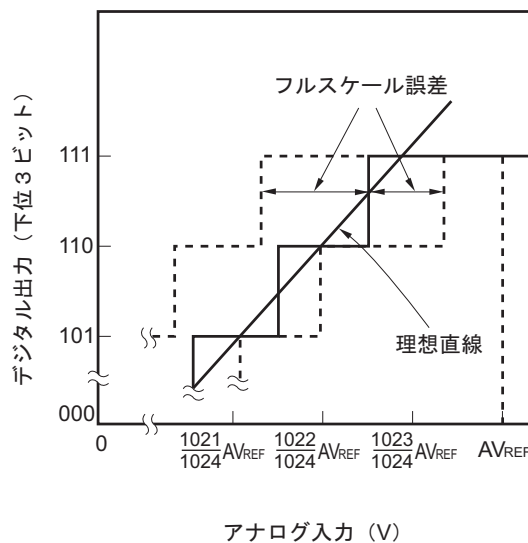
図10-20 フルスケール誤差
