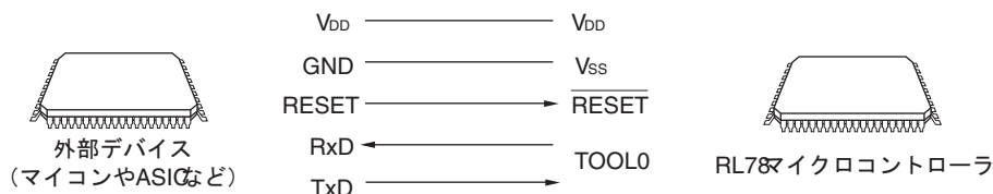
図20-4 外部デバイスとの通信
