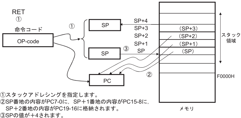
図3-36 RETの例
