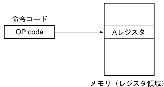
図3-16 インプライド・アドレッシングの概略
