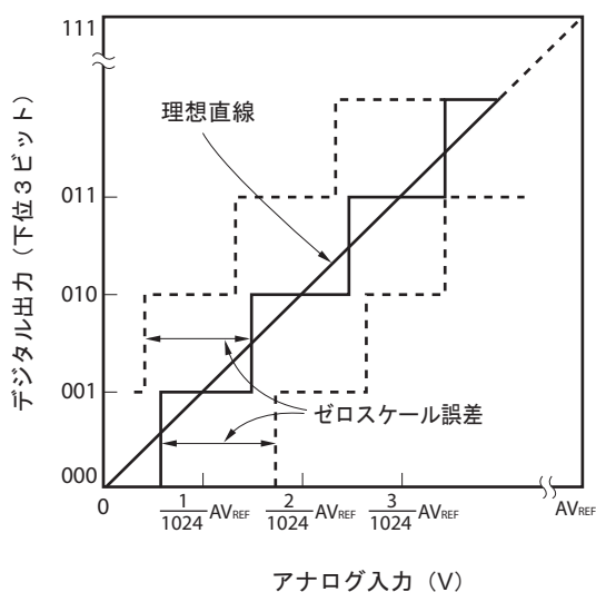
図10-19 ゼロスケール誤差
