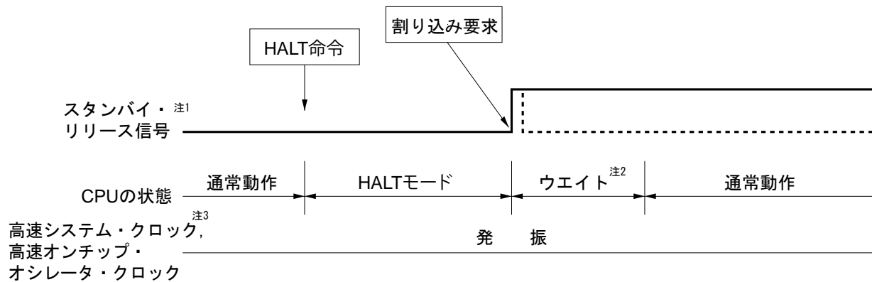
図16-1 割り込み要求発生によるHALTモードの解除
