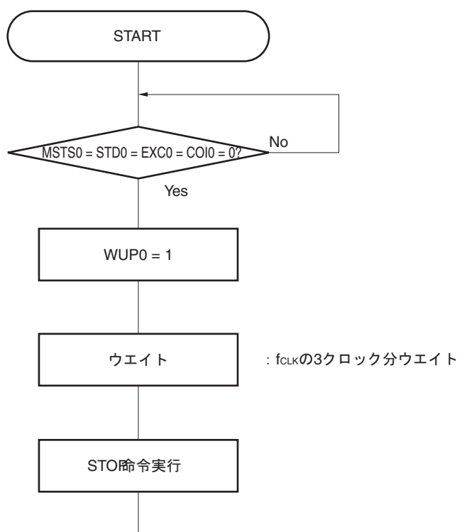
図13-21 WUP0 = 1を設定する場合のフロー
