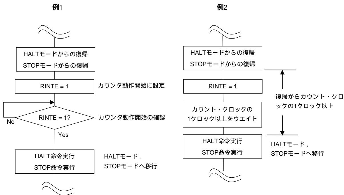
図7-6 RINTE = 1に設定後のHALTモード、STOPモードへの移行手順
