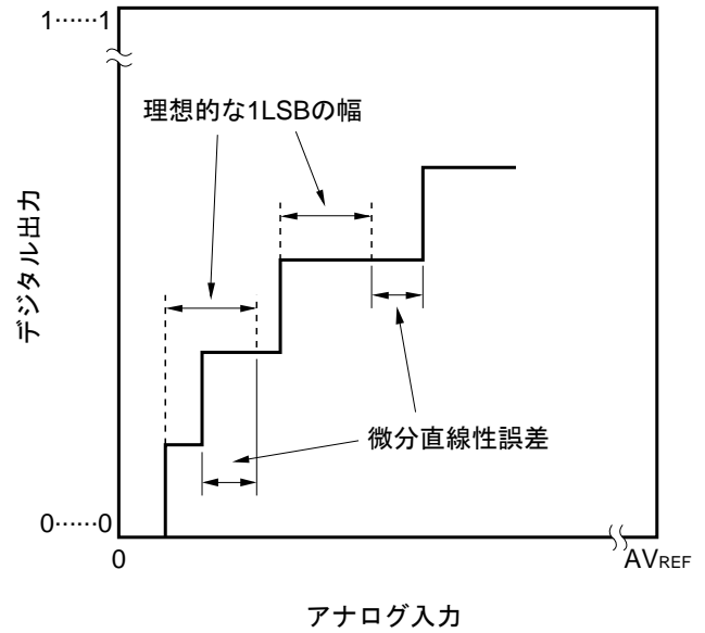
図10-22 微分直線性誤差
