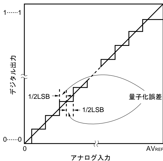
図10-18 量子化誤差
