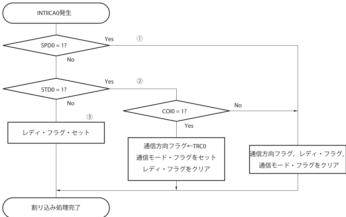
図13-30 スレーブ動作手順（2）
