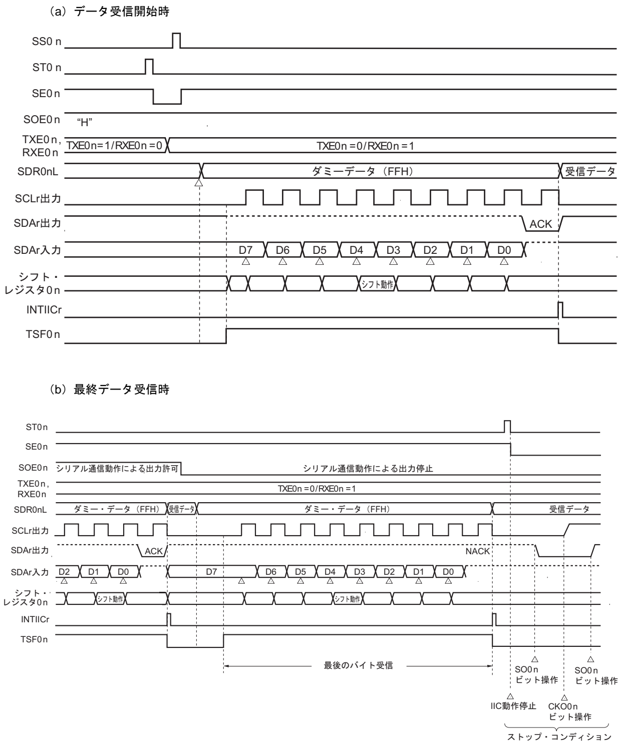
図12-94 データ受信のタイミング・チャート
