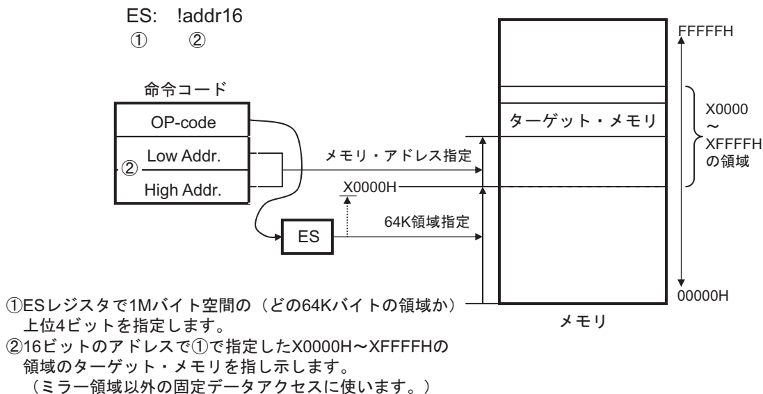
図3-19 ES:!addr16の例
