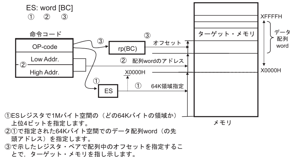
図3-30 ES:word[BC]の例
