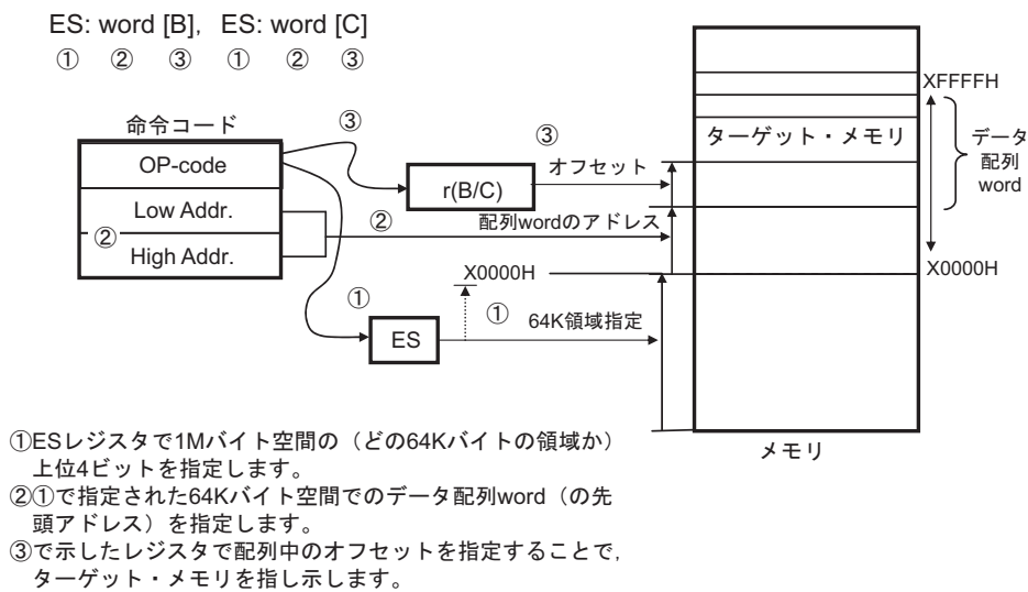
図3-30 ES:word[BC]の例
