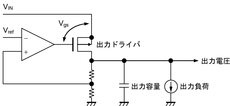
図13 回路図
