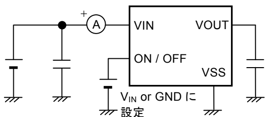
図6 測定回路2
