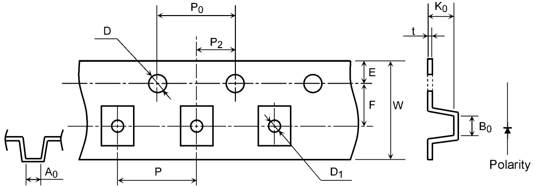
Fig. 12.3.1 Tape Dimensions
