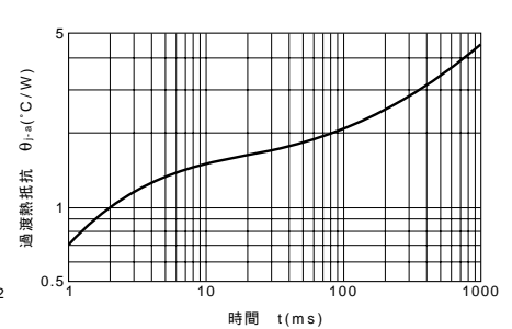
θj-a-t特性
