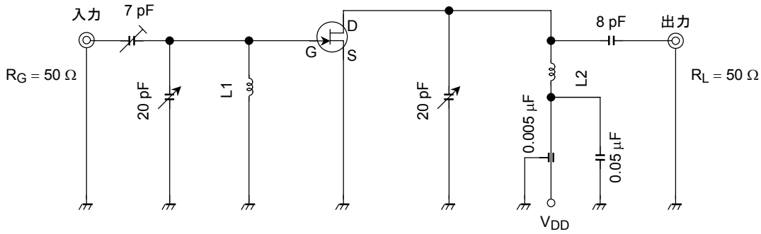
L1: \phi 0.8 mm 銀メッキ線空心 3T, 捲径 \phi 10 mm, 捲長 10 mm L2: \phi 0.8 mm 銀メッキ線空心 3.5T, 捲径 \phi 10 mm, 捲長 10 mm
