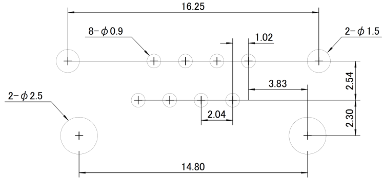
C-00159 7810-8P8C (unit : mm)
