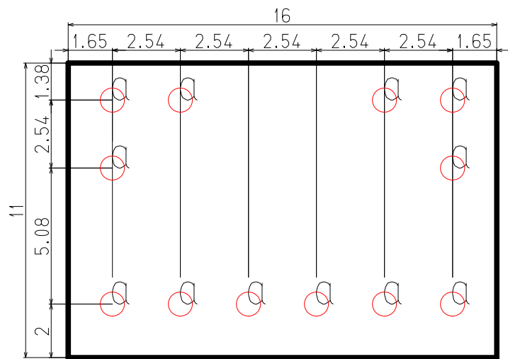
穴加工図
