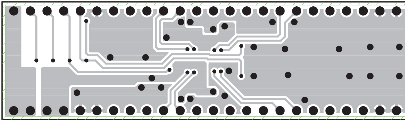
BOT (半田面パターン)
