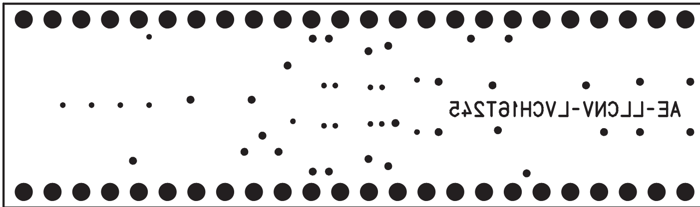
半田面レジスト
