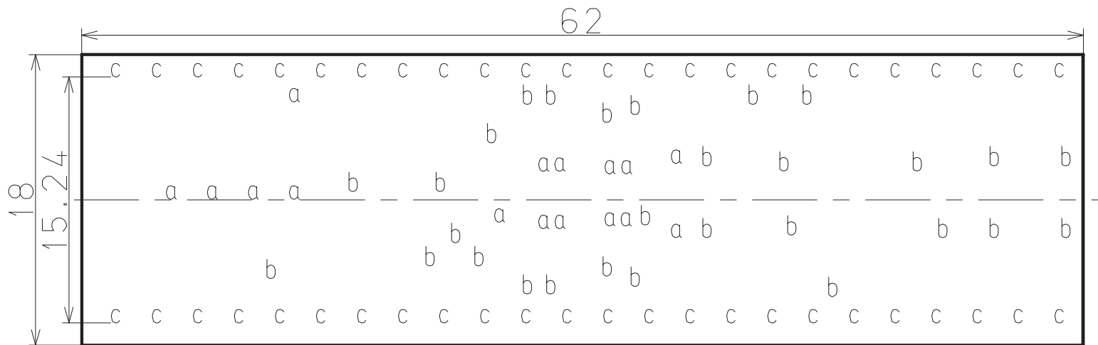
穴加工図
