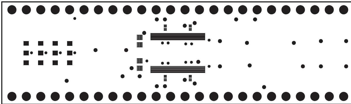
部品面レジスト
