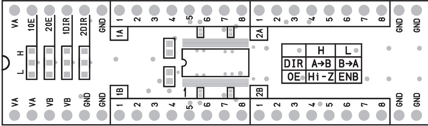
部品面シルク 部品面レジスト
