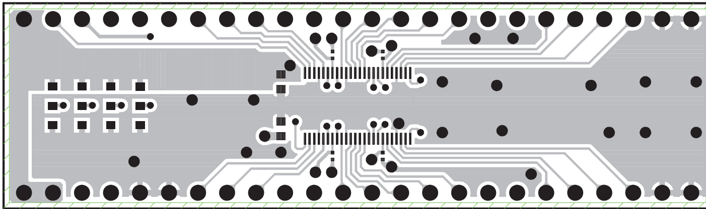
TOP (部品面パターン)
