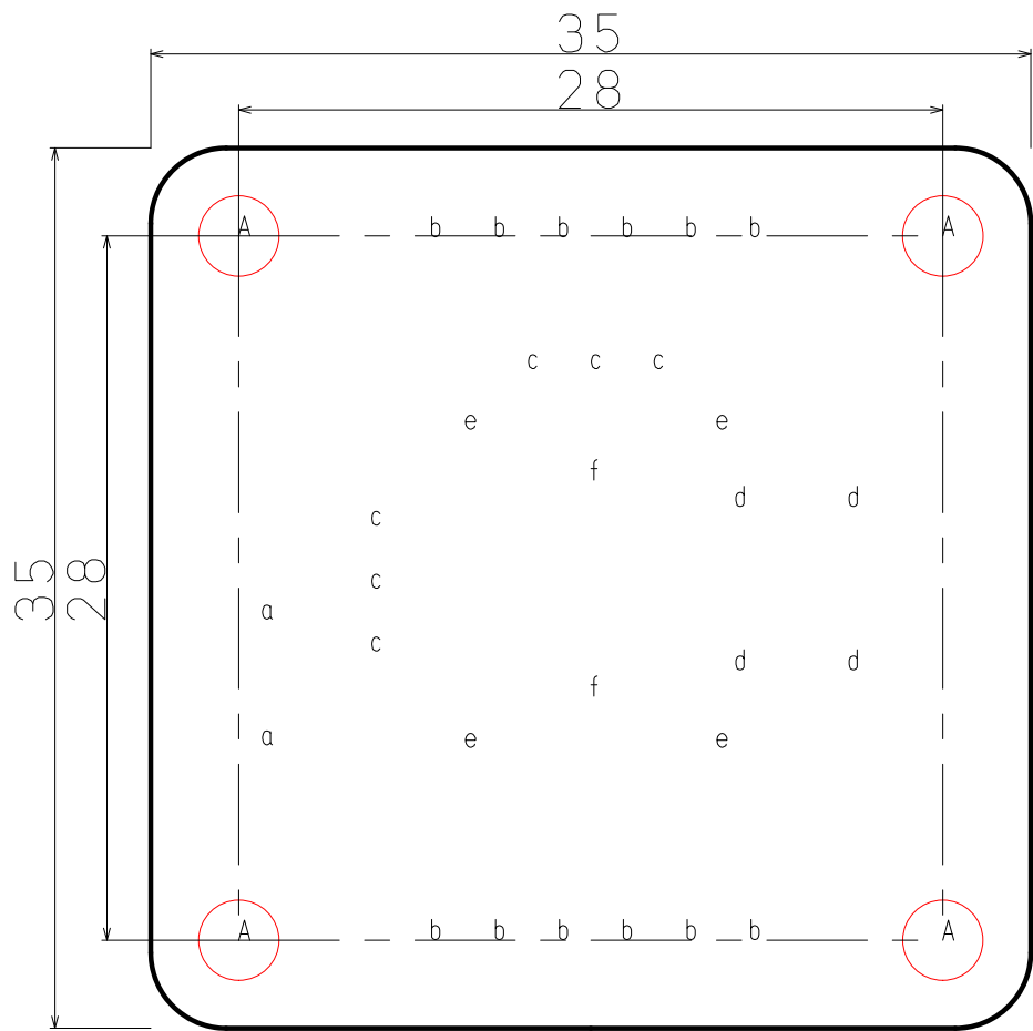
穴加工図
