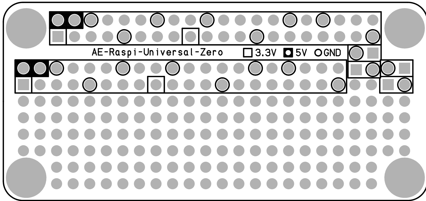
部品面シルク 部品面レジスト
