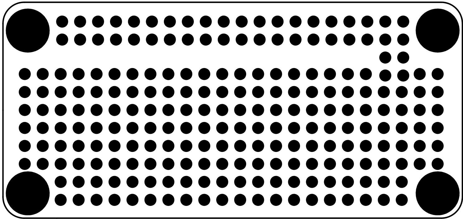
半田面レジスト
