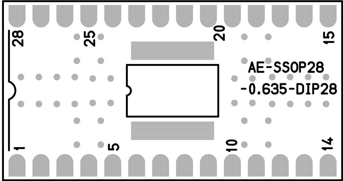
部品面シルク 部品面レジスト
