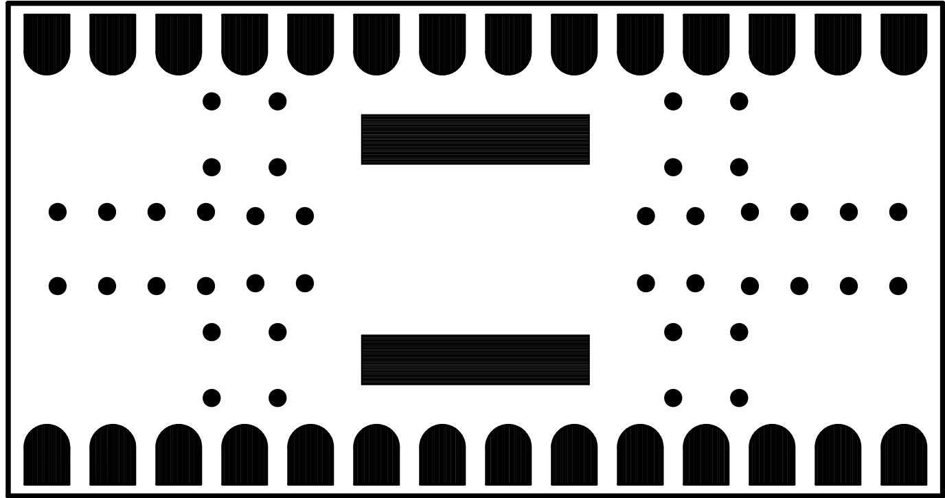
部品面レジスト
