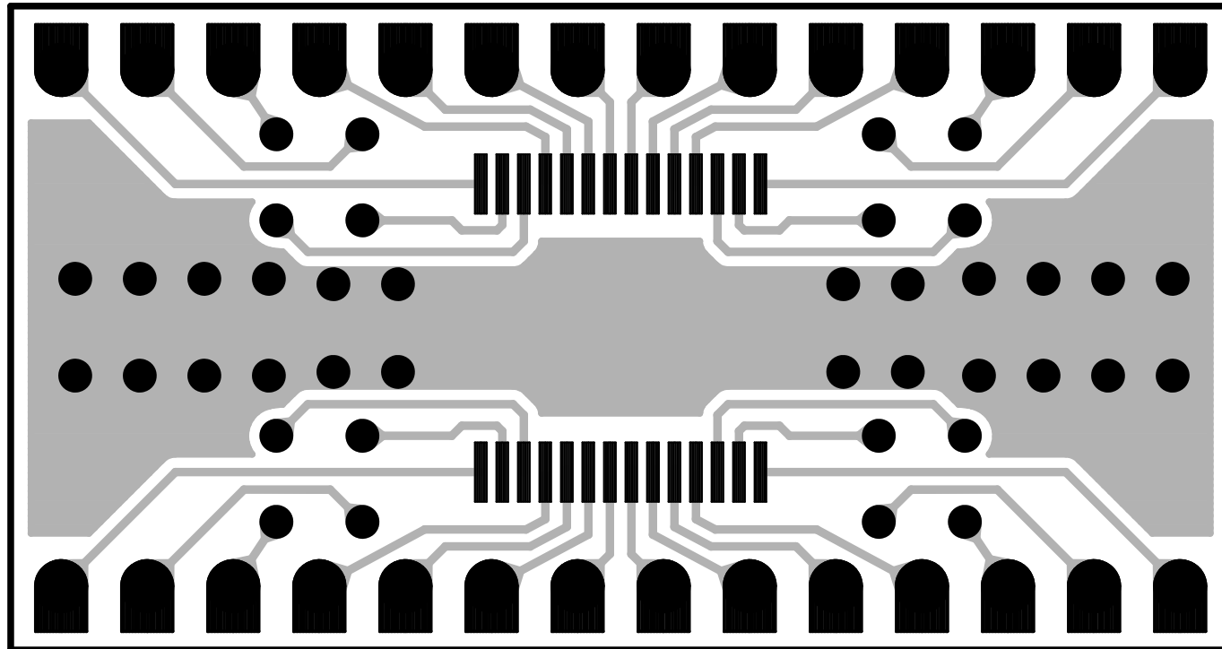
TOP (部品面パターン)
