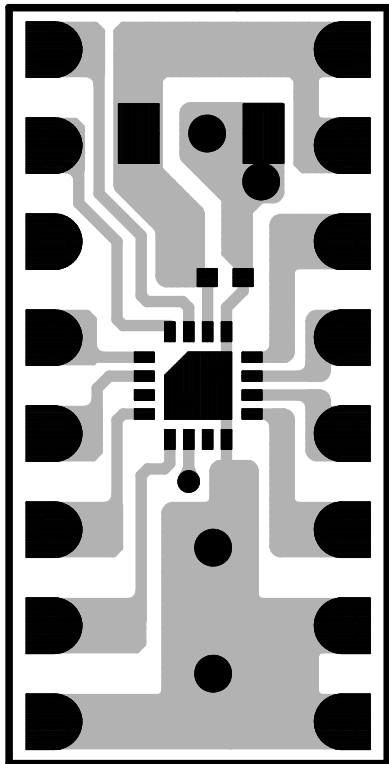
TOP (部品面パターン)
