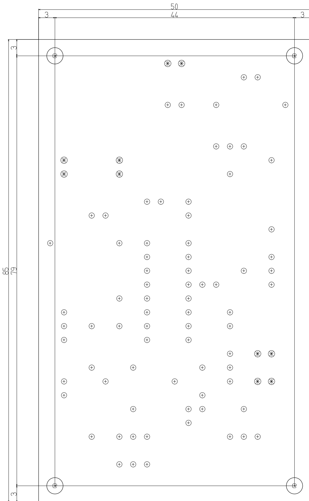
AE-XR2206 基板外形图
