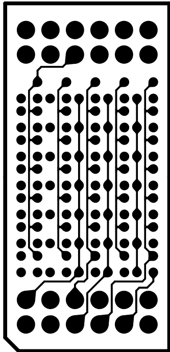
L 2 (内層パターン)
