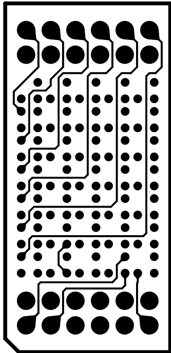
BOT (半田面パターン)
