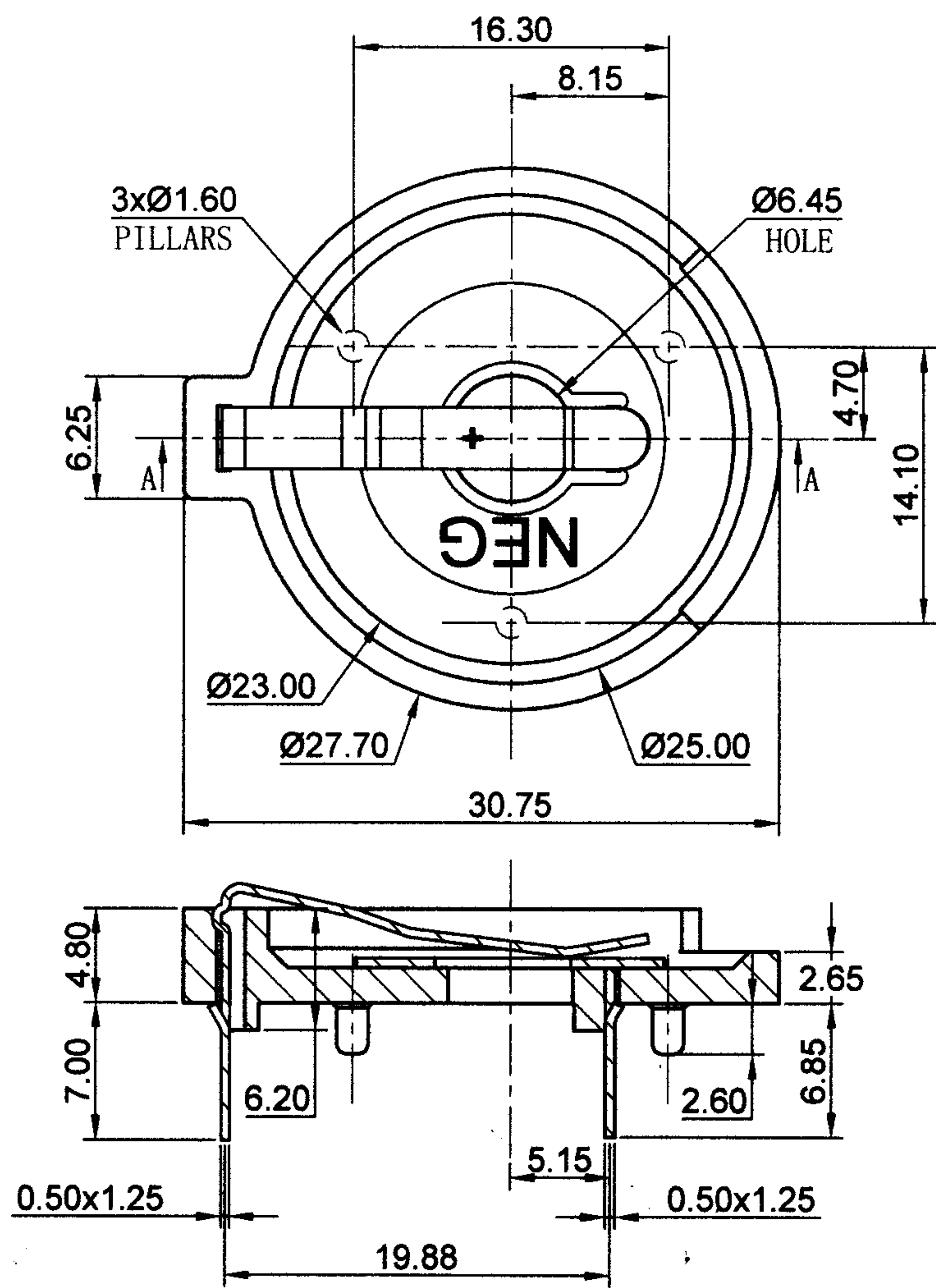
SECTION A-A
