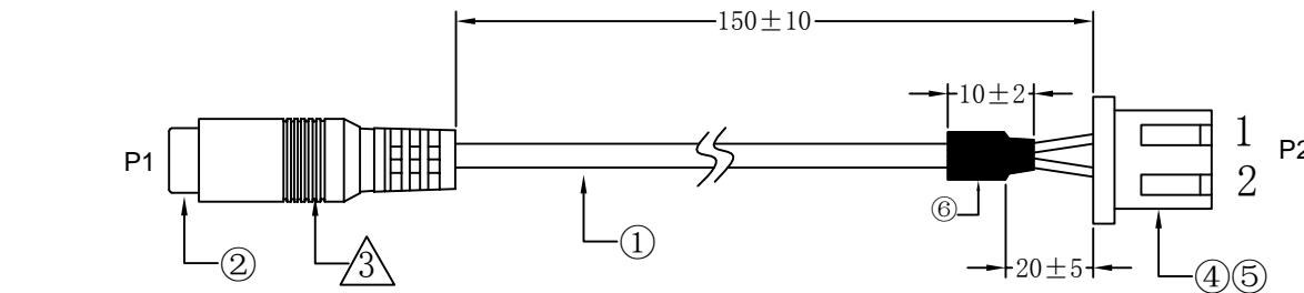
接线图: Wiring Diagram
