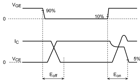
図 6.2.3 スwitching損失のタイミングチャート
