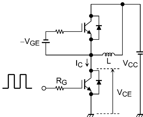
図 6.2.1 スwitching時間の測定回路
