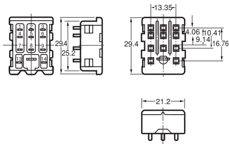
外形寸法図
