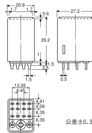
外形寸法図
