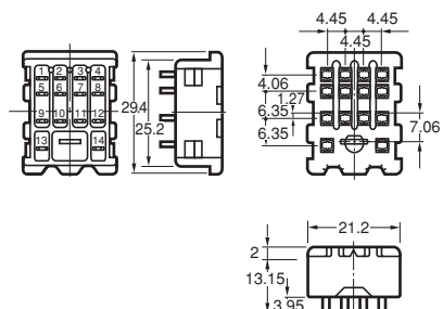
外形寸法図
