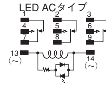
端子配列・内部結線図(BOTTOM VIEW)
