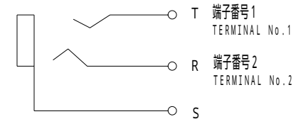
回路図 CIRCUIT
