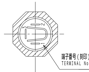
A-A' 断面 A-A' Sect
