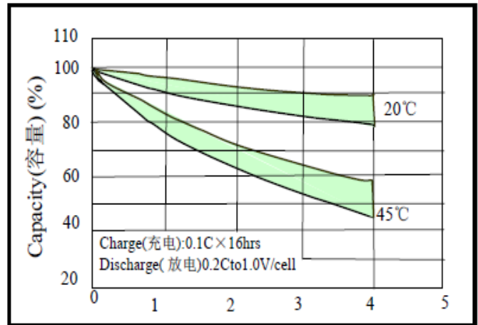
Storage & self discharge Curves 不同温度荷电保持曲线图
