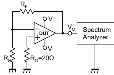
図9 入力換算雑音電圧
