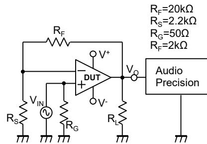
図11 全高調波歪率
