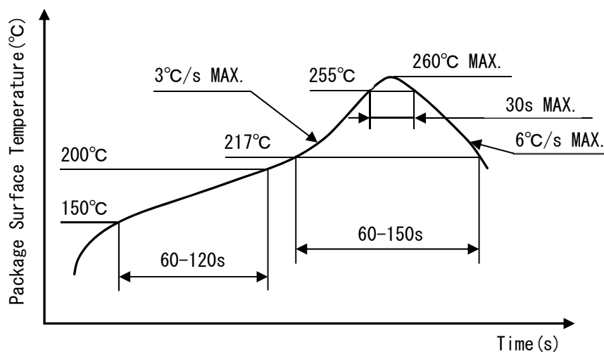
リフロープロファイル
