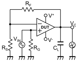
図8 利得帯域幅積、位相余裕
