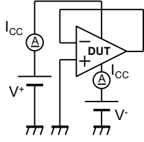
図1 消費電流
