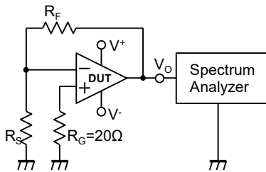
図10 スルーレート
