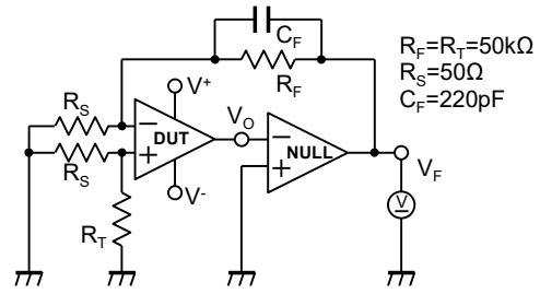
図2 入力オフセット電圧、電源電圧除去比
