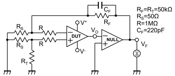
図4 入力オフセット電流
