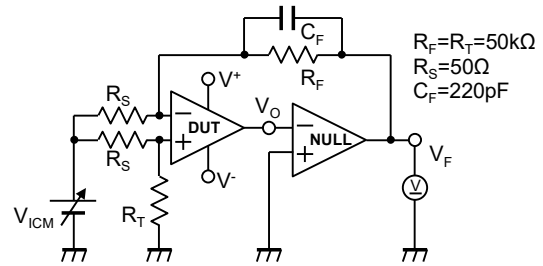
図6 同相信号除去比
