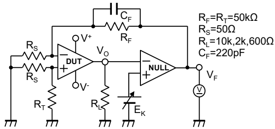
図5 電圧利得
