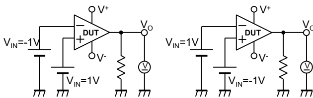
図7 最大出力電圧
