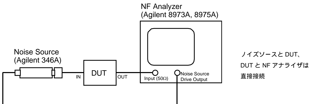
NF 測定
