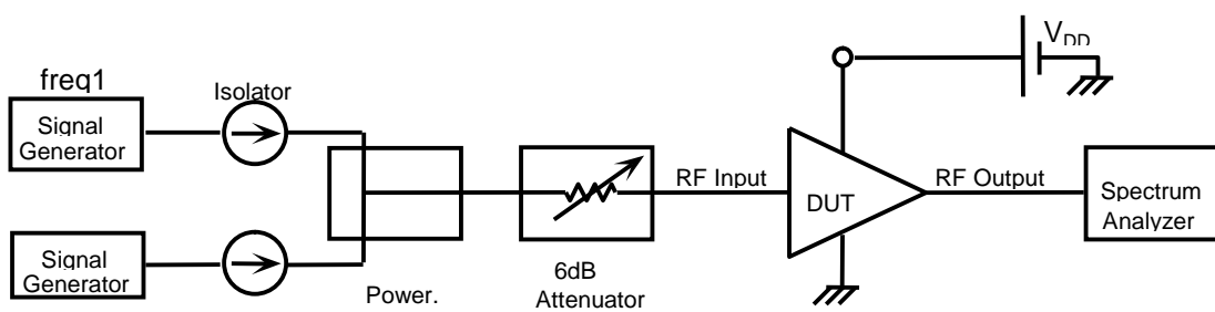
大信号特性測定ブロック
