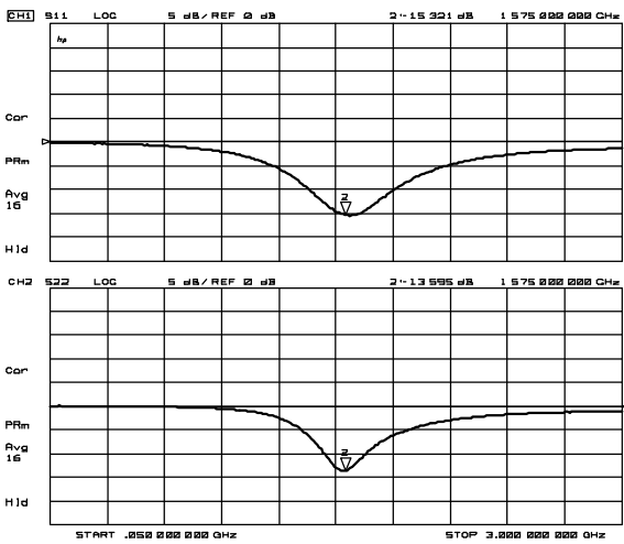
VSWR
