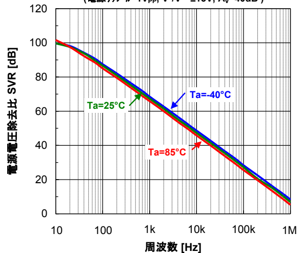
電源電圧除去比(負電源側) - 周波数 (電源リップル \Delta = 1V_{PP} , V^+/V^- = \pm 15V , A_V = 40dB )
