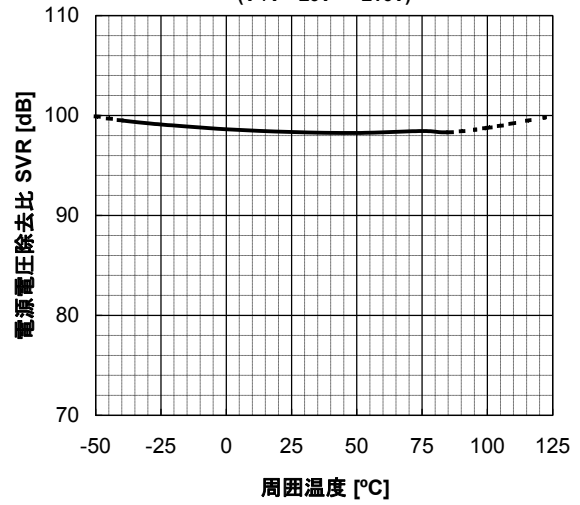
電源電圧除去比 - 周囲温度 ( V^+/V^- = \pm 6V \rightarrow \pm 16V )
