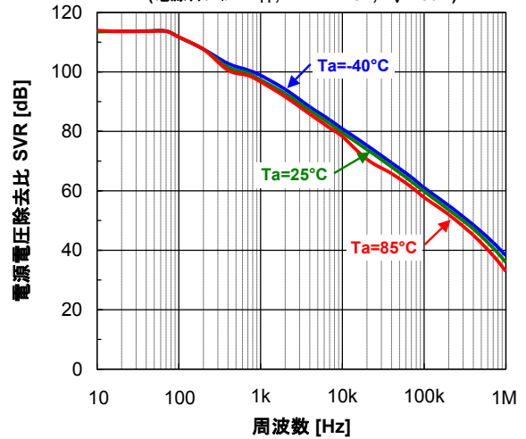
電源電圧除去比(正電源側) - 周波数 (電源リップル \Delta = 1V_{PP} , V^+/V^- = \pm 15V , A_V = 40dB )
