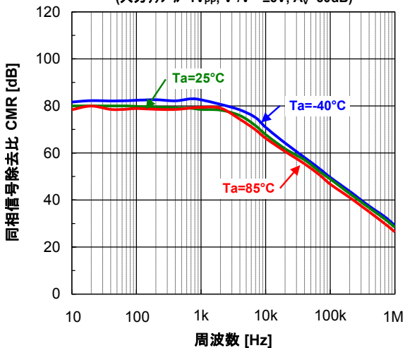
同相信号除去比 - 周波数 (入力リップル \Delta = 1V_{PP} , V^+/V^- = \pm 6V , A_V = 60dB )
