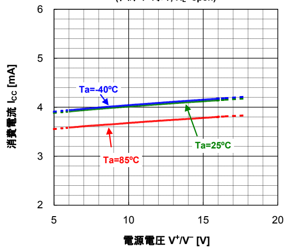
消費電流 – 電源電圧 (負荷レジスタ開放, R_L = open )
