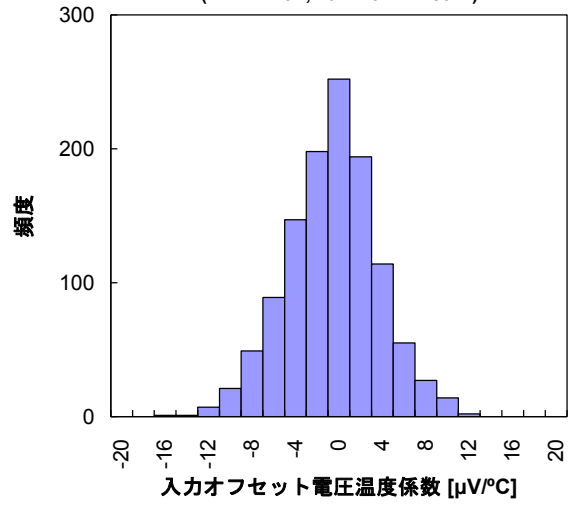
入力オフセット電圧温度係数分布 ( V^+/V^- = \pm 15V , T_a = +25^\circ C \rightarrow +85^\circ C )
