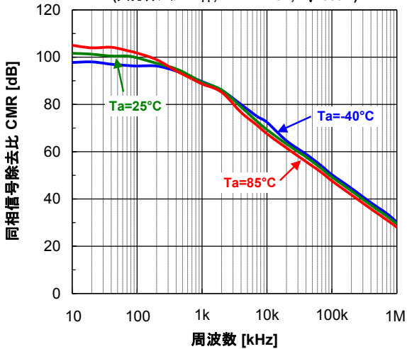
同相信号除去比 - 周波数 (入力リップル \Delta = 1V_{PP} , V^+/V^- = \pm 15V , A_V = 60dB )
