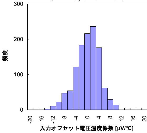
入力オフセット電圧温度係数分布 ( V^+/V^- = \pm 15V , T_a = -40^\circ C \rightarrow +25^\circ C )
