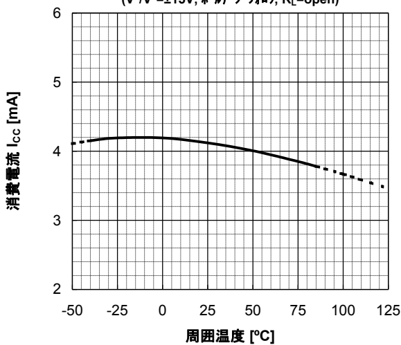
消費電流 – 周囲温度 ( V^+/V^- = \pm 15V , 負荷レジスタ開放, R_L = open )
