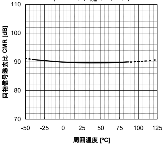
同相信号除去比 - 周囲温度 ( V^+/V^- = \pm 15V , V_{ICM} = 0V \rightarrow -10V )
