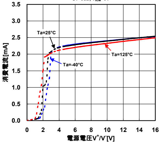
消費電流 対 電源電圧特性例 G_v=0dB, V_{ICM}=0V
