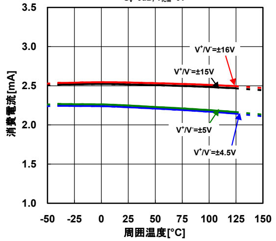
消費電流 対 周囲温度特性例 G_v=0dB, V_{ICM}=0V
