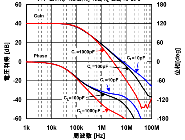
電圧利得・位相 対 周波数特性例 V^+ / V^- = \pm 5V, R_f=100k\Omega, R_G=1k\Omega, R_L=2k\Omega, T_a=25^\circ C
