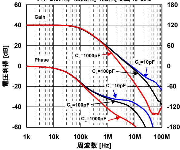
電圧利得・位相 対 周波数特性例 V^+ / V^- = \pm 15V, R_f=100k\Omega, R_G=1k\Omega, R_L=2k\Omega, T_a=25^\circ C
