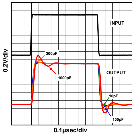
過渡応答特性例 (負荷容量) V^+ / V^- = \pm 15V, V_{IN}=1V_{pp}, R_L=2k\Omega, T_a=25^\circ C
