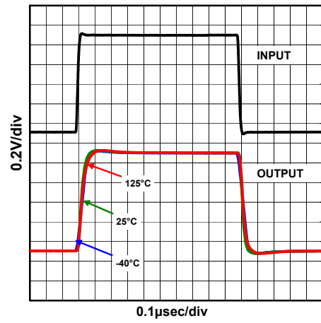
過渡応答特性例 (周囲温度) V^+ / V^- = \pm 15V, V_{IN}=1V_{pp}, R_L=2k\Omega, C_L=10pF
