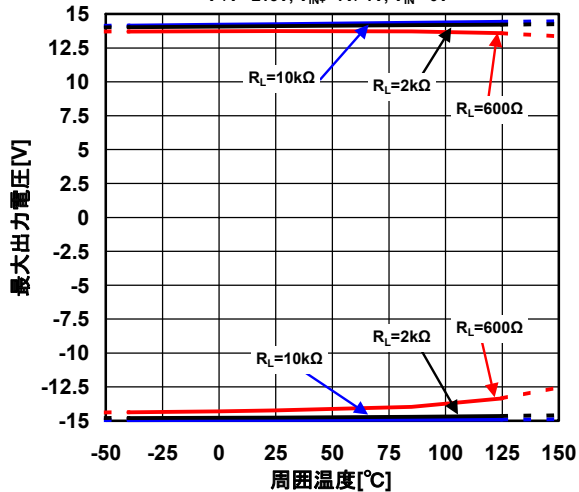
最大出力電圧 对 周囲温度特性例
