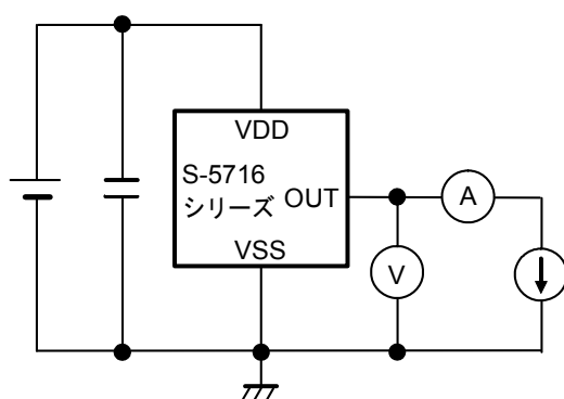
図8 測定回路3
