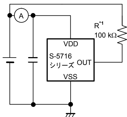
図6 測定回路1
