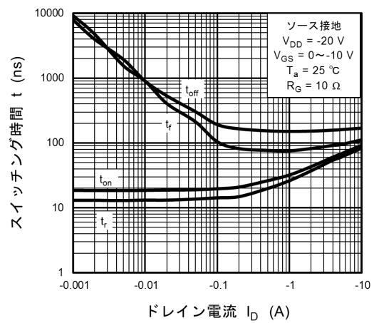
図 7.10 t - I D
