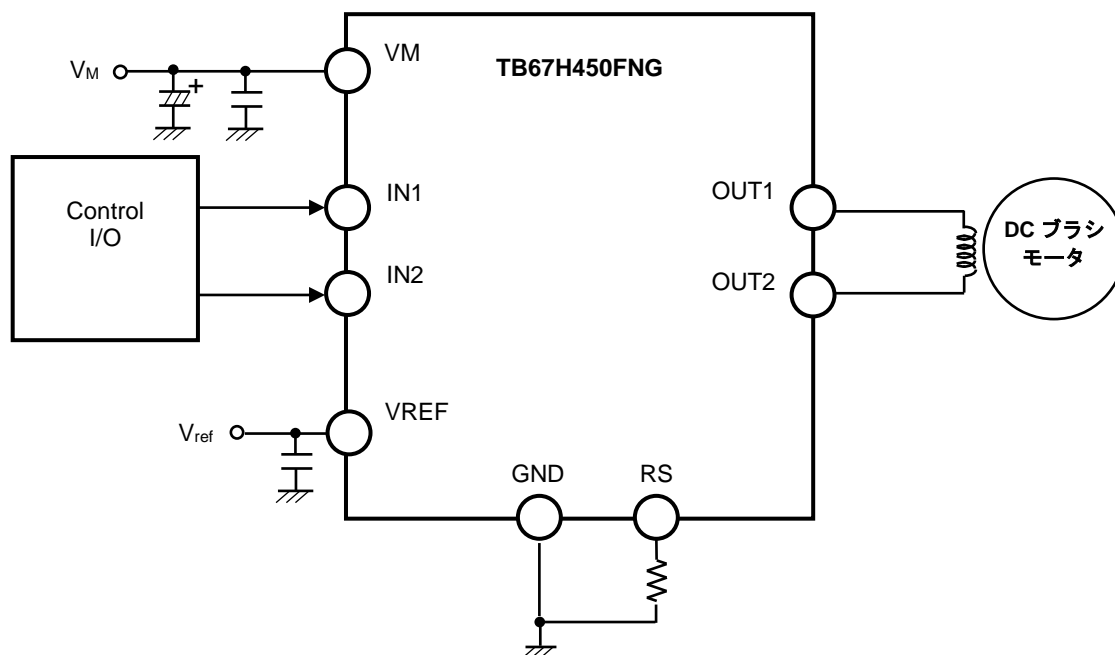
図 7-1 応用回路例(DC ブラシモータ)
