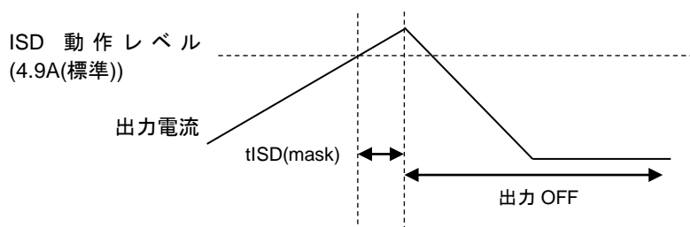
図 8-1 過電流検出動作
