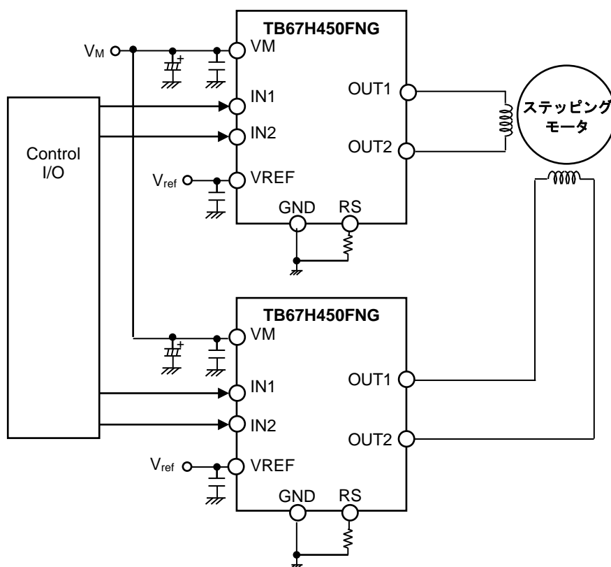
図 7-2 応用回路例(ステッピングモータ)
