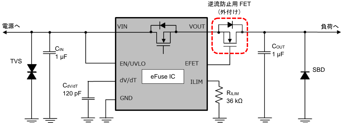
逆流防止機能を使用時の eFuse IC 周辺回路例
