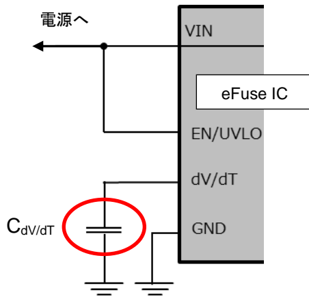
dV/dT 端子周辺外付け回路
