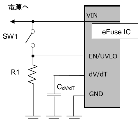
EN/UVLO 端子の接続例 (VIN とスイッチで接続)
