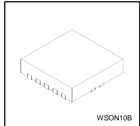
質量: 19.3 mg (標準)
