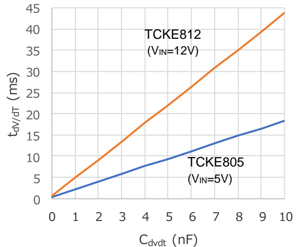
C_{dV/dT} - t_{dV/dT} 特性
