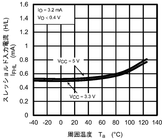
図 12.2.9 I_{FHL} - T_a
