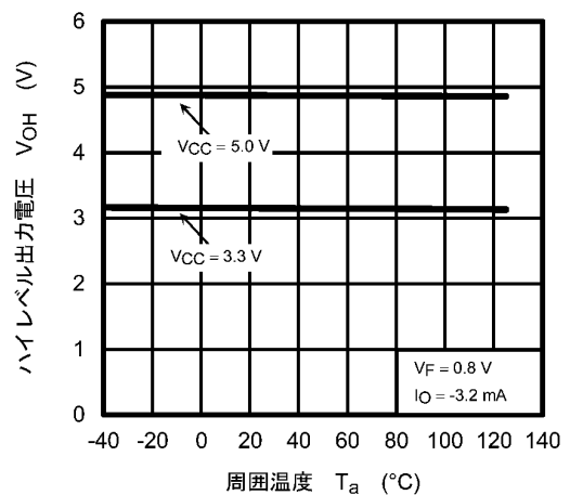
図 12.2.6 V_{OH} - T_a
