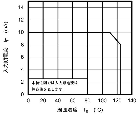
図 12.2.2 I_F - T_a
