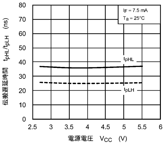
図 12.2.17 t_{pHL}/t_{pLH} - V_{CC}
