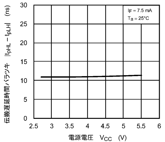
図 12.2.18 |t_{pHL} - t_{pLH}| - V_{CC}
