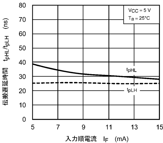
図 12.2.15 t_{pHL}/t_{pLH} - I_F
