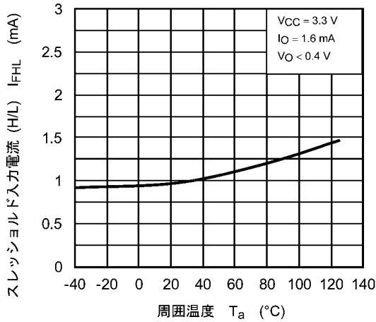
図 12.2.7 I FHL - T a
