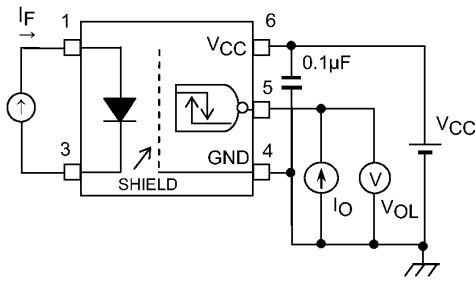
図 12.1.1 VOL測定回路
