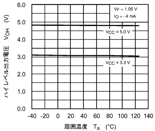
図 12.2.4 V_{OH} - T_a
