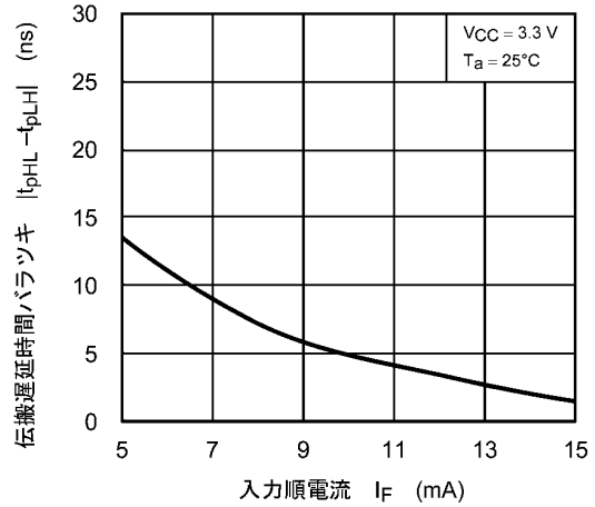
図 12.2.14 |t_{pHL} - t_{pLH}| - I_F
