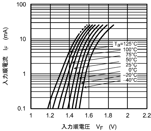
図 12.2.1 I_F - V_F
