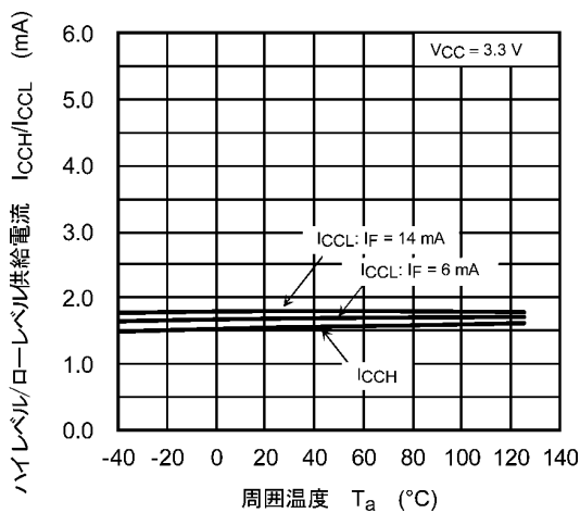
図 12.2.5 I_{CCH}/I_{CCL} - T_a
