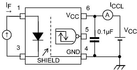
図 12.1.3 ICCL測定回路
