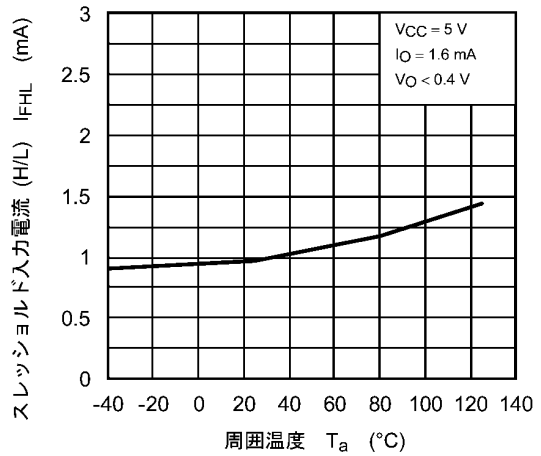
図 12.2.8 I FHL - T a
