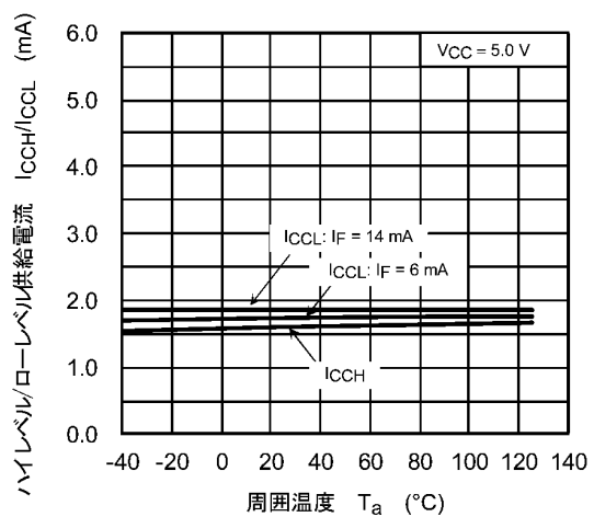
図 12.2.6 I_{CCH}/I_{CCL} - T_a
