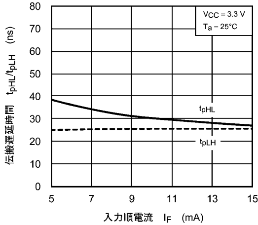
図 12.2.13 t_{pHL}/t_{pLH} - I_F
