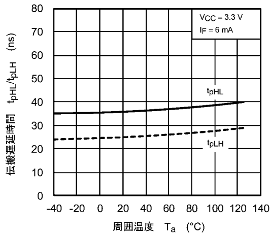
図 12.2.9 t pHL /t pLH - T a
