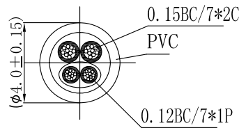
线材剖面图
