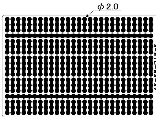
AE-SB-DIP-F L1-PATTERN
