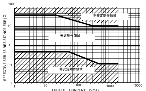
Fig.34 ESR vs Io 特性 (BAxxDD0, 22µF)
