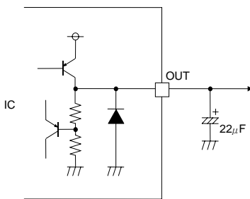
Fig.32 出力等価回路
