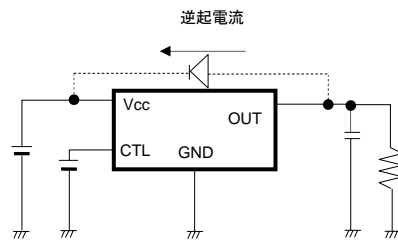
Fig.35: バイパスダイオード
