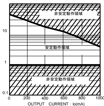
Fig.33 ESR - Io 特性 (BAxxCC0, 22µF)
