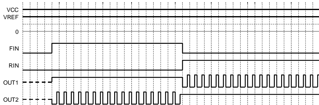
Fig.38 VREF 制御モード(タイミングチャート)
