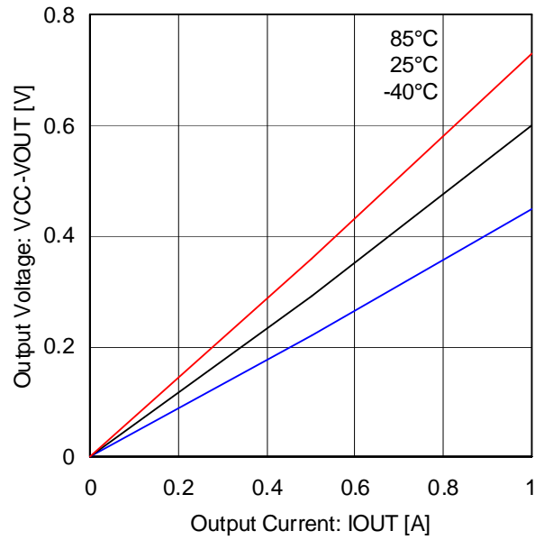
Fig.22 出力 H 電圧(BD6221/26)
