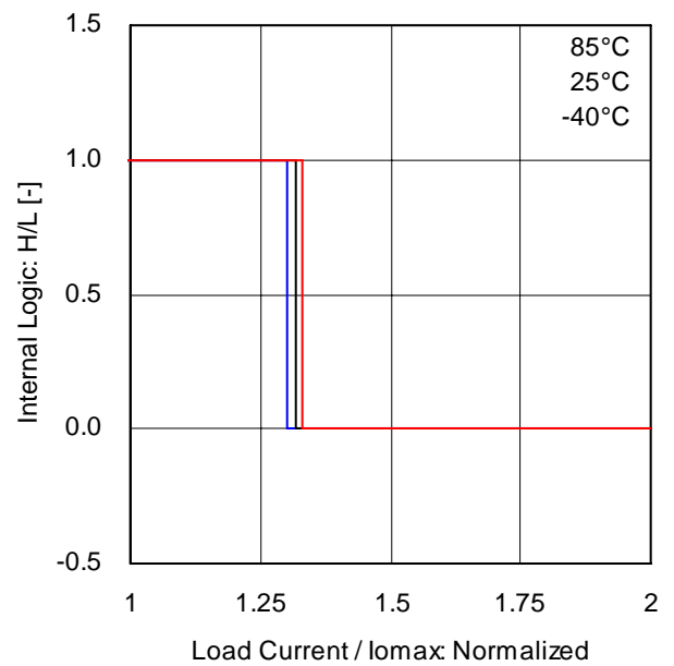
Fig.20 過電流保護回路特性(下)
