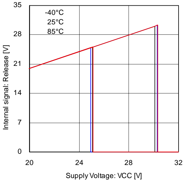
Fig.17 過電圧保護回路特性
