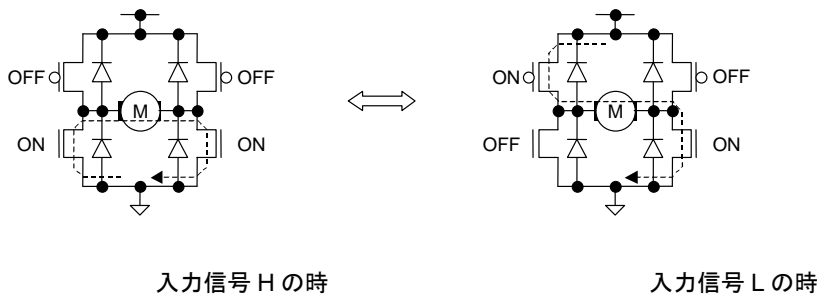
Fig.36 PWM 制御モード(出力)
