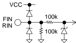
Fig.40 FIN / RIN
