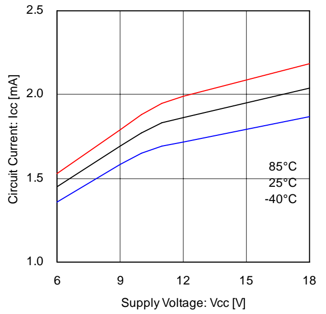
Fig.10 回路電流(2ch)
