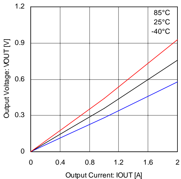
Fig.29 出力 L 電圧(BD62222)
