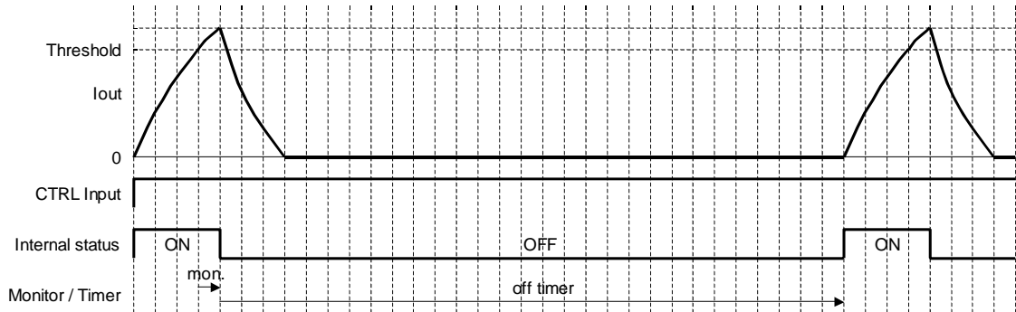
Fig.39 過電流保護動作の例(タイミングチャート)
