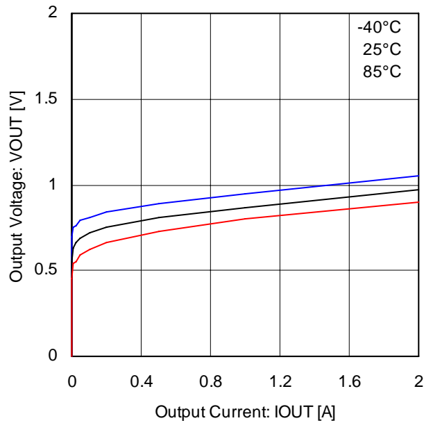
Fig.32 下側 Di 特性(BD6222)
