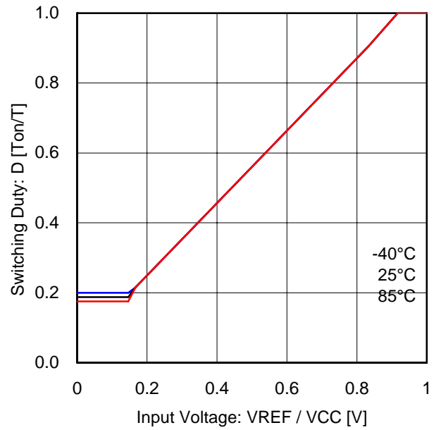
Fig.14 VREF - DUTY 特性(VCC=12V)
