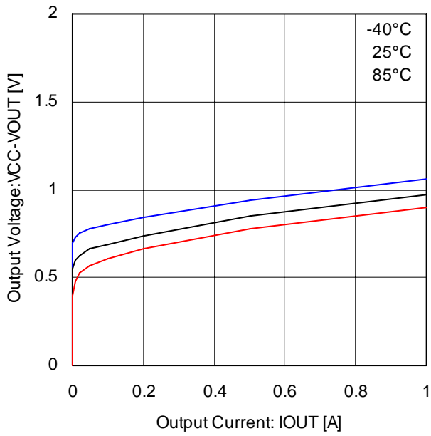
Fig.25 上側 Di 特性(BD6221/26)
