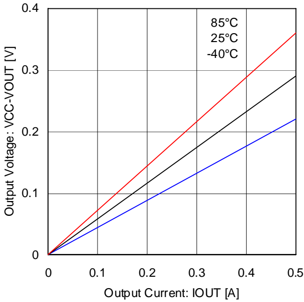
Fig.21 出力 H 電圧(BD6220/25)
