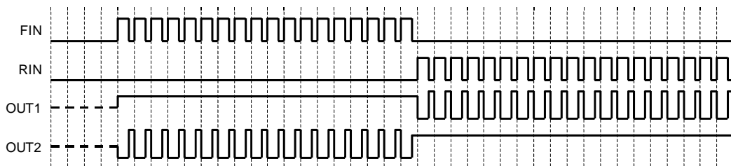
Fig.35 PWM 制御モード(タイミングチャート)
