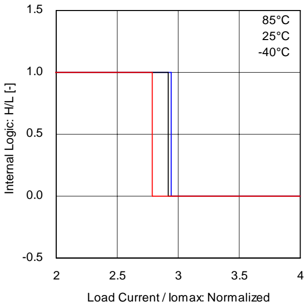
Fig.19 過電流保護回路特性(上)
