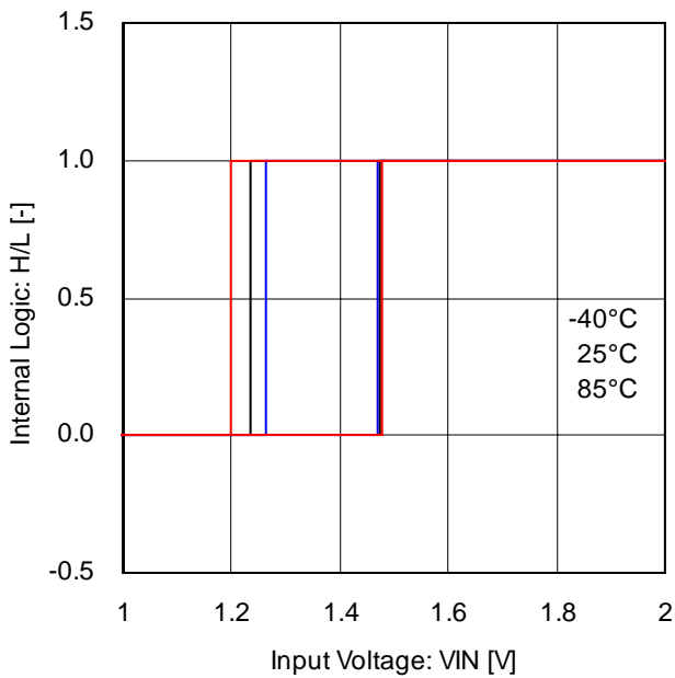
Fig.11 入カスレッシュヨルド電圧
