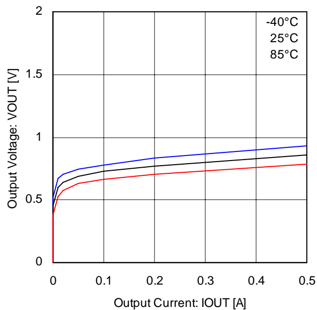
Fig.30 下側 Di 特性(BD6220/25)
