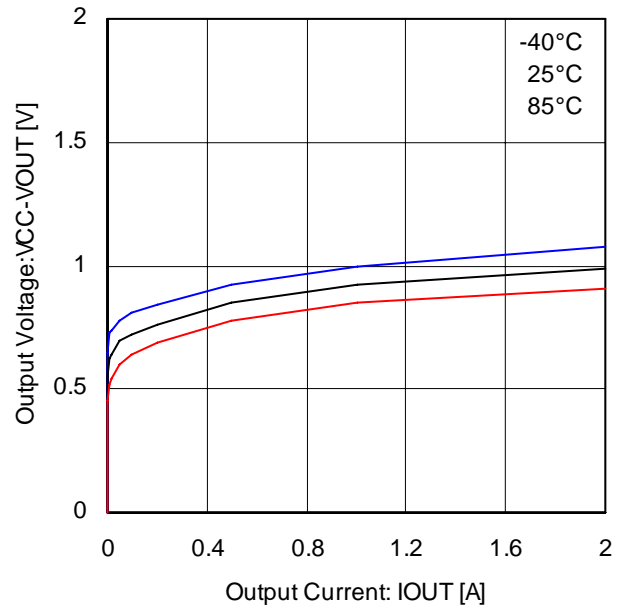
Fig.26 上側 Di 特性(BD6222)
