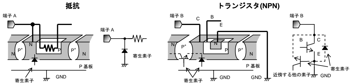
Fig.44 ICの簡易構造例
