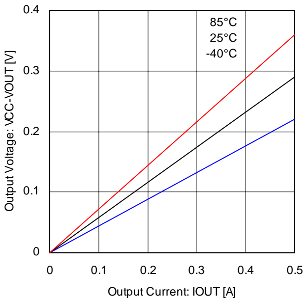
Fig.23 出力 H 電圧(BD6222)
