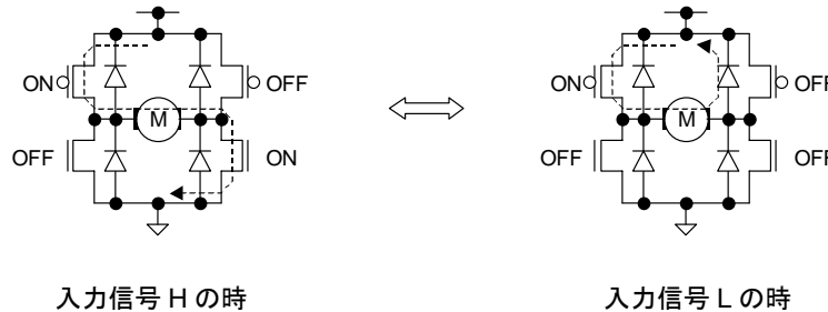
Fig.34 PWM 制御モード(出力)
