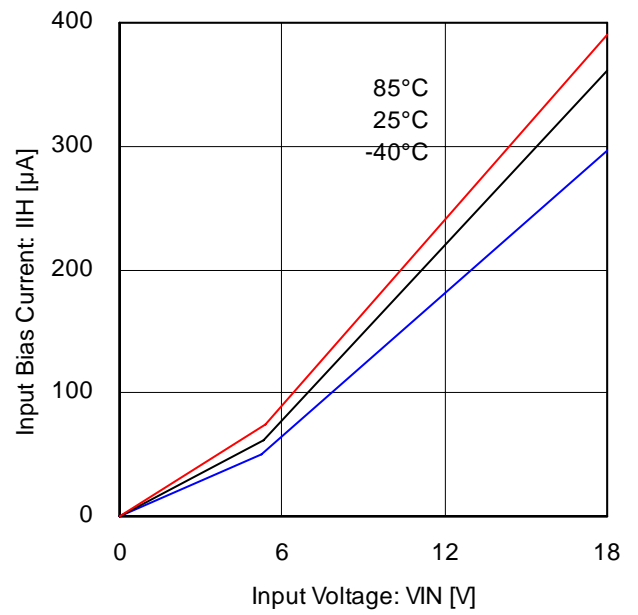
Fig.12 入カバイアス電流
