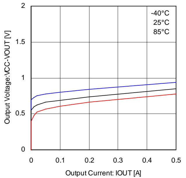
Fig.24 上側 Di 特性(BD6220/25)
