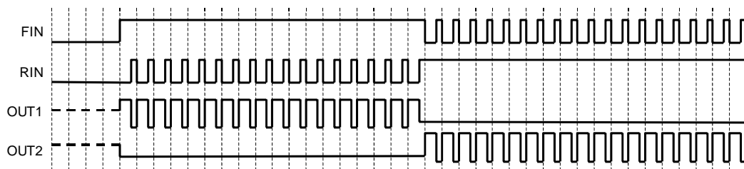
Fig.36 PWM 制御モード(出力)
