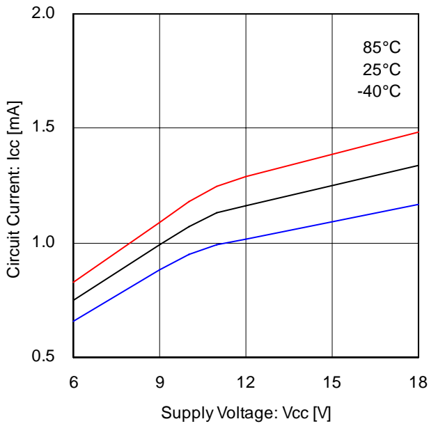
Fig.9 回路電流(1ch)
