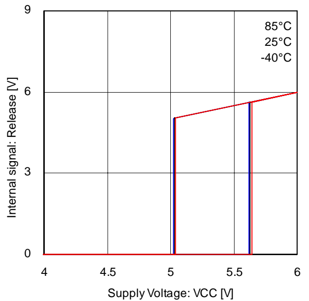
Fig.16 不足電圧保護回路特性
