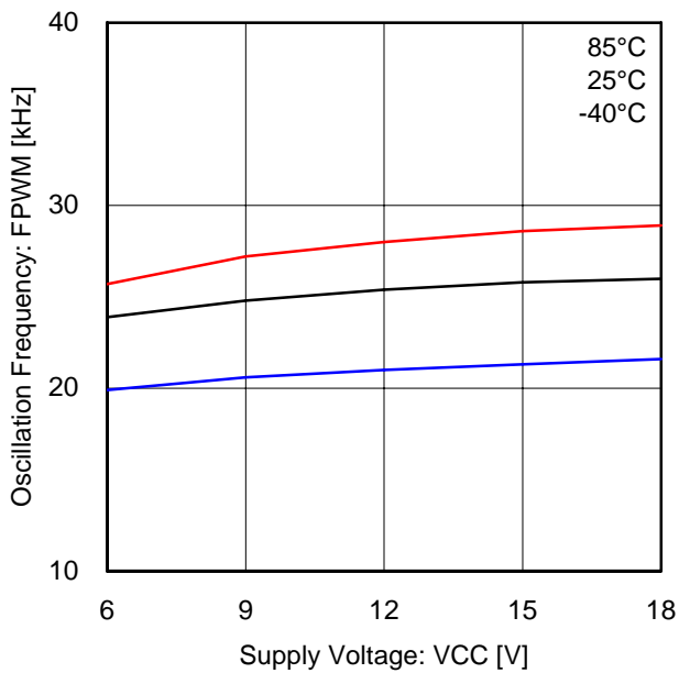
Fig.15 VCC-キャリア周波数特性
