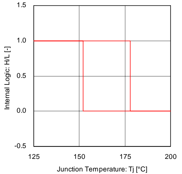
Fig.18 過熱保護回路特性
