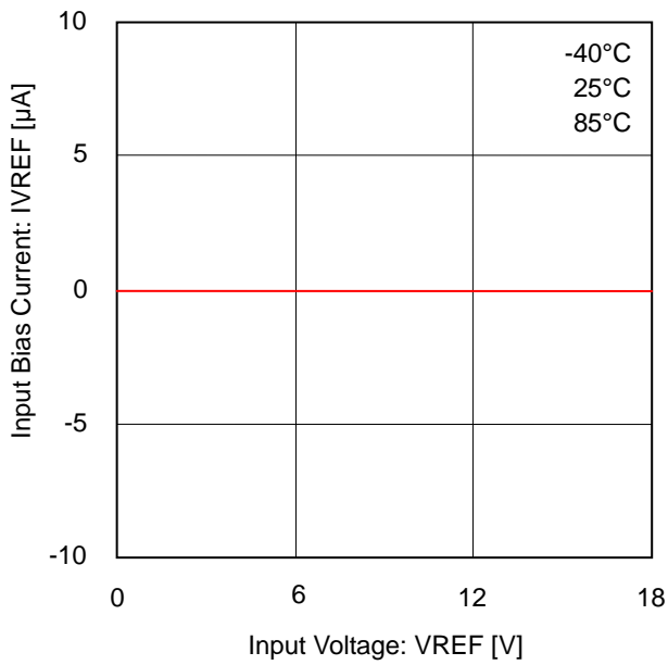
Fig.13 VREF 入力バイアス電流
