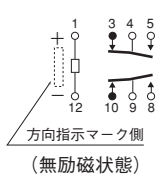
端子配列・内部結線図 (BOTTOM VIEW) シングルスティブル型
