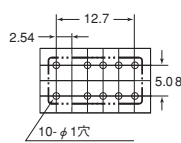
プリント板加工図 (BOTTOM VIEW)
