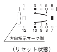
端子配列・内部結線図 (BOTTOM VIEW) 2巻線ラッチング型
