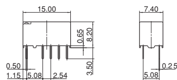
2巻線ラッチング型 外形寸法図 標準プリント板用端子
