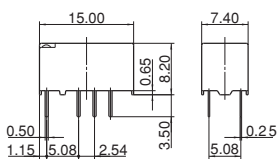
シングルスティブル型 外形寸法図 標準プリント板用端子
