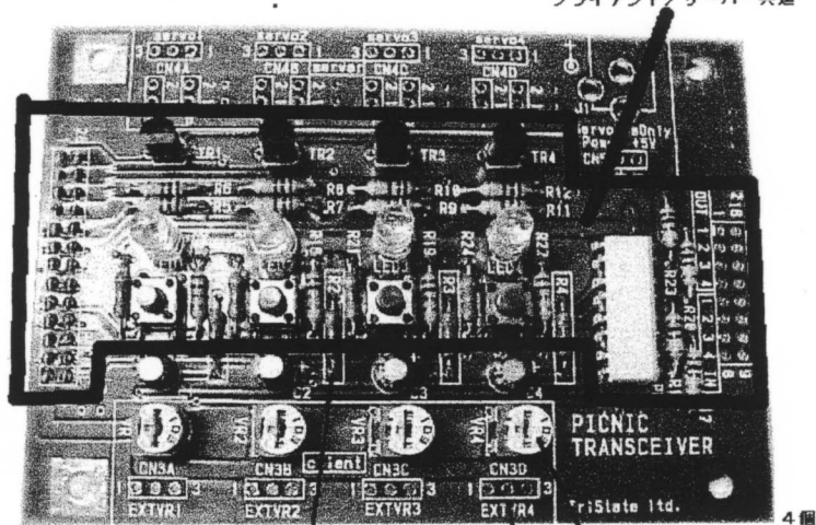
サーバー用基板上ボリューム 又は外部ボリューム用端子 4個
