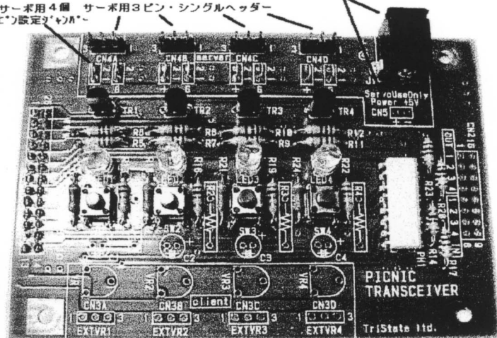
サーバー専用DC5Vコネクタ
