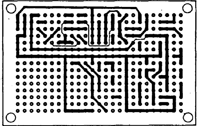
パターン図
