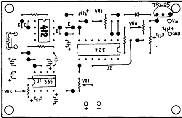
部品配置図
